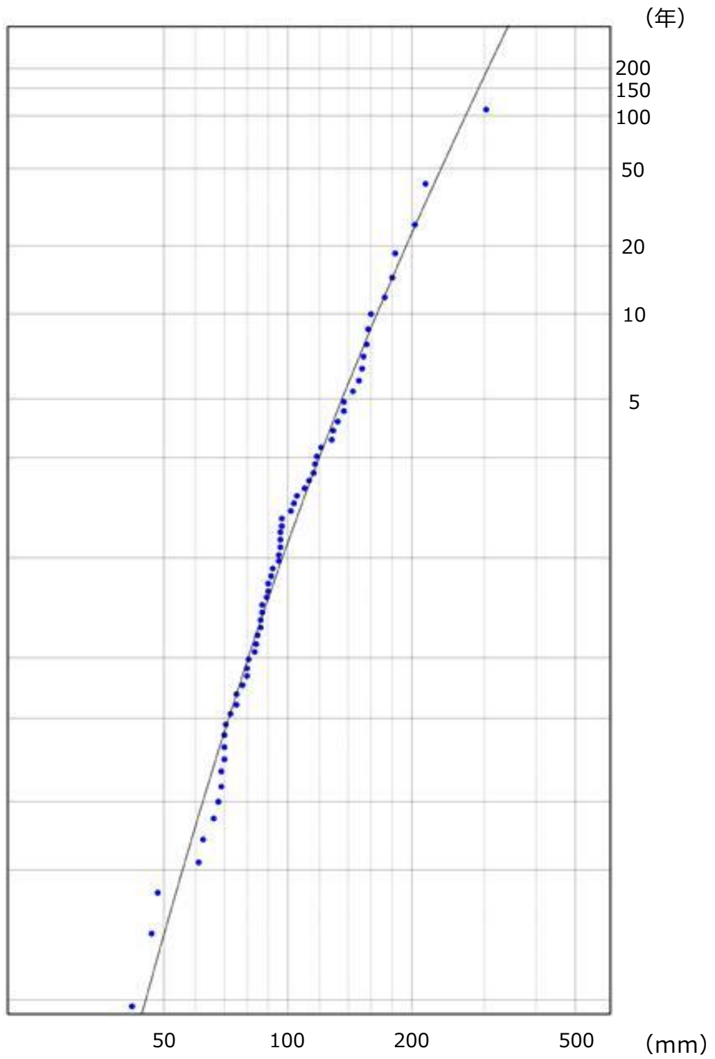
第2図 100年超過確率24時間雨量（観測地点「恵曇，鹿島」） 確率統計解析結果
