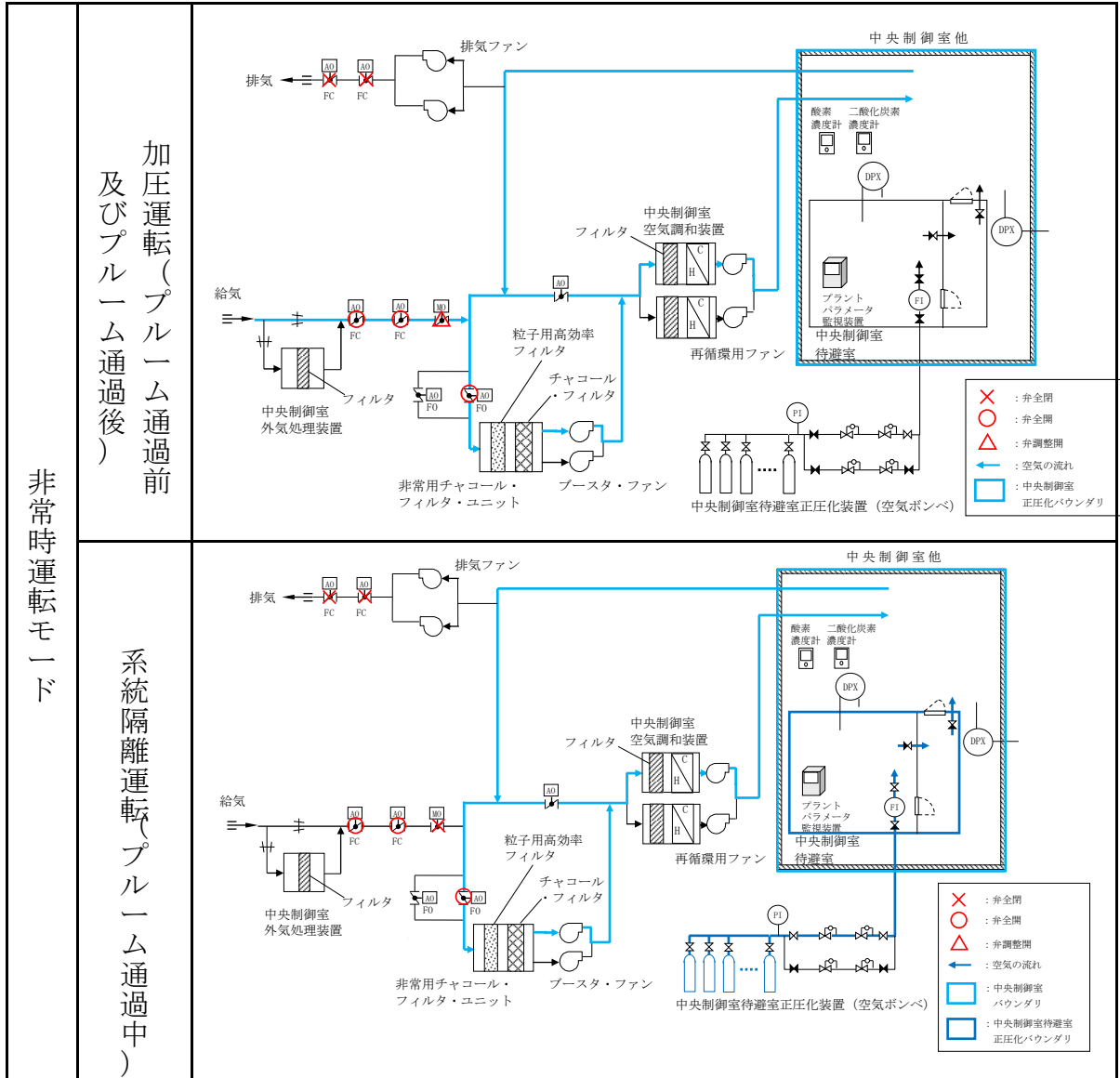
図 2.4-19 運転モード毎の中央制御室換気系 系統概要図 (2/2)
