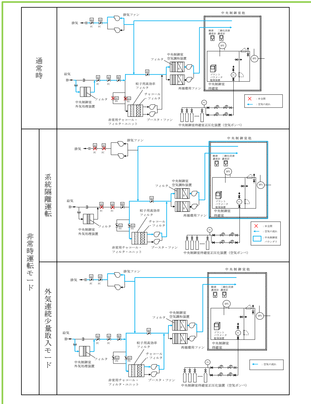
図 2.4-19 運転モード毎の中央制御室換気系 系統概要図（1／2）
