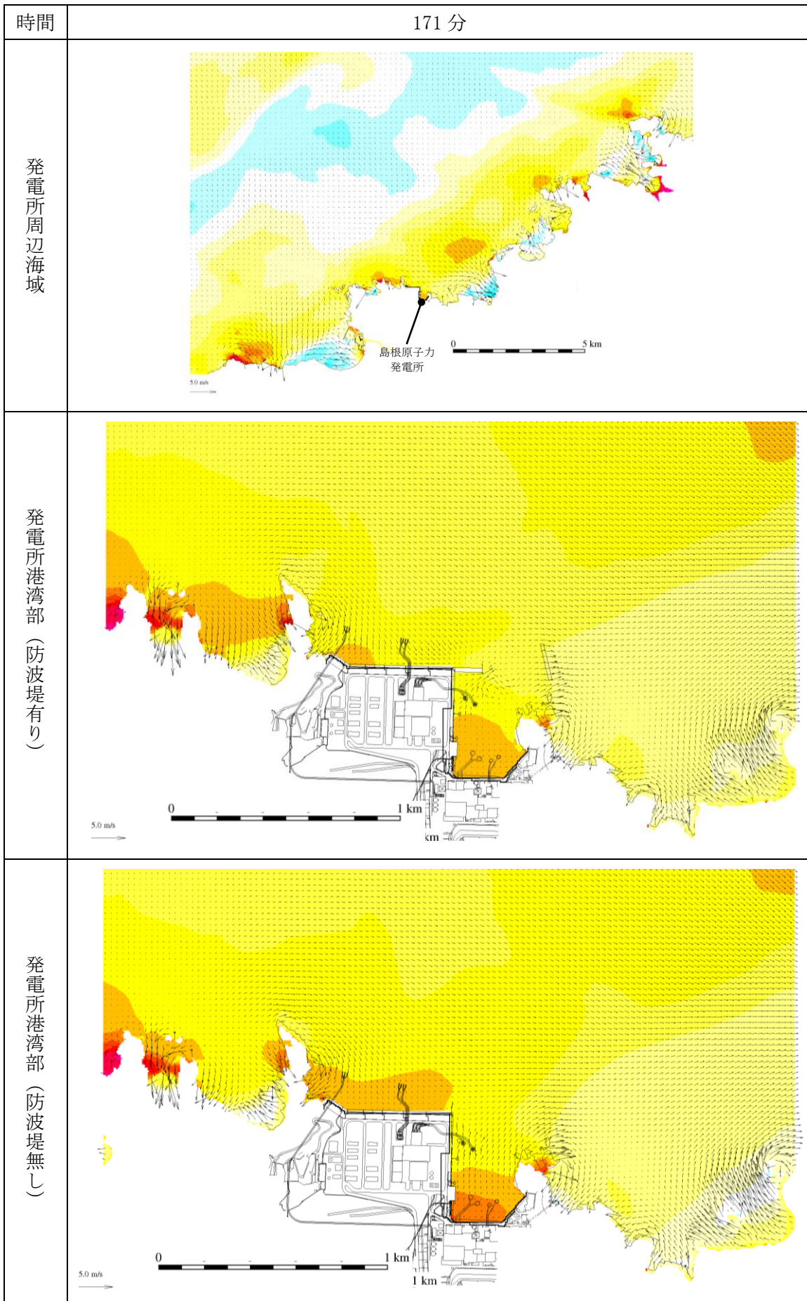
第 1 図(143) 基準津波 1 の水位変動・流向ベクトル
