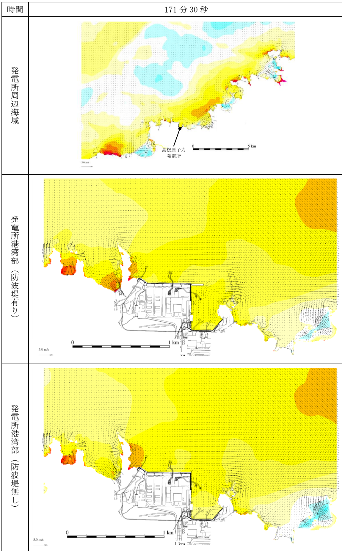
第 1 図(144) 基準津波 1 の水位変動・流向ベクトル
