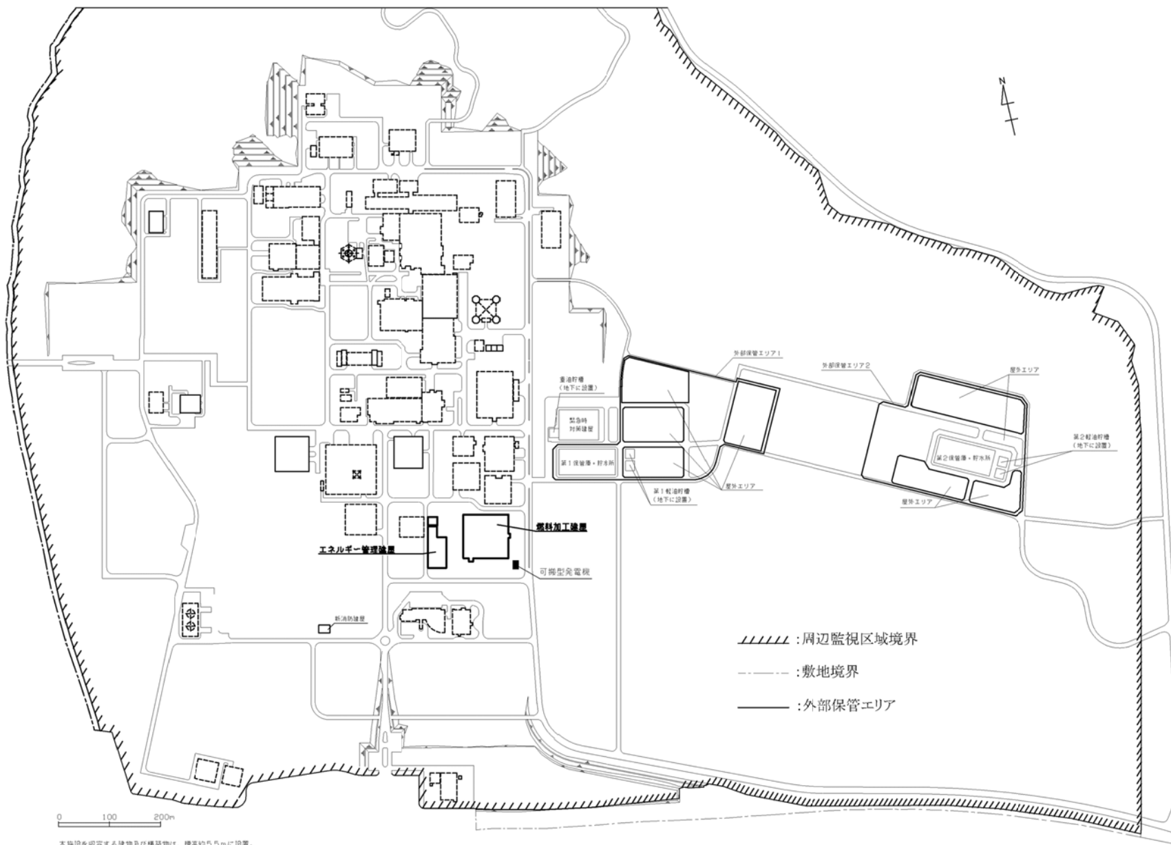
第1図 再処理事業所内の可搬型重大事故等対処設備の保管場
