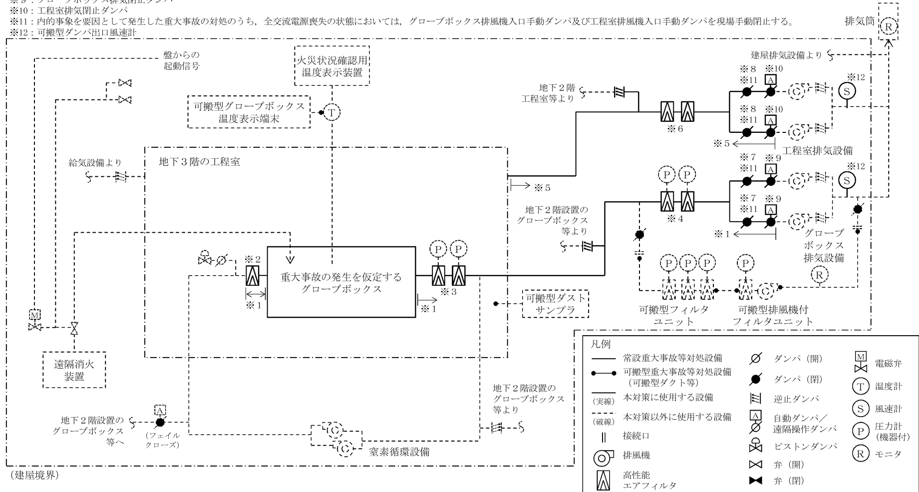
第6-4図 放出防止設備の系統概要図（内の事象の対処時）（その1） 外部放出抑制設備の設計基準対象の施設と兼用一覧
