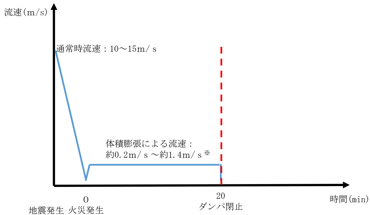
第6-23 図 工程室排気ダクト内の流速推移
