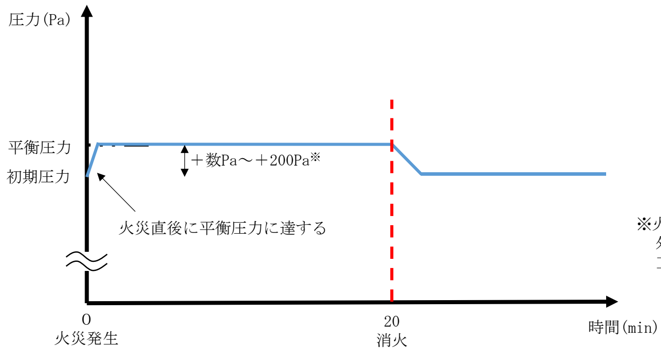
第6-21図 工程室内圧力推移
