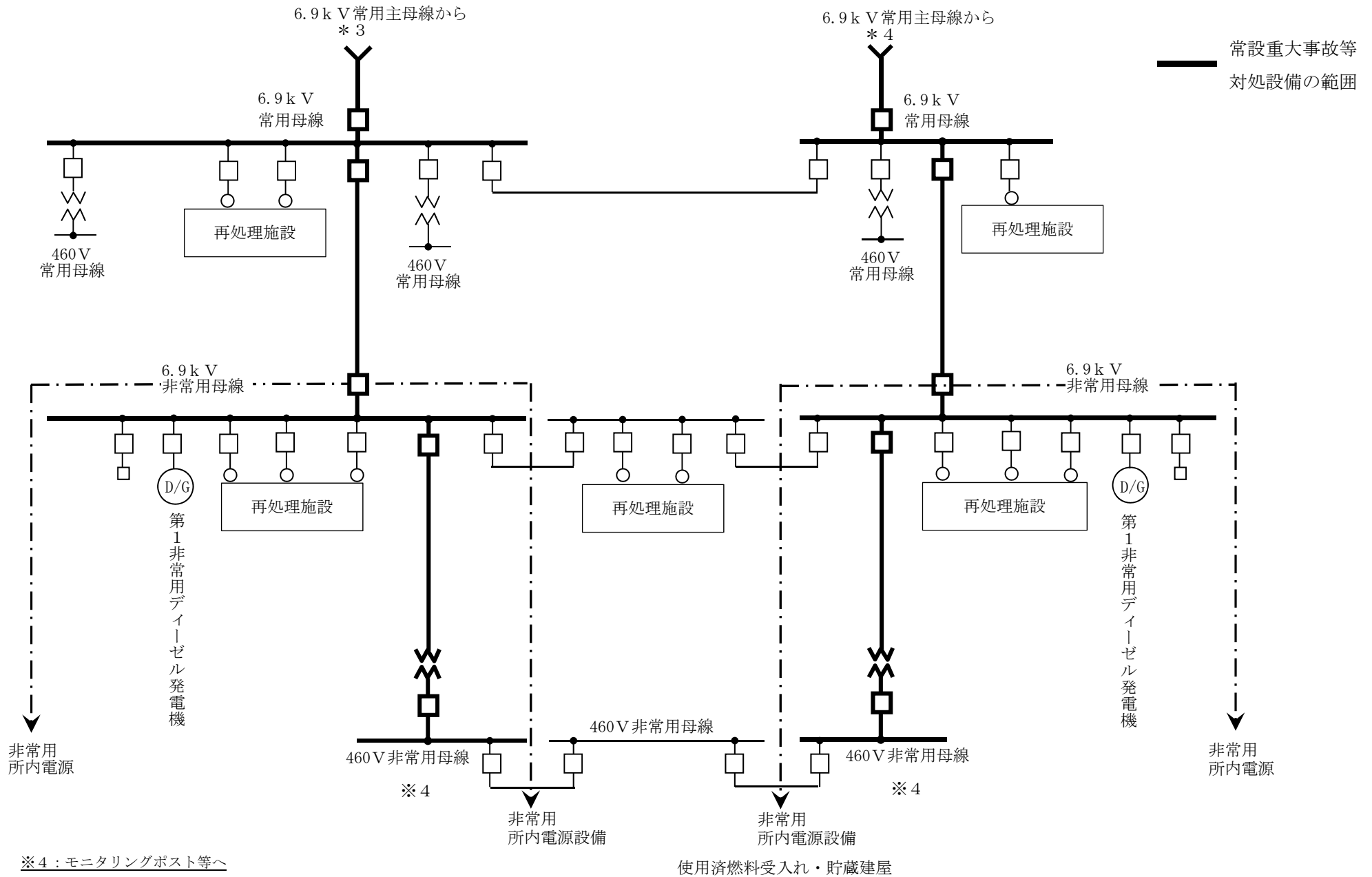
第 32. 6 図 全交流電源喪失以外の状態において重大事故等に対処するための設備の系統図(3 / 5)
