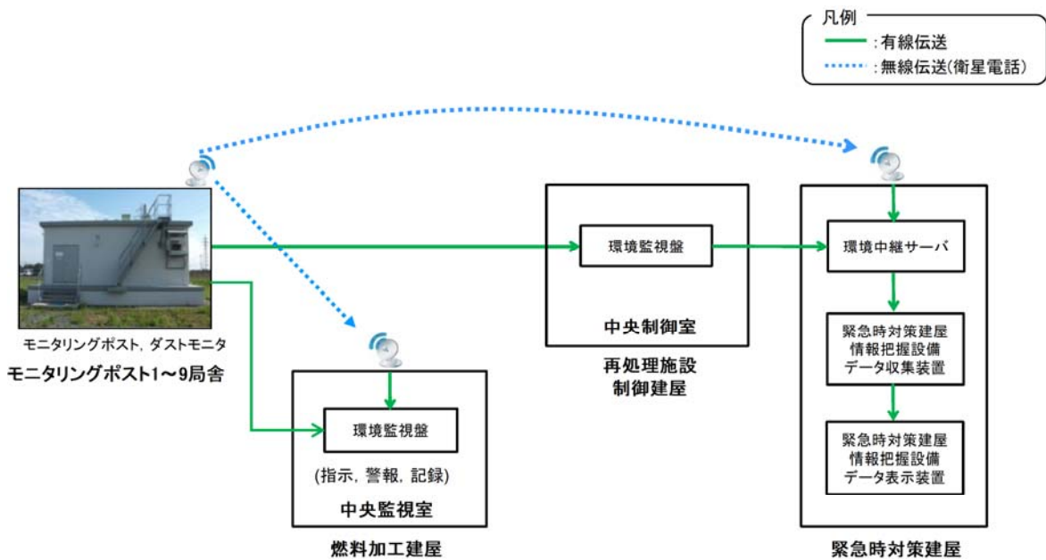
第4図 モニタリングポスト等の系統概略図
