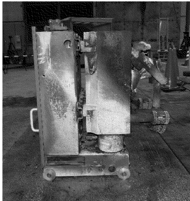
遮断器室アーク発生、アーク火災有、消火後の遮断器の様子
