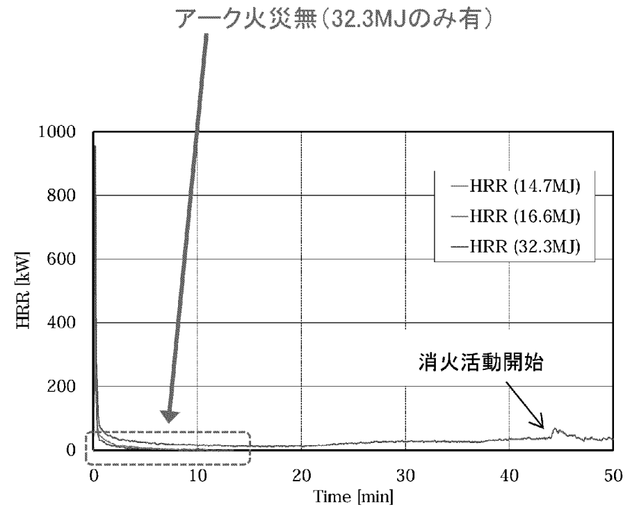
発熱速度(HRR)測定結果(M/C(D/G)試験時)
