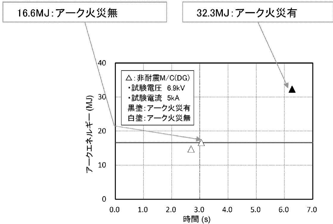
試験結果 (アーク火災発生状況)
