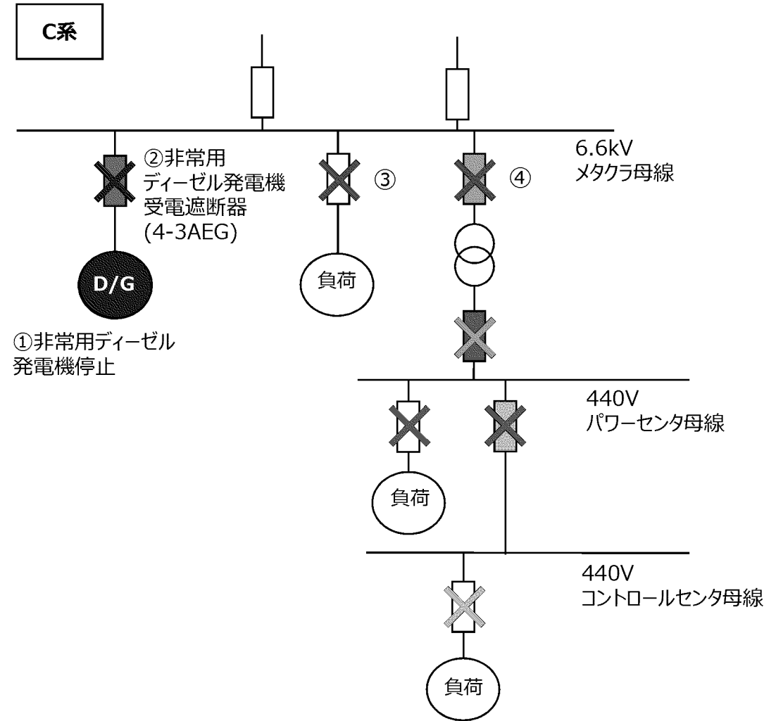
玄海3号機 所内電気系統 (概要図)
