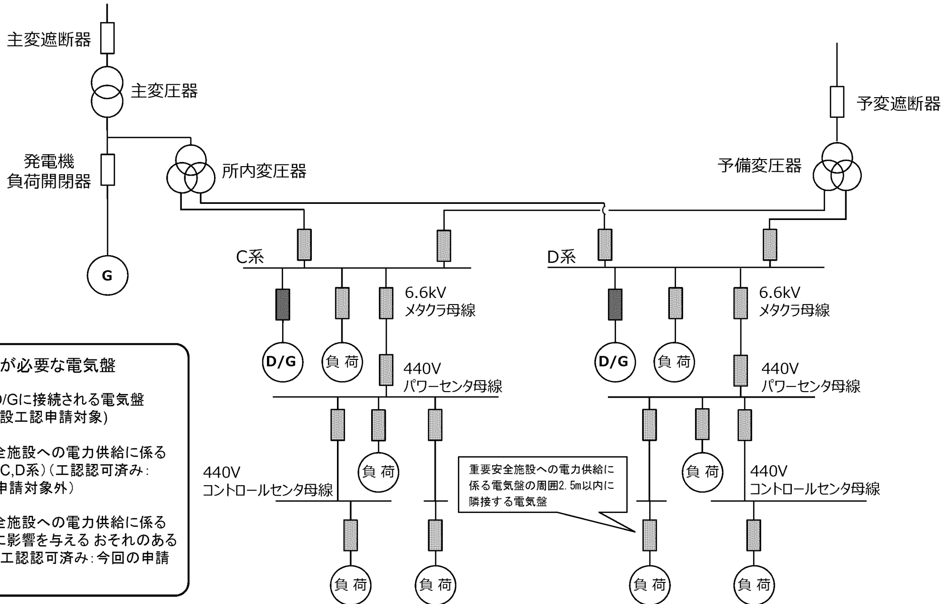
玄海3号機 所内電気系統(概要図)
