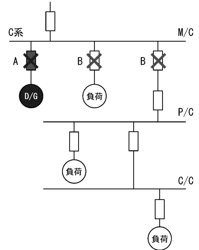
玄海3号機 所内電気系統（概略図）
