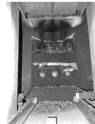
盤内開口部の状態(遮断器室)
