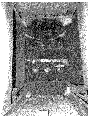
盤内開口部の状態(遮断器室)
