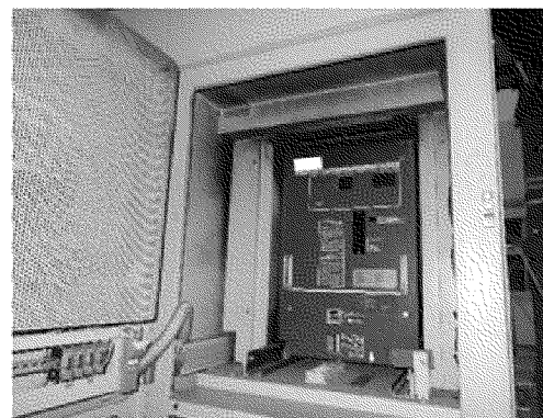
試験後の盤正面の状態
