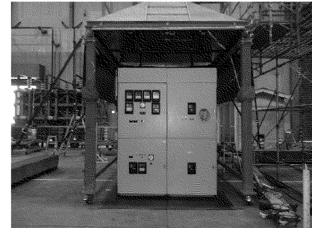
試験状況(M/C(D/G)試験時)
