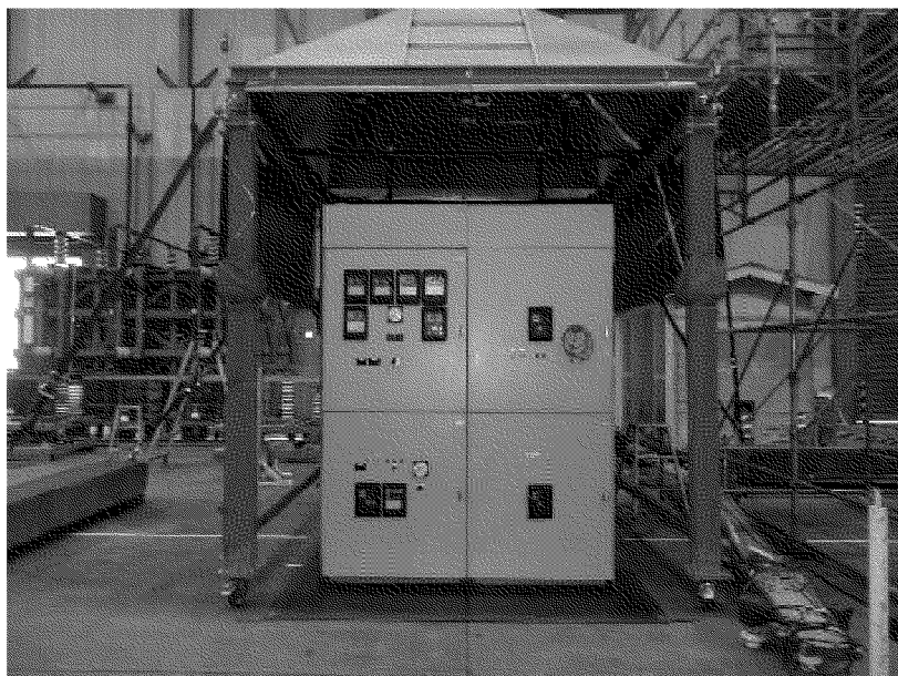
試験状況(M/C(D/G)試験時)
