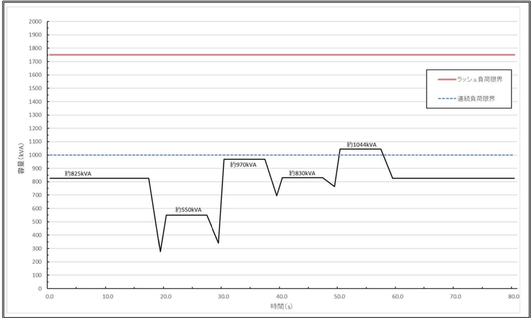
第5. 2. 7-2. 2-5図 負荷容量曲線
