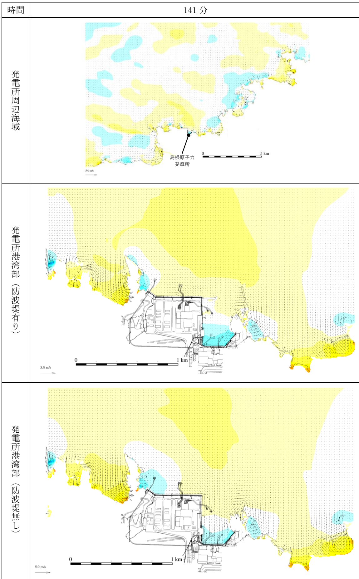
第 1 図(83) 基準津波 1 の水位変動・流向ベクトル
