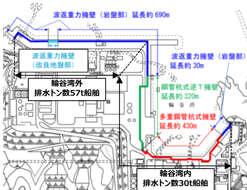
第 10-5-5 図 対象漂流物の設定
