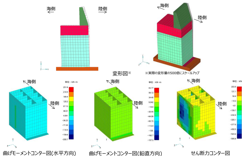
第 10-5-6 図 3次元静的 FEM 解析結果
