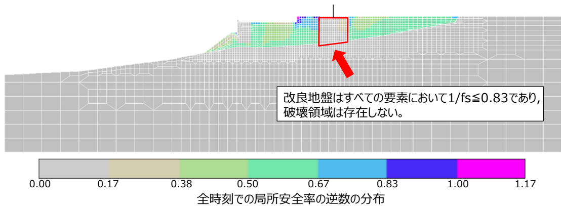
第 10-4-8 図 全時刻での局所安全率の逆数の分布
