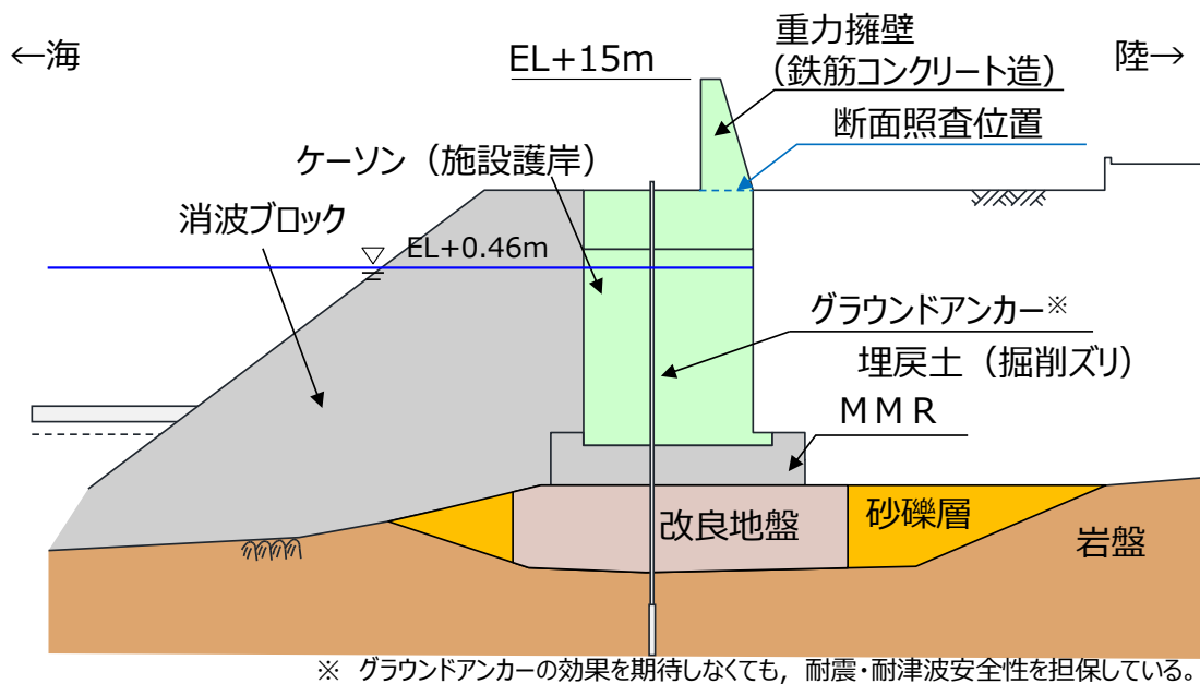
第 10-5-4 図 地下水位概要図（津波時）
