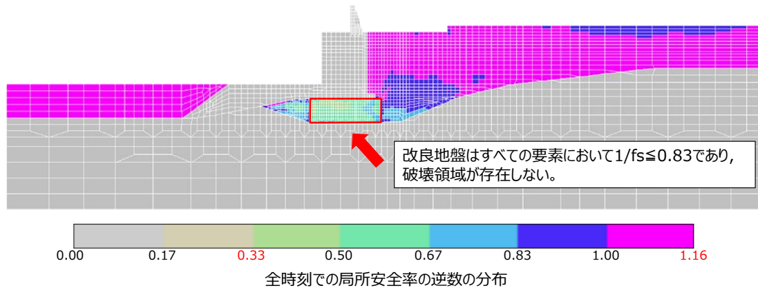
第 10-5-7 図 全時刻での局所安全率の逆数の分布
