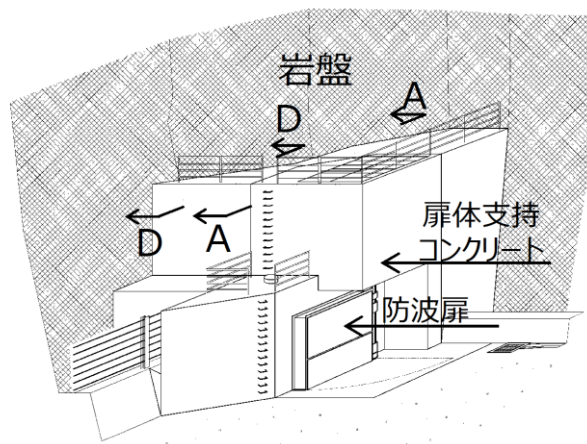
第8-24図 1号放水連絡通路防波扉の鳥瞰図（2）
