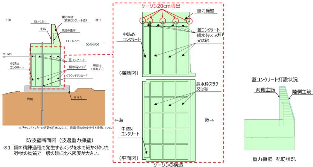
第7-46 図 防波壁（波返重力擁壁） ケーソンの構造
