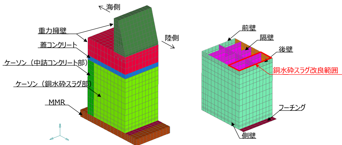
第10-5-3 図 3次元静的FEM解析の解析モデル図 (改良地盤部)
