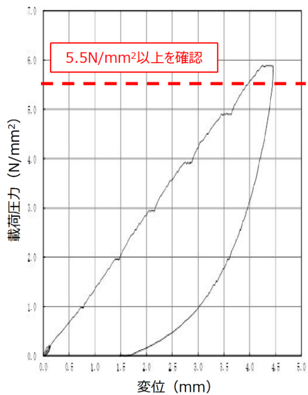
第 6-33 図 防波壁 (鋼管杭式逆 T 擁壁) 平板載荷試験結果
