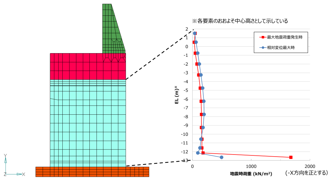
3次元モデルにおける地震時荷重入力位置
