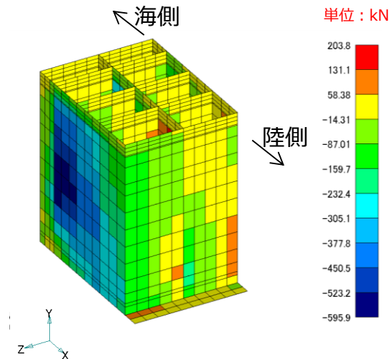
第 7-35 図 ケーソンの変形図及び断面力図(モーメント図及びせん断力図)
