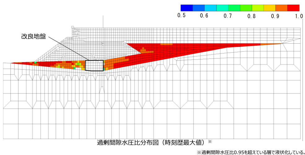
第 10-3-10 図 改良地盤①（砂礫層）前面有りの全時刻での過剰間隙水圧比の分布
