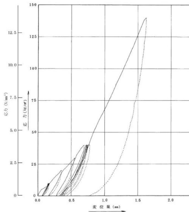
第 6-31 図 防波壁（鋼管杭式逆 T 擁壁）平板載荷試験結果
