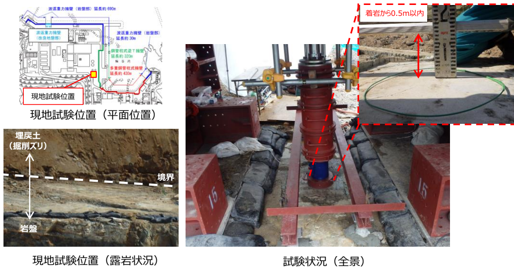
第 6-32 図 防波壁 (鋼管杭式逆 T 擁壁) 平板載荷試験概要
