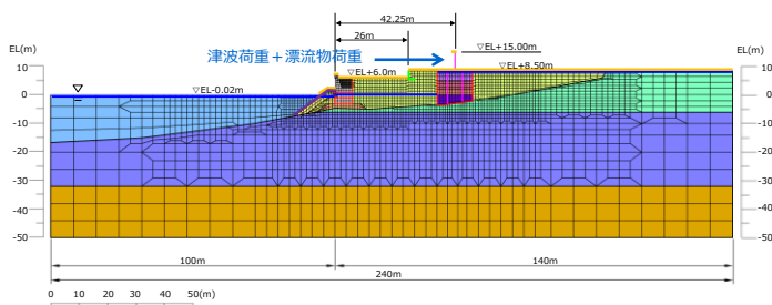
第 6-21 図 解析の概要
