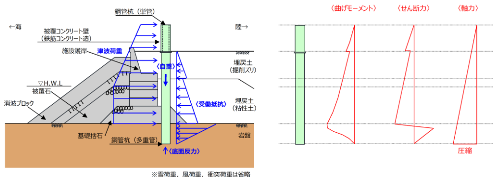
荷重図
