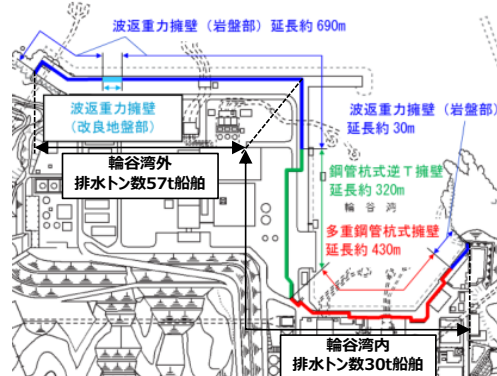
第10-3-5図 対象漂流物の設定
