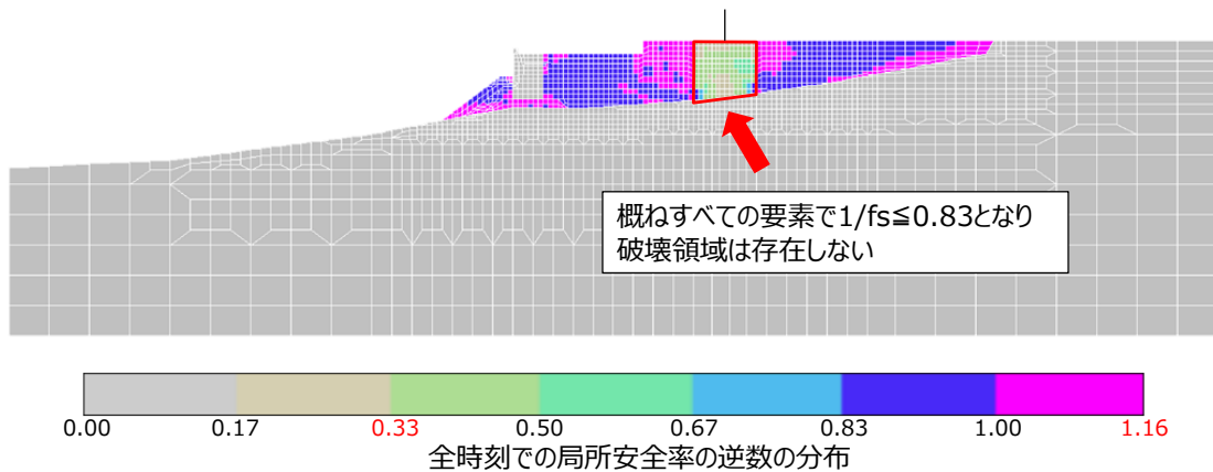
第 10-4-7 図 全時刻での局所安全率の逆数の分布
