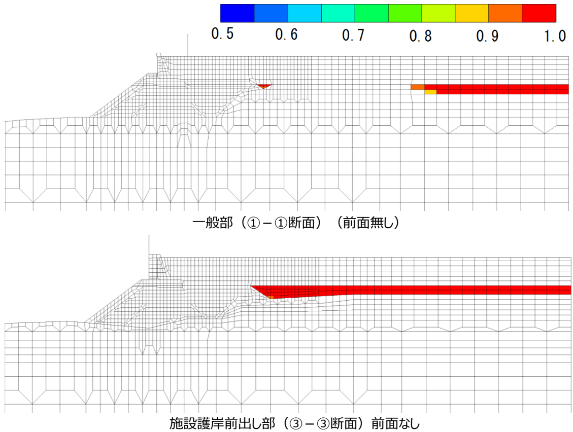
第 10-3-12 図 【参考】全時刻での過剰間隙水圧比の分布
