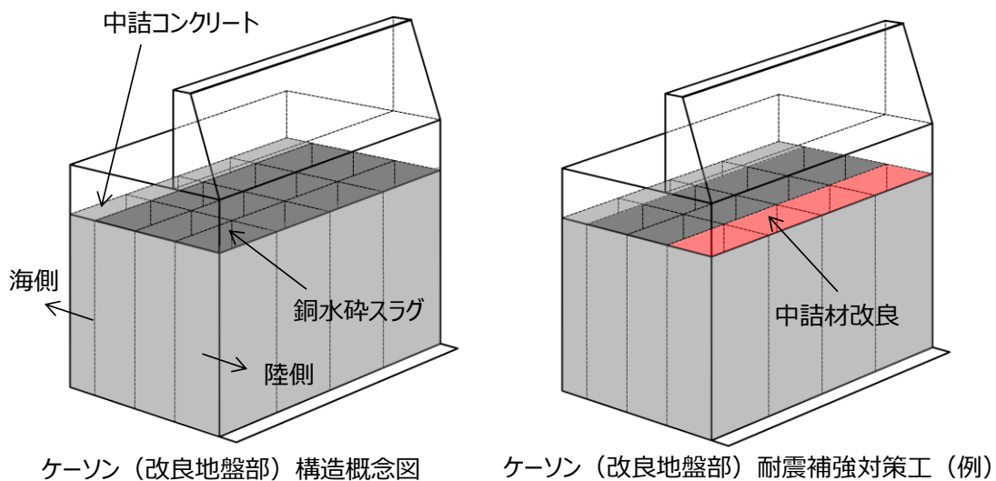
第7-35 図 ケーソン(改良地盤部)構造概念及び耐震補強対策工(例)
