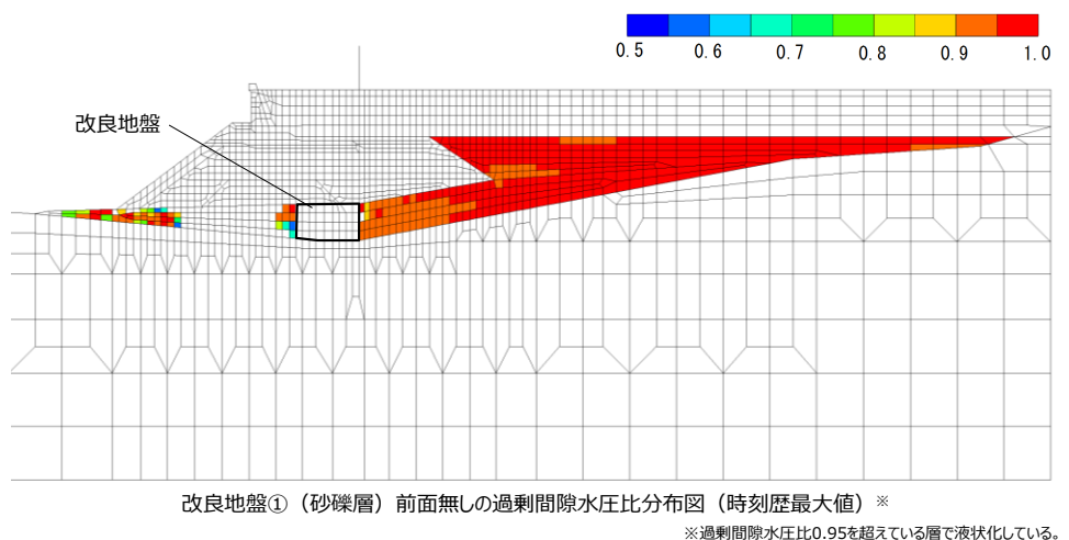
第 10-3-11 図 改良地盤①（砂礫層）前面無しの全時刻での過剰間隙水圧比の分布
