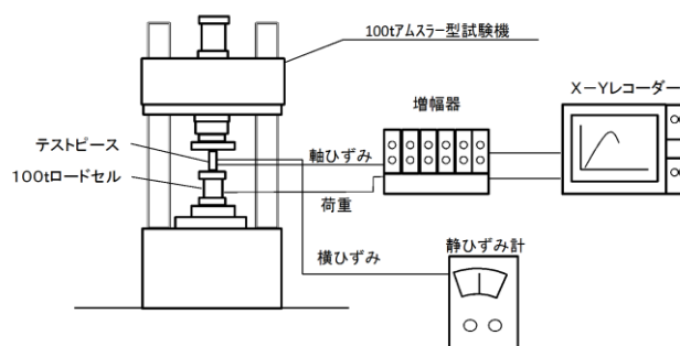
第9-18図 一軸圧縮試験概要
