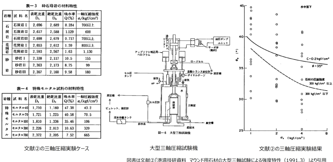
第 9-9 図 文献②の三軸圧縮実験ケース及び実験結果
