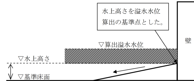
図 2-1 溢水水位算出時の床勾配の考え方
