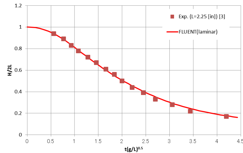
第 6 図 水柱高さ H の時間変化
