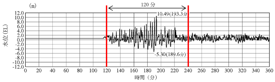
2号炉取水槽（入力津波1，防波堤無し）
