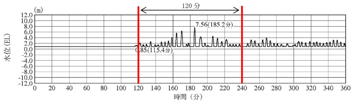
2号炉放水槽（入力津波 1，防波堤無し）
