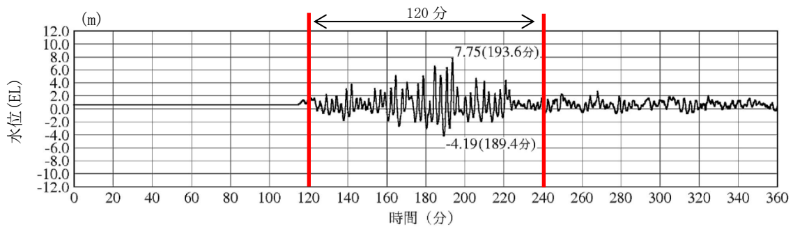
3号炉取水槽（入力津波1，防波堤無し）
