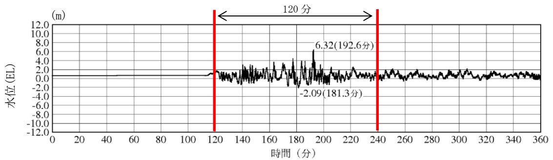
2号炉放水接合槽（入力津波 1，防波堤有り）
