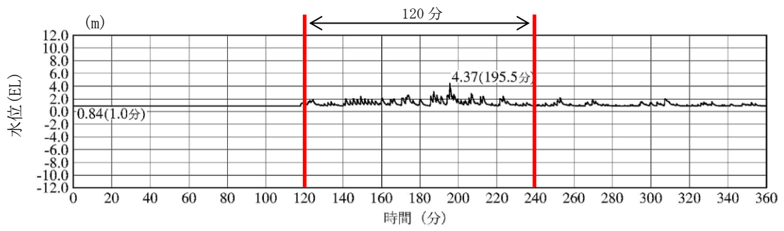
1号炉放水槽 (入力津波 1, 防波堤有り)
