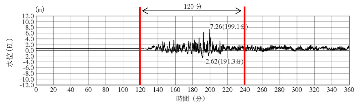
3号炉放水槽（入力津波 5，防波堤無し）
