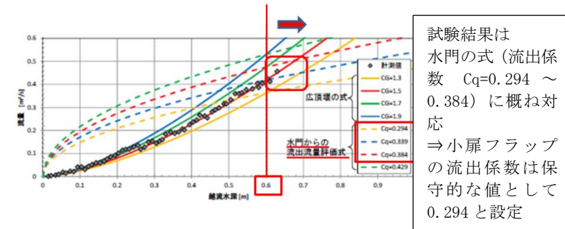
図 3-7 流出係数の設定 (水門の式)
