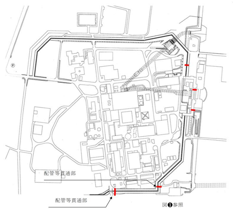
第2.2-43図 防潮堤貫通部配置図
