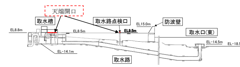
第 2.2-19 図 3号炉 取水施設の断面図
