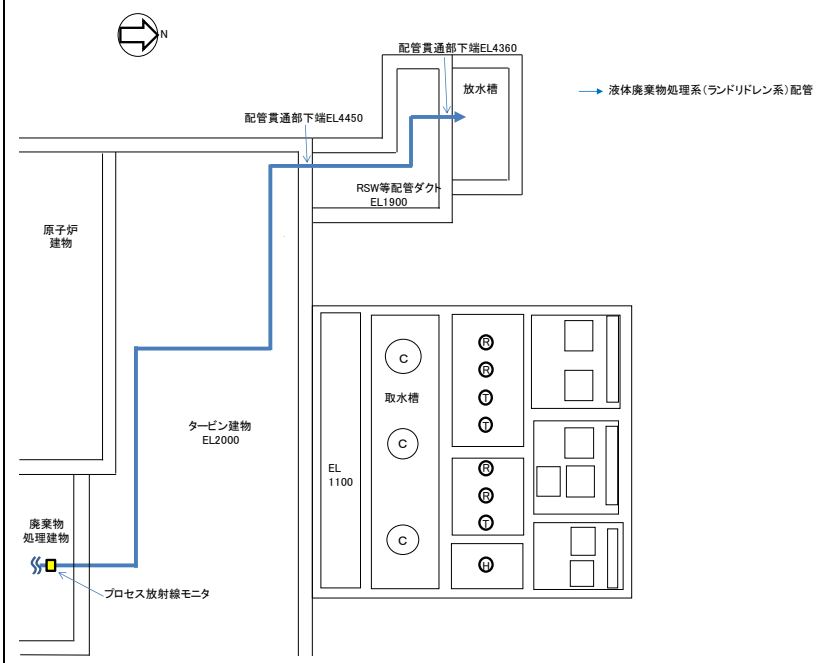
第2.2-16図 その他排水管の経路概要図
