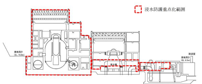
第2.4-2-2図 浸水防護重点化範囲(断面図)
