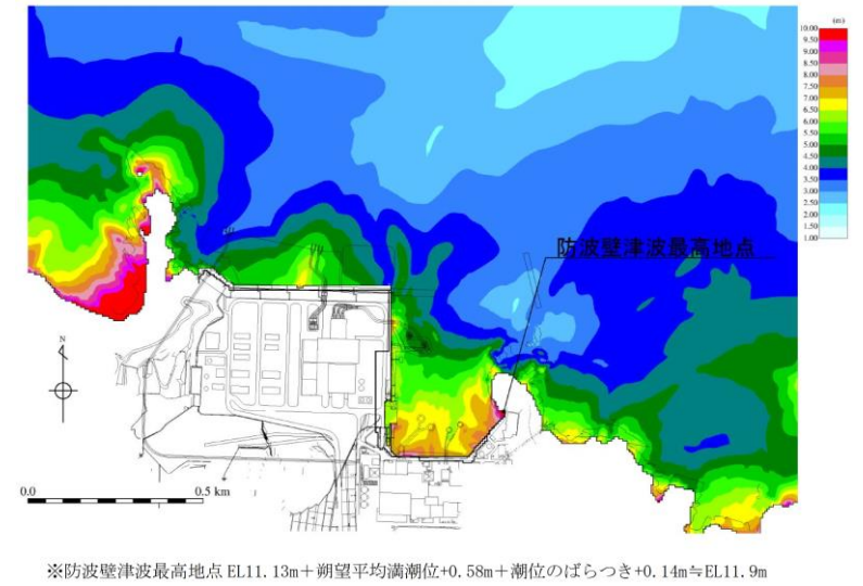
第2.2-1-1図 基準津波の遡上波による最高水位分布 (基準津波1:防波堤無し)
