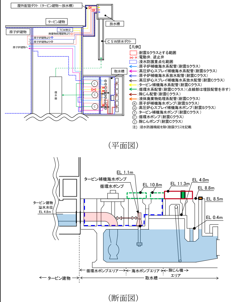
第2.4-8-2図 浸水防護重点化範囲内に設置する海域と接続する低耐震クラスの機器及び配管への対策概要図
