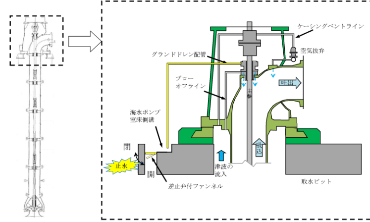
図 2.3-5 海水ポンプグランドドレン配管接続図 (変更後)
