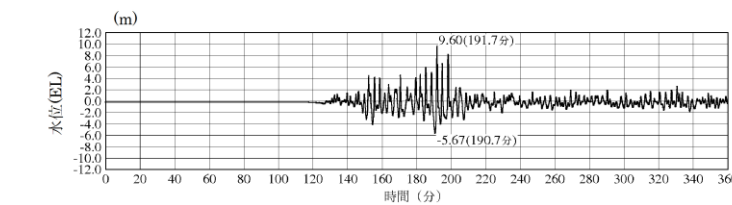
※最大水位下降量-5.67m-地殻変動量 0.34m≒EL-6.1m 2号炉取水槽 (入力津波6, 防波堤無し) ※下降側 ポンプ停止時
