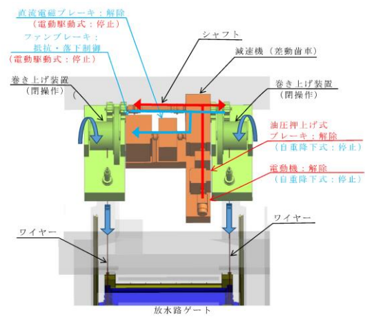
第10.6-3図 放水路ゲート概念図
