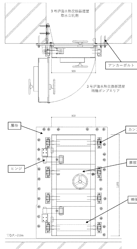
第10.6-8図 水密扉概念図
