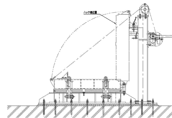
第10.6-9図 浸水防止蓋概念図
