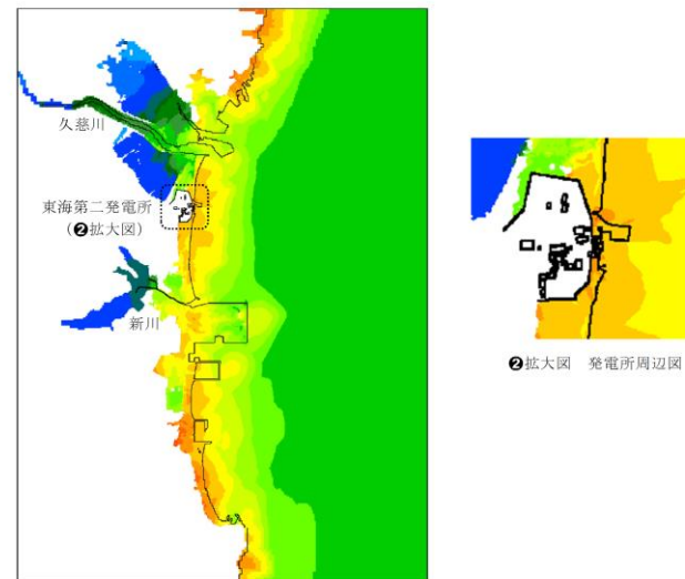
防波堤なし
