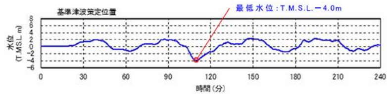
基準津波 2
