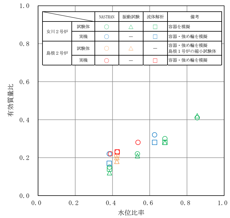
第1図 水位と有効質量比の関係
