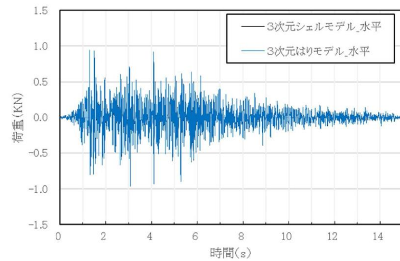
別紙 5-17 図 水平荷重時刻歴 (X方向) の比較 (3次元シェルモデル, 3次元はりモデル)
