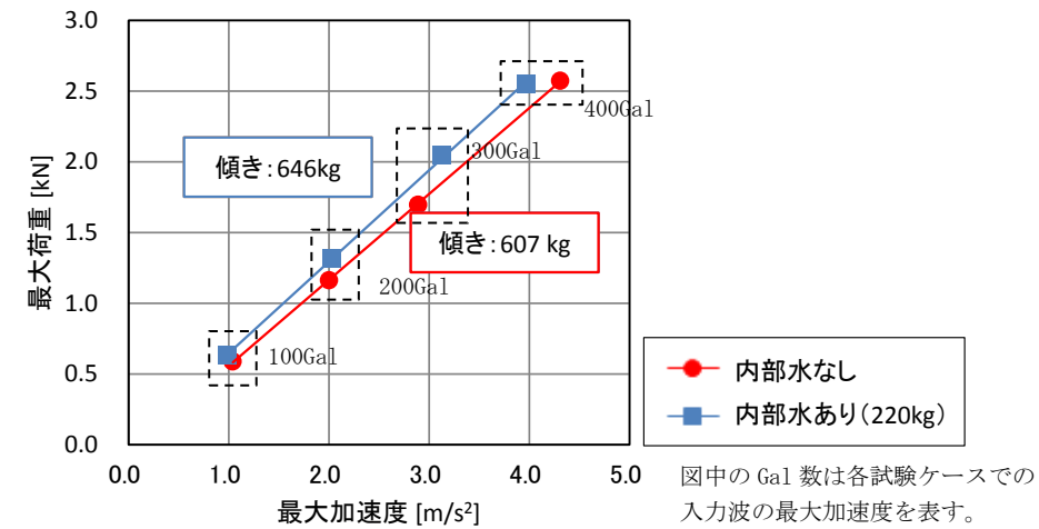
第 3.3-2 図 振動試験における最大加速度と最大荷重の関係 (ランダム波A) (本文第 4.2-8 図の再掲)
