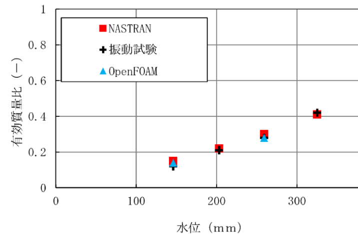
第4.4-1図 各手法の有効質量比の評価結果
