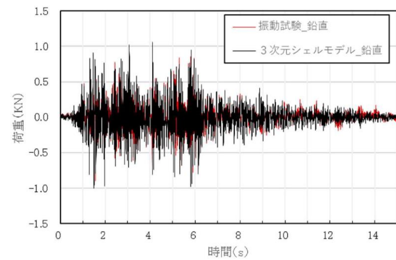
別紙 5-16 図 鉛直荷重時刻歴 (Z方向) の比較 (振動試験, 3次元シェルモデル)
