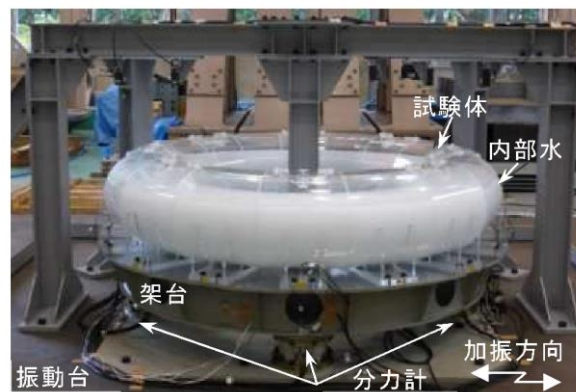
第4.2-2 図 試験装置の写真
