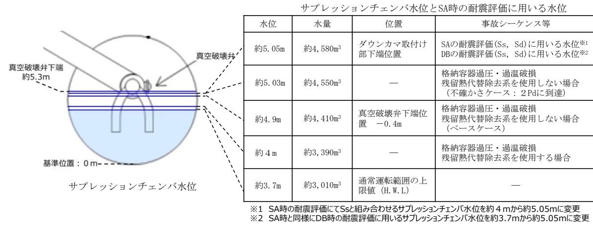
第1図 重大事故時のサプレッションチェンバの水位と耐震評価に用いる水位との関係
