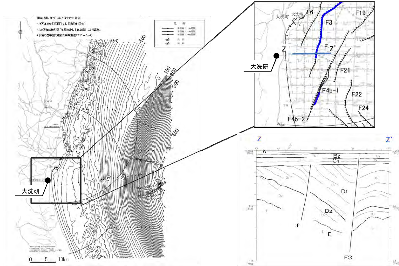
Z-Z' 断面
