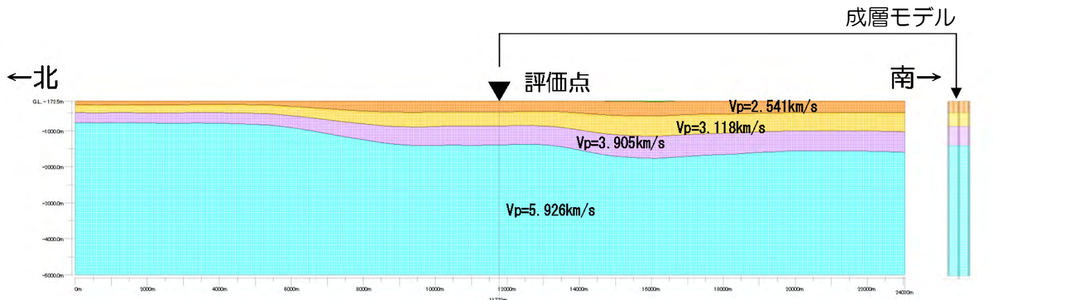
2次元FEMモデル（南北断面）
