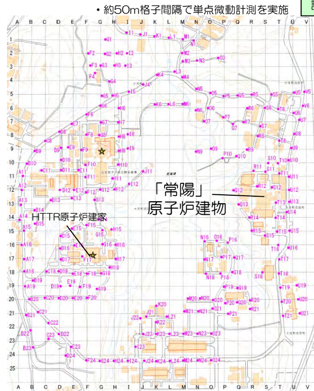
大洗研の測定位置図
