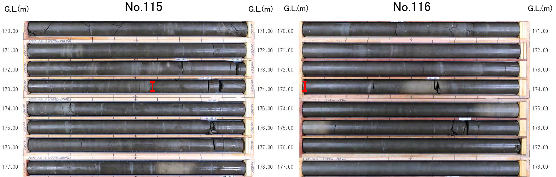
I 解放基盤表面設定深度 (T.P.-135m)
