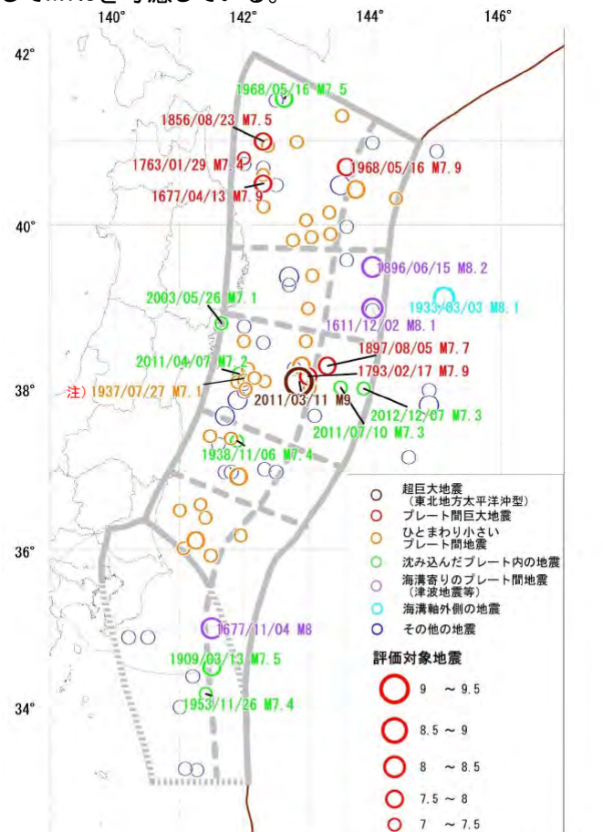
注) 沈み込んだプレート内の地震の可能性もある。 地震本部(2019)
