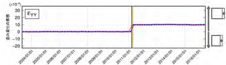
ひずみ変化の累積(大洗研敷地周辺)
