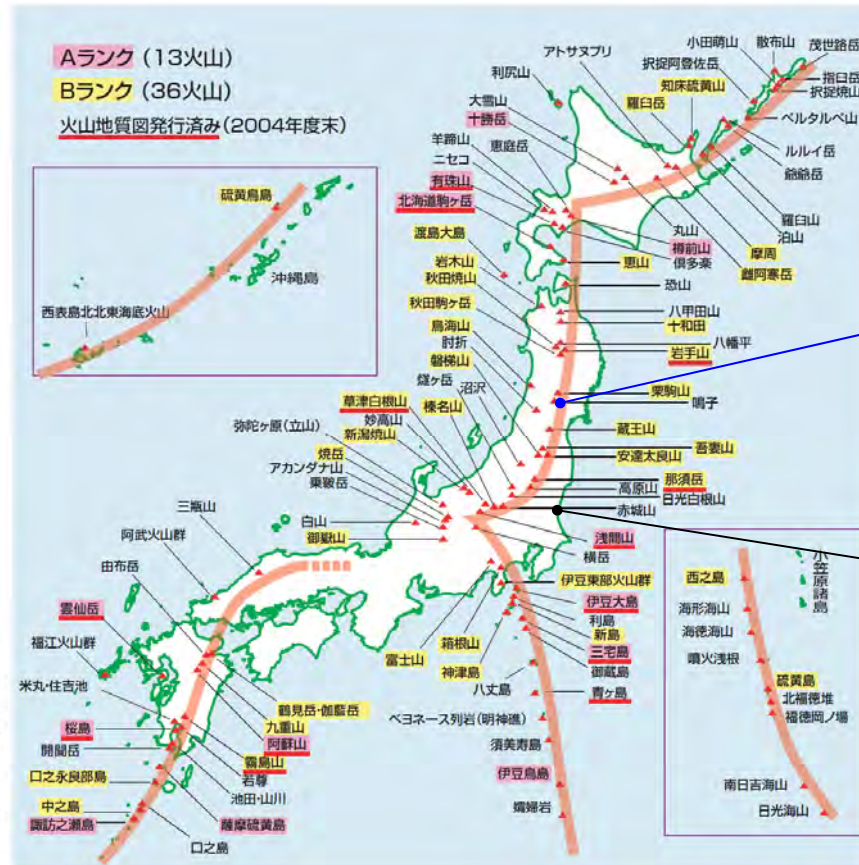
火山フロント 産業技術総合研究所(2004)に一部加筆
