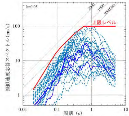
図8 震源を事前に特定できない地震による震源近傍の観測記録の水平動応答スペクトルとその上限レベル (実線は1997年鹿児島県北西部地震の鶴田ダムのスペクトル、破線はスケージングの観点から確実に事前に震源を特定できるとは断定できないと判断したMj6.5(Mw6.2)以下の7地震のスペクトル)
