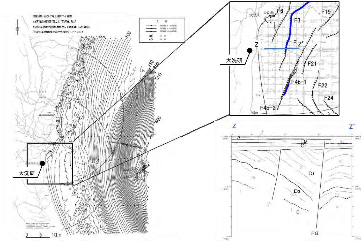
Z-Z' 断面
