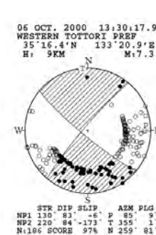
P波初動による発震機構解 気象庁(2000)より抜粋
