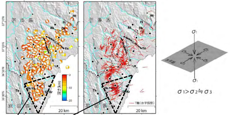
図11 得られたメカニズム解とT軸の分布 左：下半球投影のメカニズム解。深さで色分けした。井戸沢断層(It)と湯ノ岳断層(Yn)の地表地震断層 (Mizoguchi et al., in preparation) を○で示す。中：メカニズム解のT軸方位 (水平投影)。右：推定される応力場の概念図。
