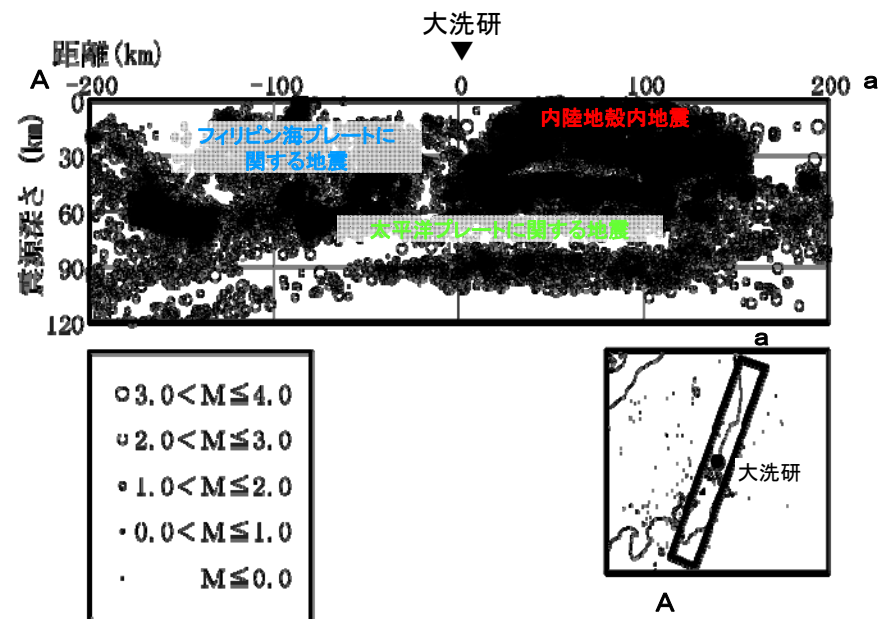
(気象庁, 2011年3月～2015年12月)
