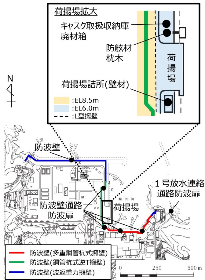
図－1 3 漂流物配置位置
