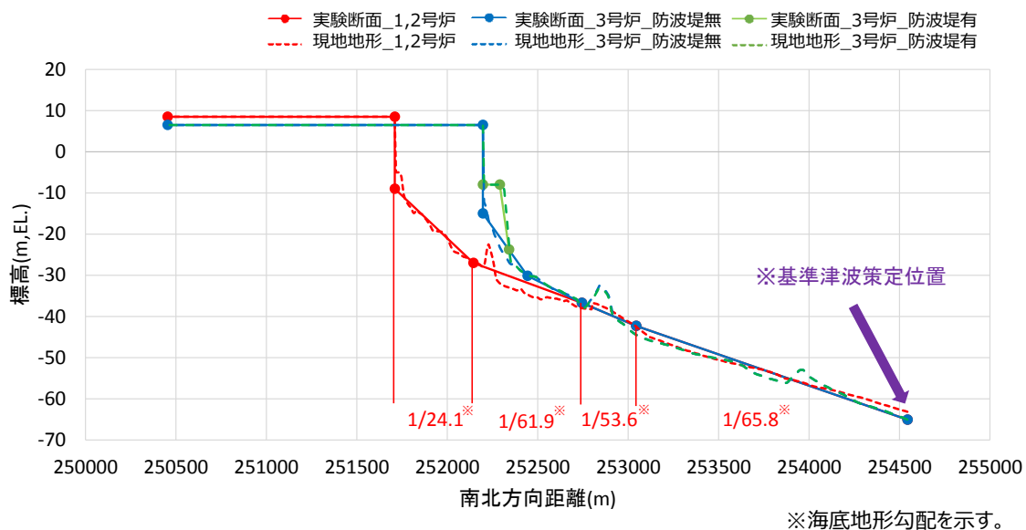
第15図 検討断面図
