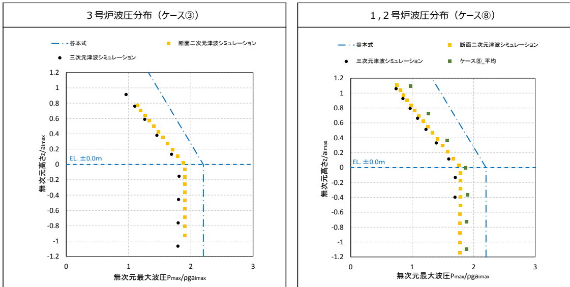
第58図 断面二次元津波シミュレーション, 三次元津波シミュレーション, 水理模型実験(1, 2号炉), 既往の算定式(谷本式)により算定した波圧分布
