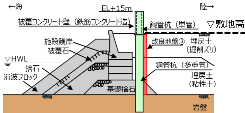
第50図(1) 防波壁(多重鋼管杭式擁壁)断面図
