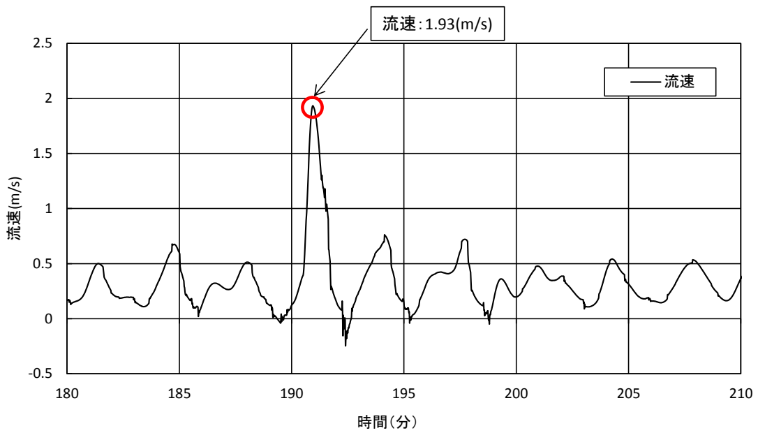
第 2.5-30 図 流速評価結果 (入力津波 6)
