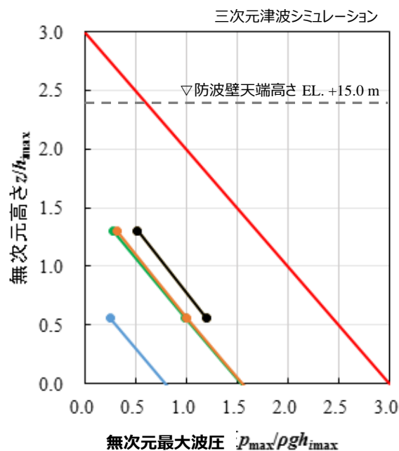
第56図 無次元最大波圧分布 (3号炉東側前面)
