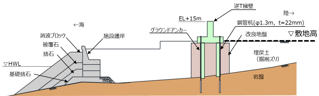
第50図(3) 防波壁(鋼管杭式逆T擁壁)断面図
