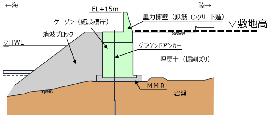
第50図(2) 防波壁(波返重力擁壁)断面図
