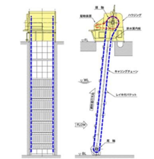
第 2.5-28 図 除塵装置の概要
