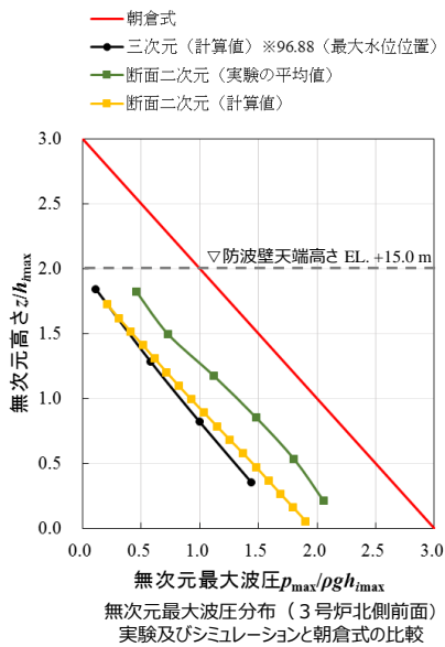
第54図 無次元最大波圧分布 (3号炉北側前面)
