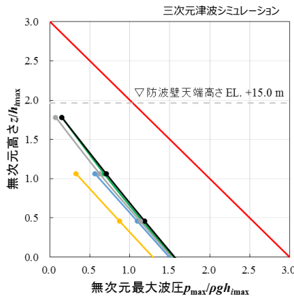
無次元最大波圧分布 (1, 2号炉前面) 三次元津波シミュレーションと朝倉式の比較
