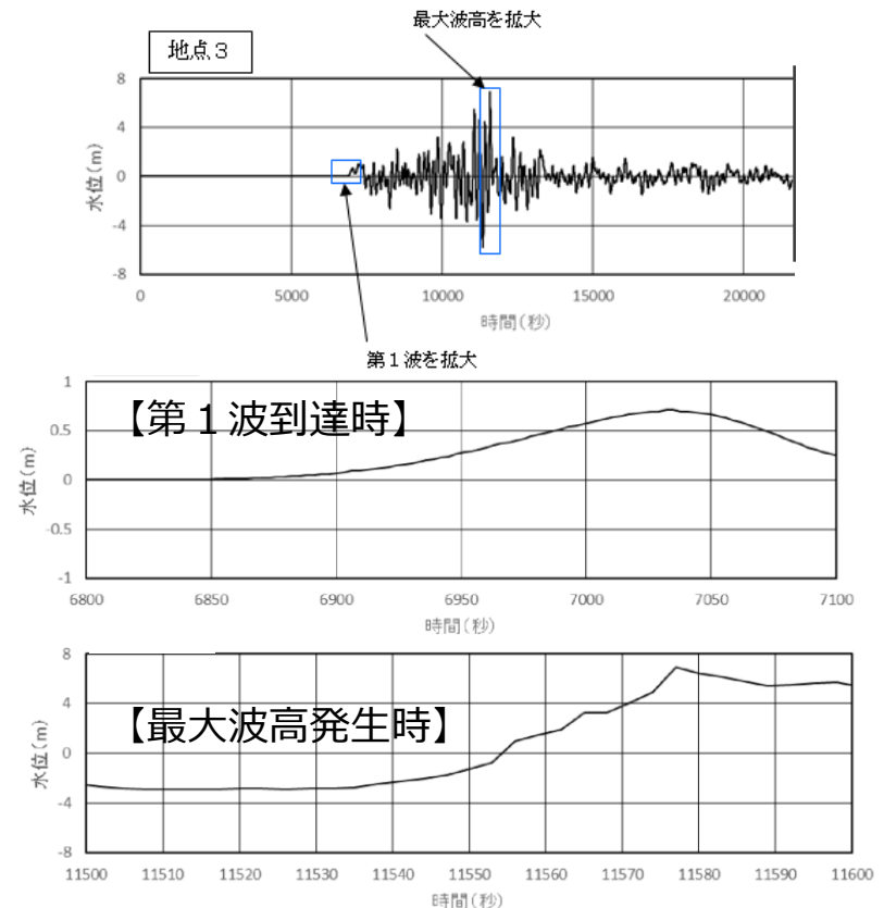
津波高さの時刻歴波形図(地点3，基準津波1：防波堤無)
