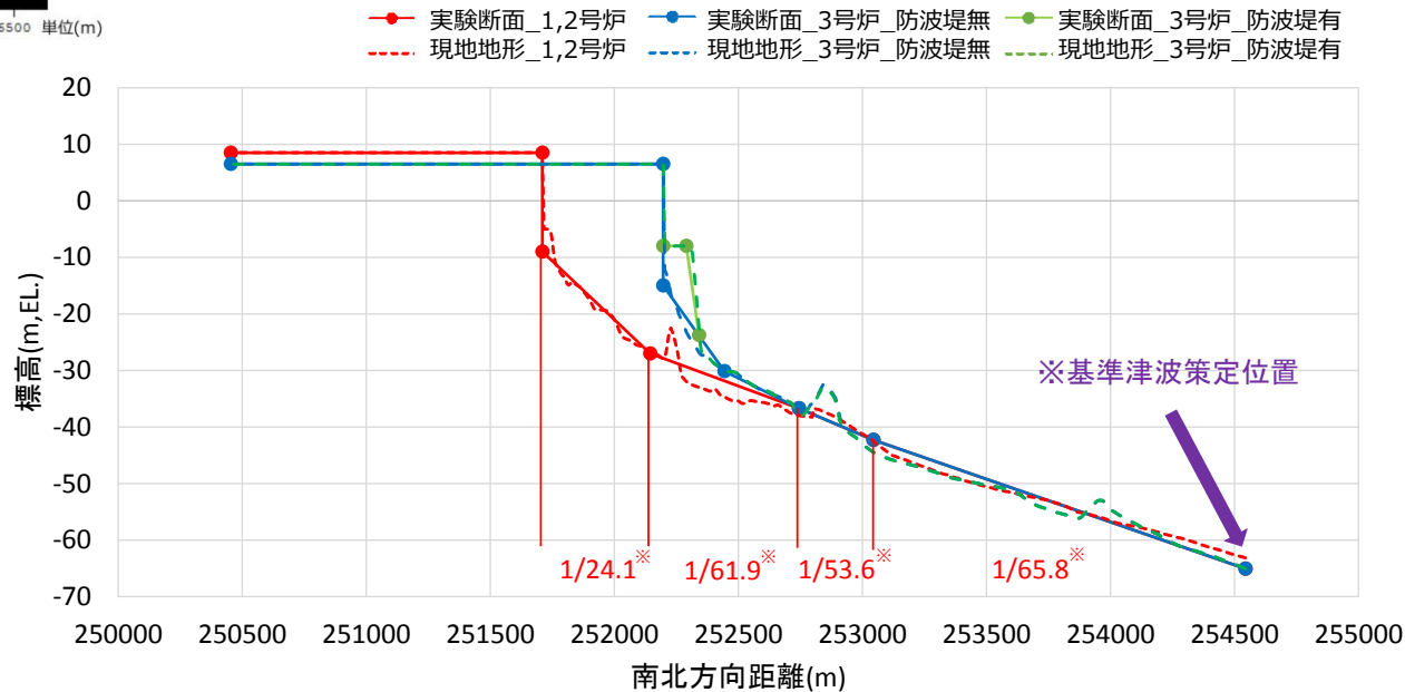
検討断面図
