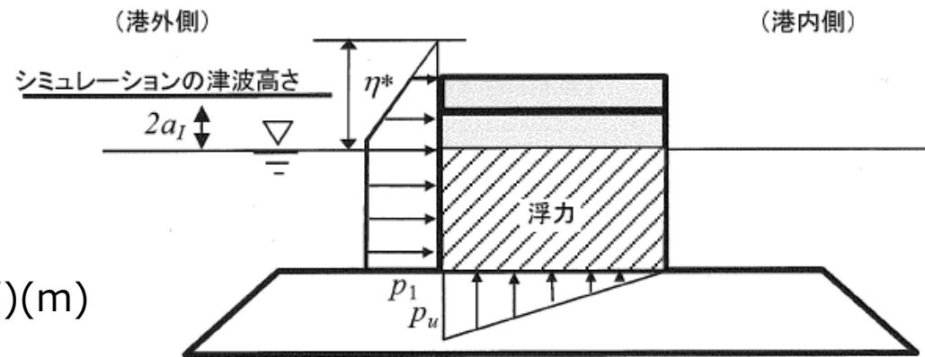
谷本式による波圧分布 (背面水位が押し波時に静水面より下がらない場合)
