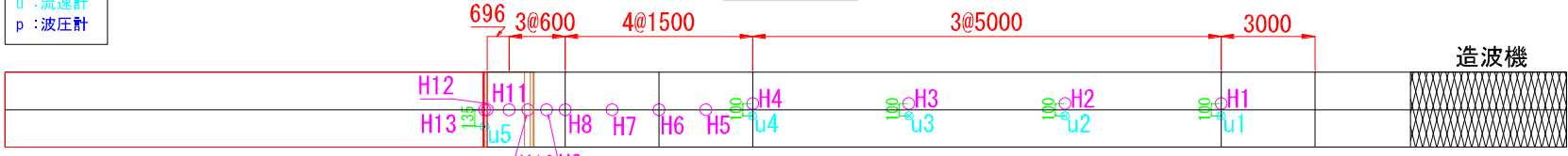
断面図
