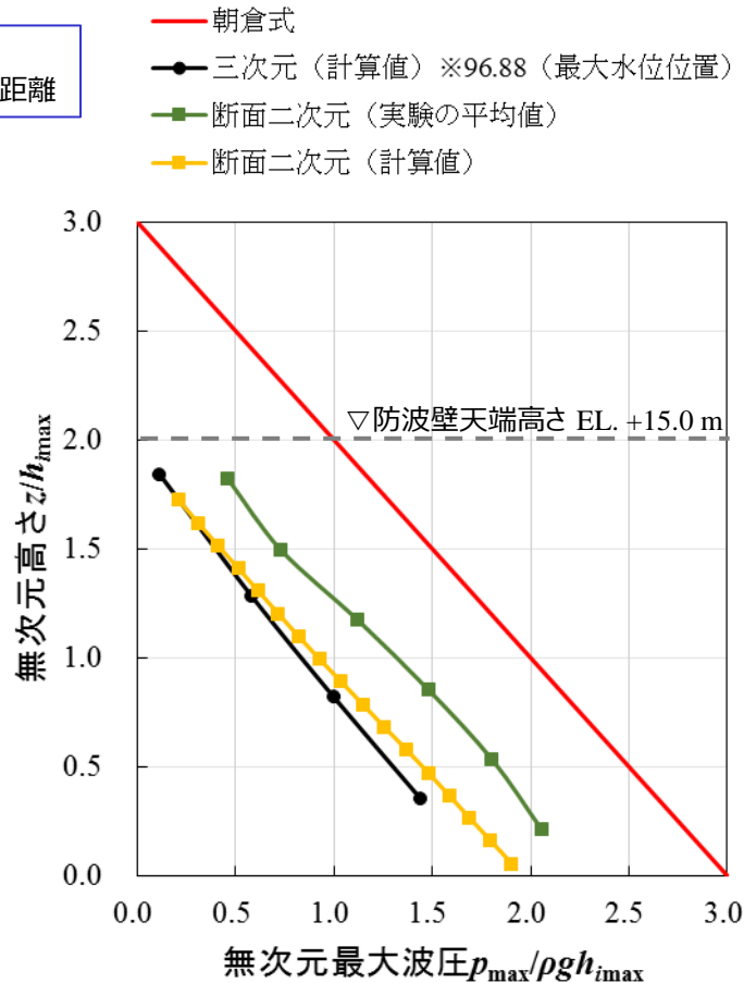
無次元最大波圧分布（3号炉北側前面） 実験及びシミュレーションと朝倉式の比較
