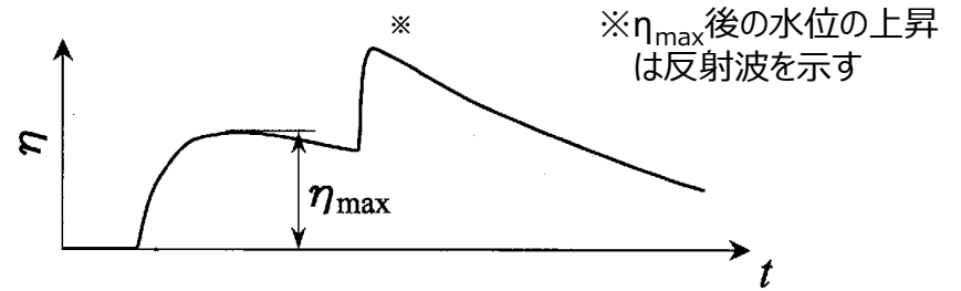
非分裂波の最大遡上水深
