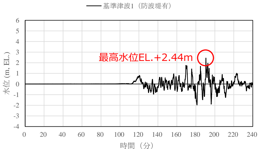
入射津波の造波波形図（防波堤有）
