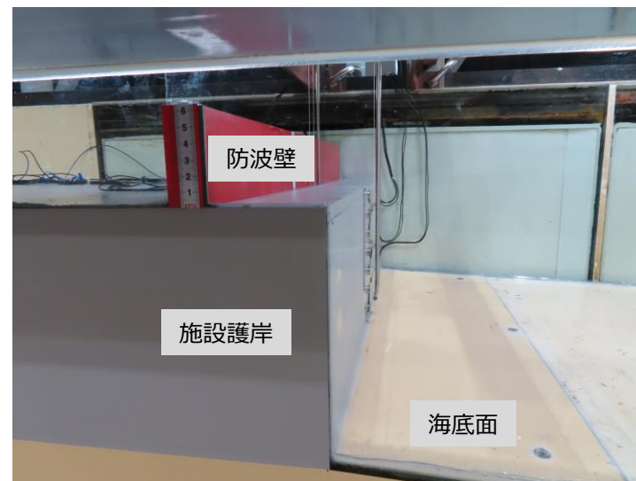
側面
