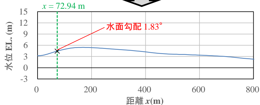
水位分布の拡大図 (t = 254.4s)
