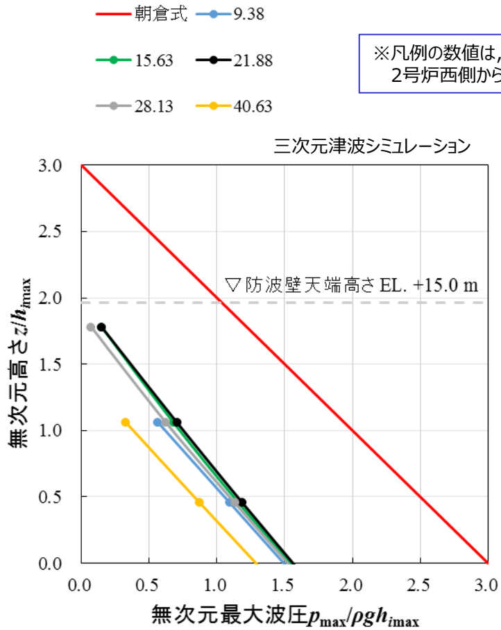
無次元最大波圧分布（1, 2号炉前面） 三次元津波シミュレーションと朝倉式の比較
