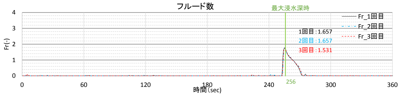
最大浸水深及び同時刻におけるフルード数（進行波成分）の時刻歴波形
