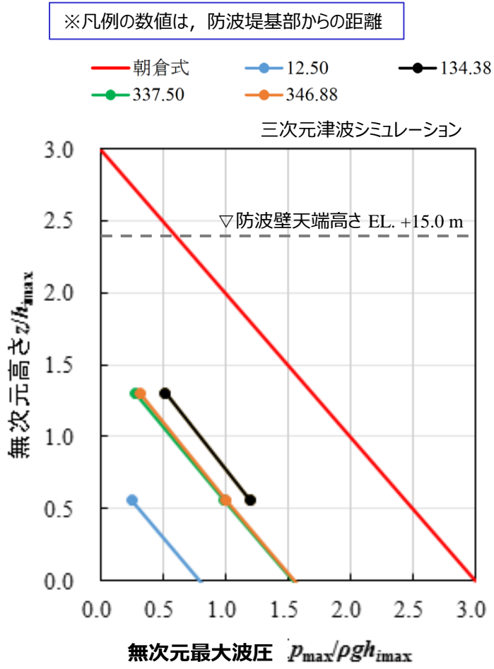
無次元最大波圧分布（3号炉東側前面）
