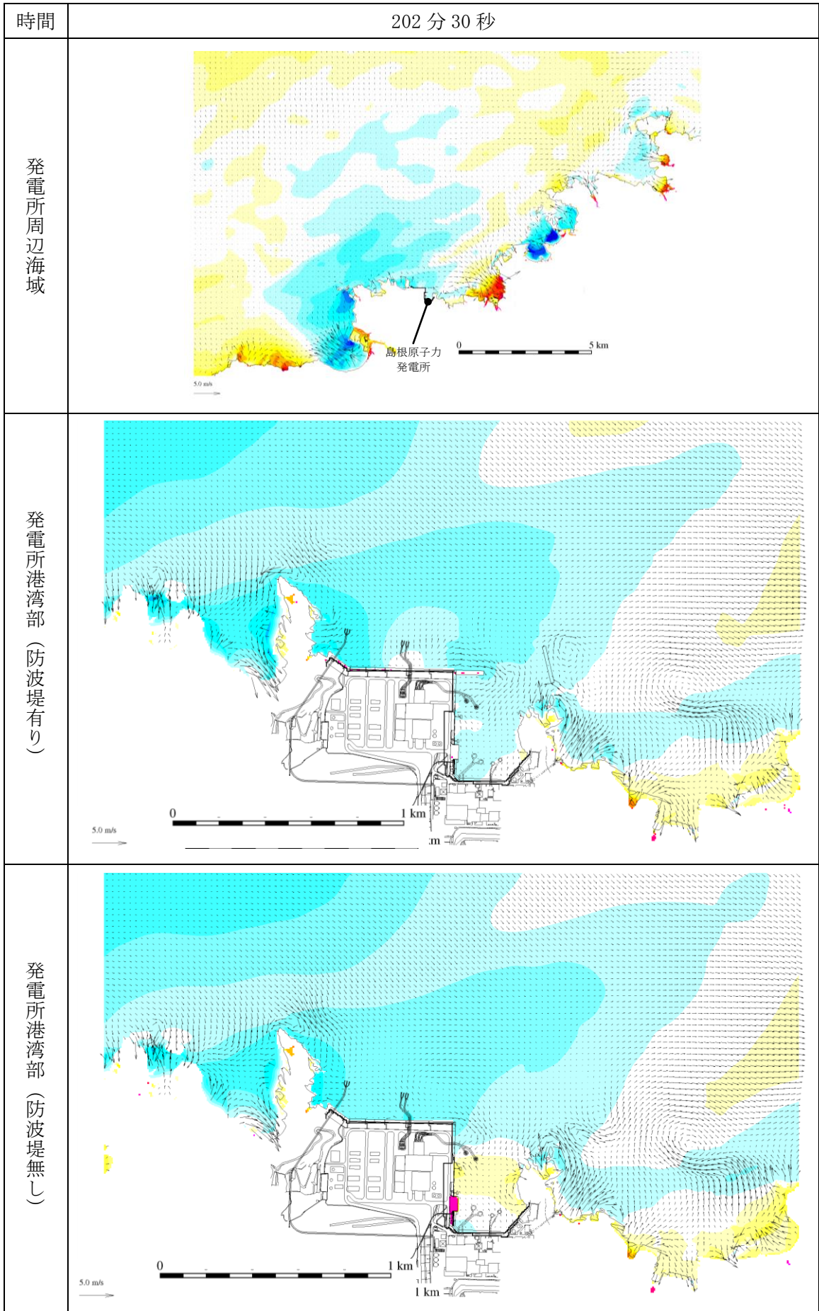
第 1 図 (206) 基準津波 1 の水位変動・流向ベクトル
