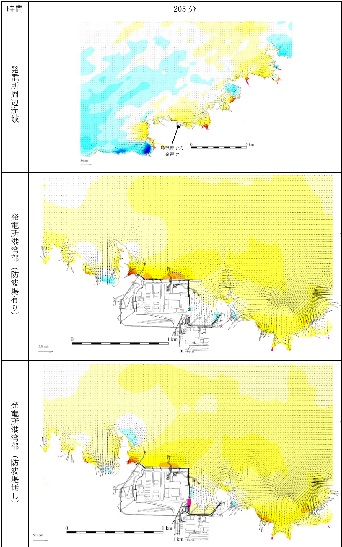
第 1 図 (211) 基準津波 1 の水位変動・流向ベクトル
