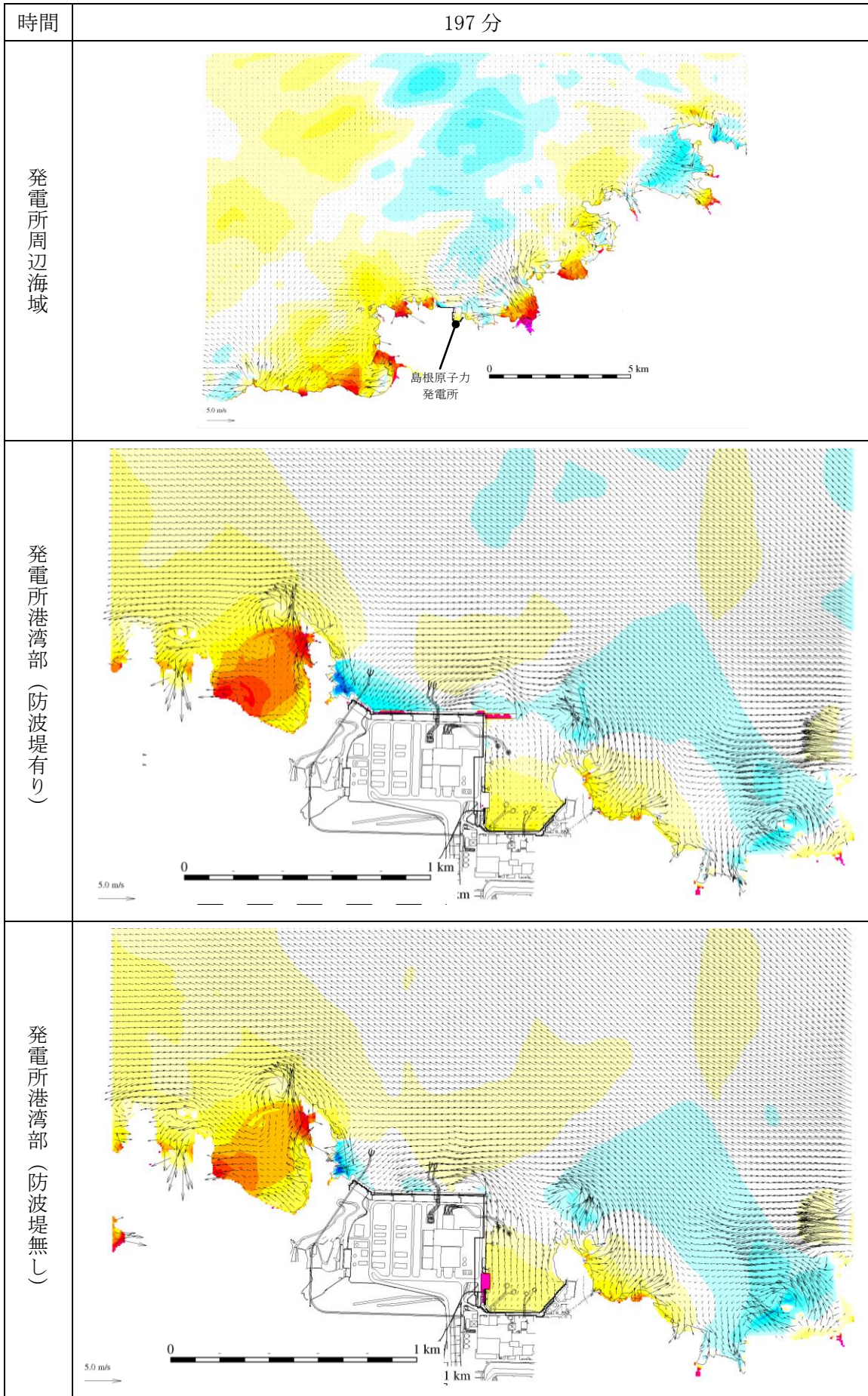
第 1 図(195) 基準津波 1 の水位変動・流向ベクトル
