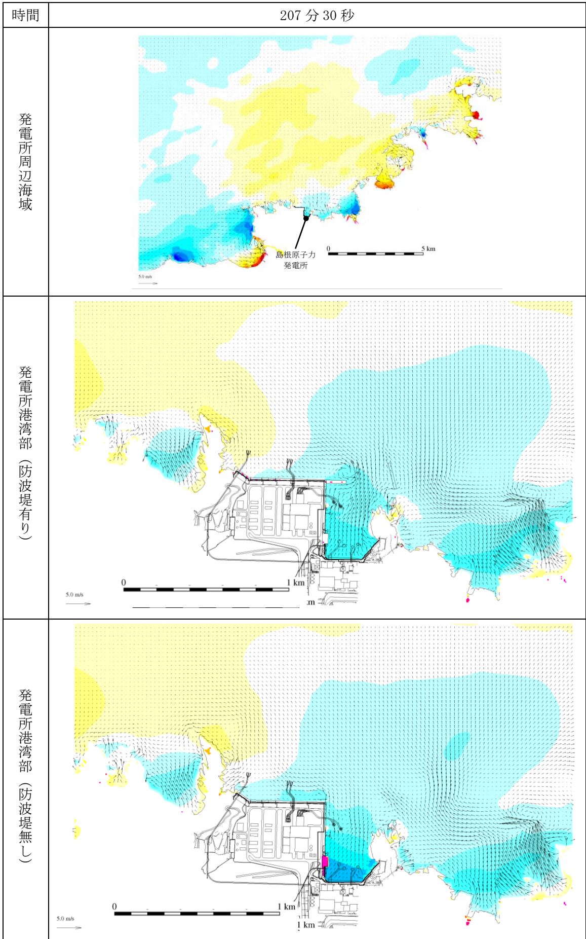
第 1 図 (216) 基準津波 1 の水位変動・流向ベクトル
