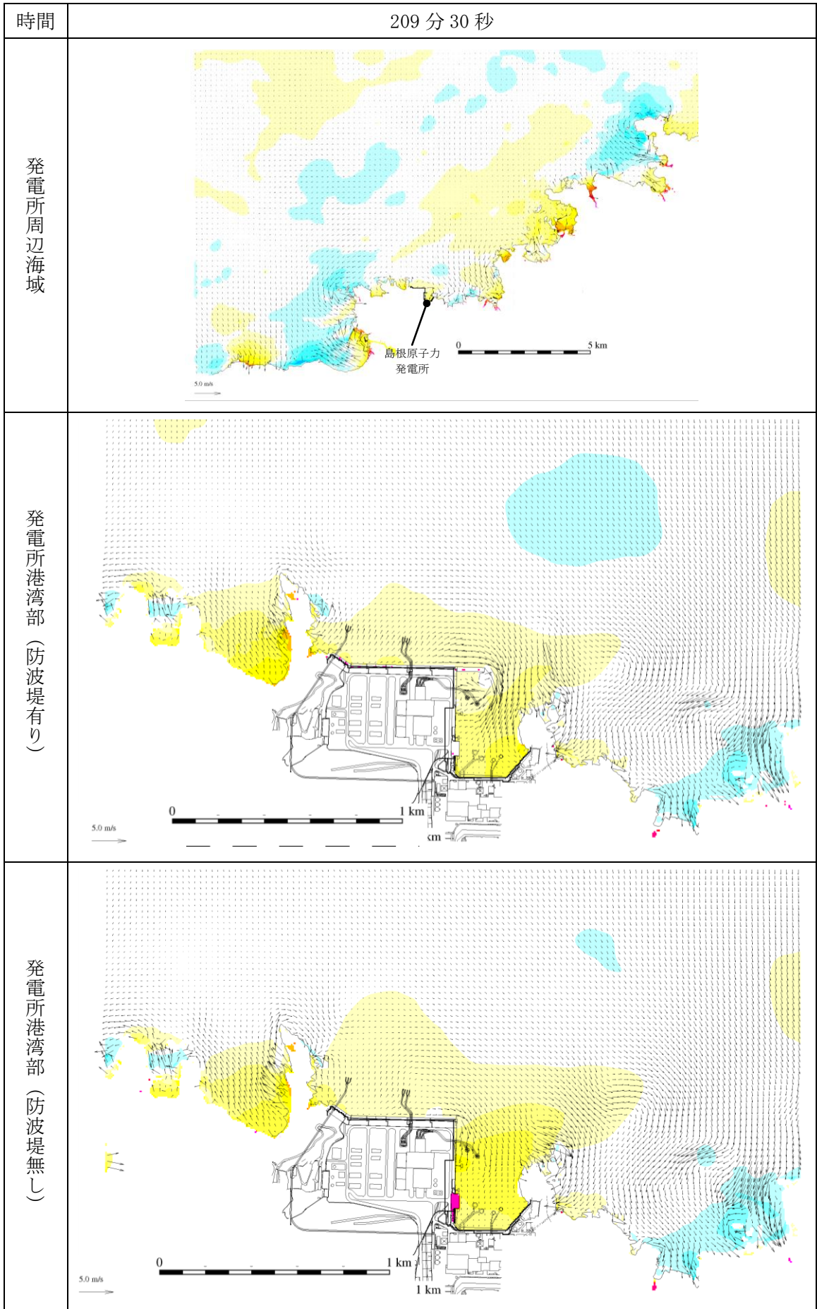
第 1 図 (220) 基準津波 1 の水位変動・流向ベクトル
