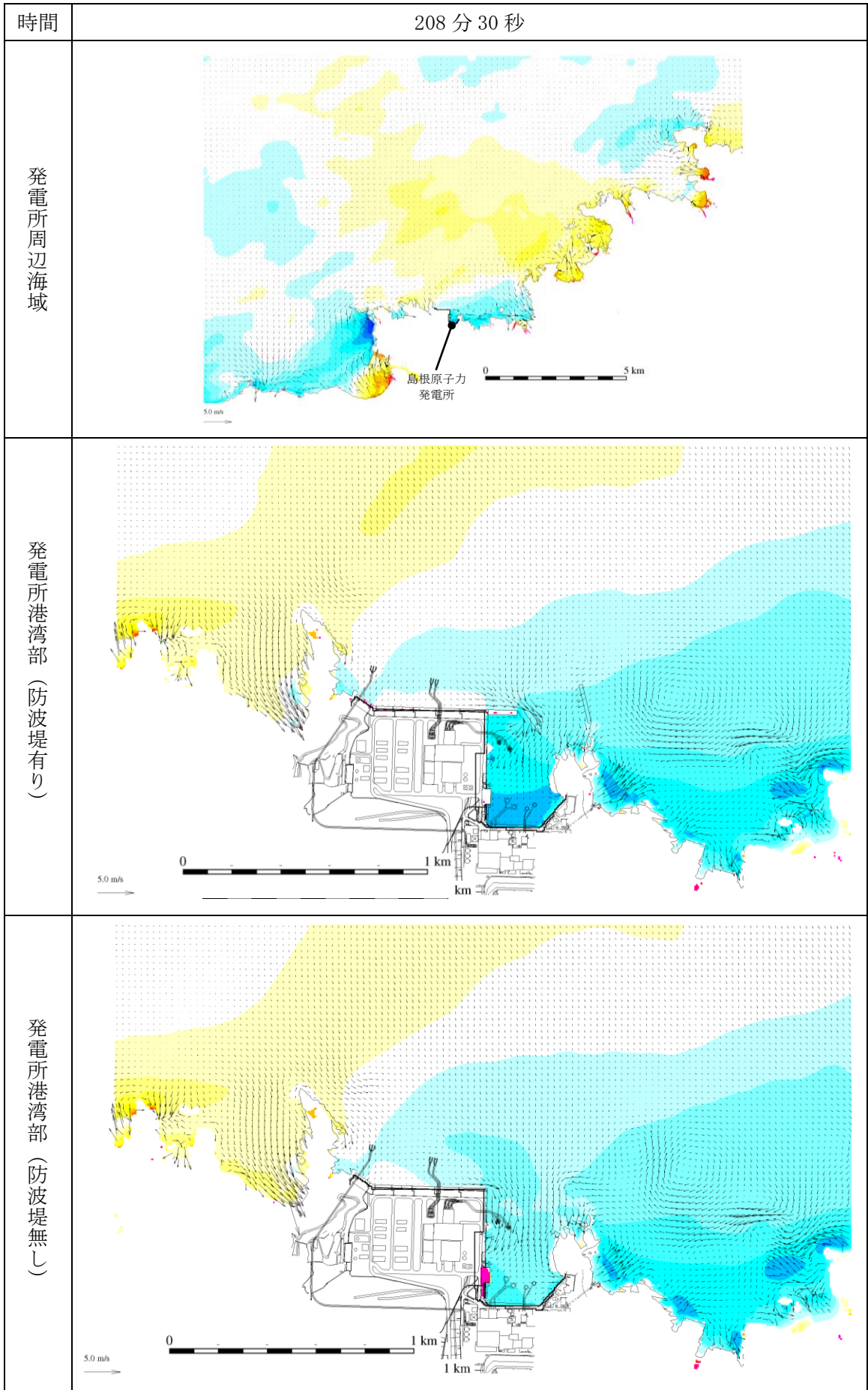
第 1 図 (218) 基準津波 1 の水位変動・流向ベクトル
