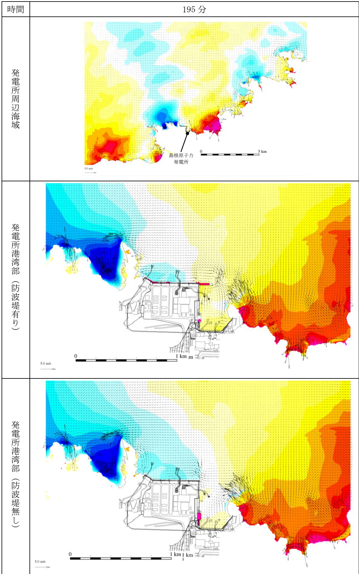
第 1 図(191) 基準津波 1 の水位変動・流向ベクトル
