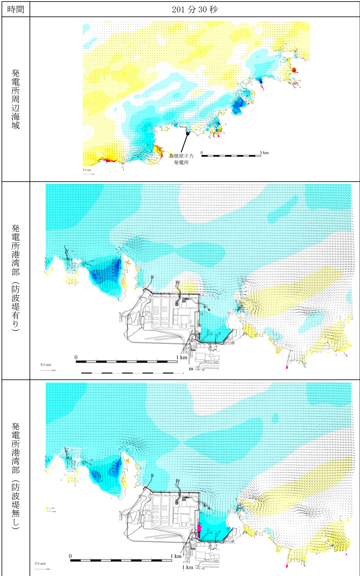
第 1 図 (204) 基準津波 1 の水位変動・流向ベクトル
