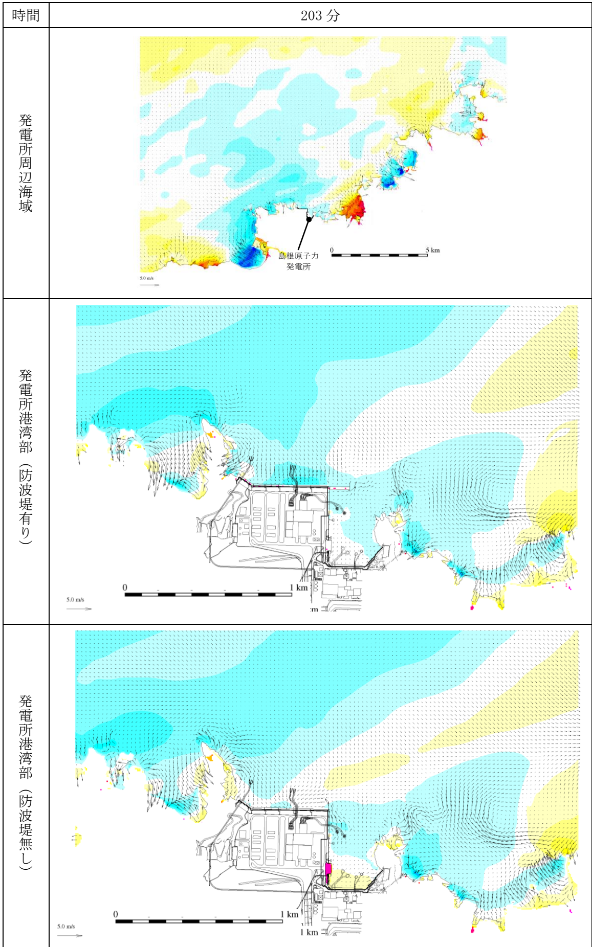
第 1 図 (207) 基準津波 1 の水位変動・流向ベクトル
