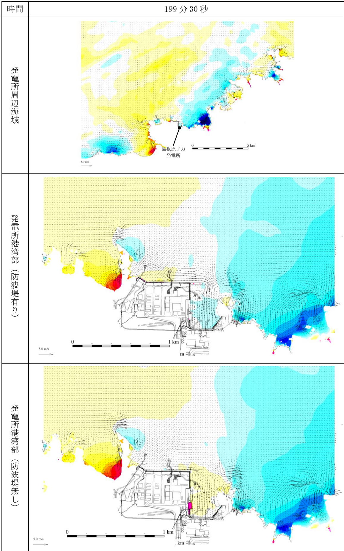
第 1 図 (200) 基準津波 1 の水位変動・流向ベクトル
