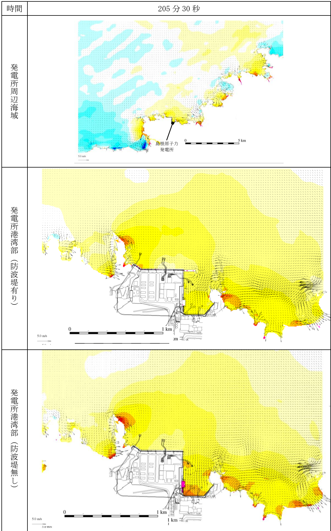
第 1 図 (212) 基準津波 1 の水位変動・流向ベクトル
