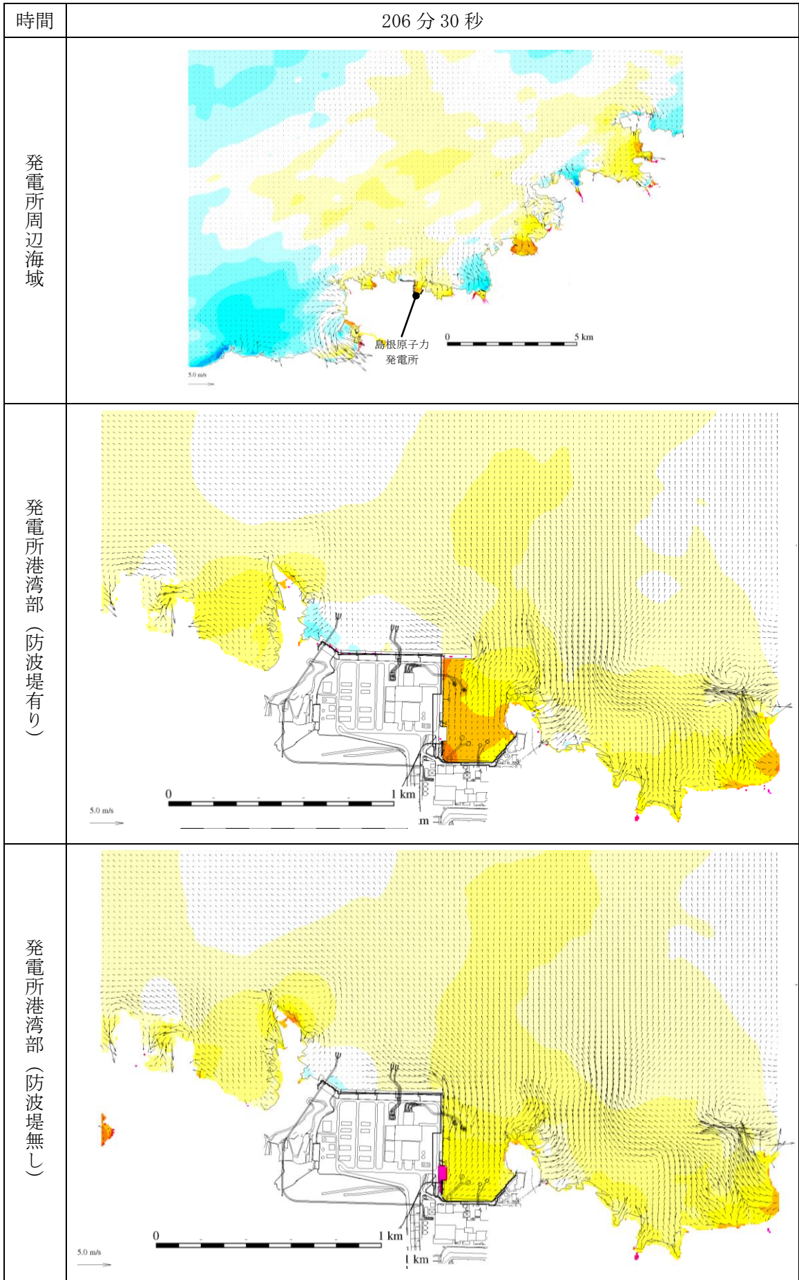
第 1 図 (214) 基準津波 1 の水位変動・流向ベクトル
