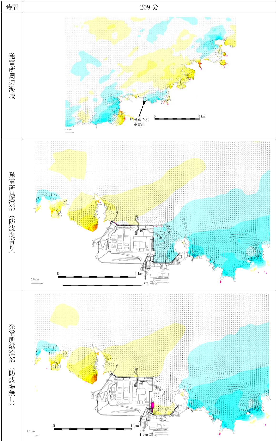
第 1 図 (219) 基準津波 1 の水位変動・流向ベクトル
