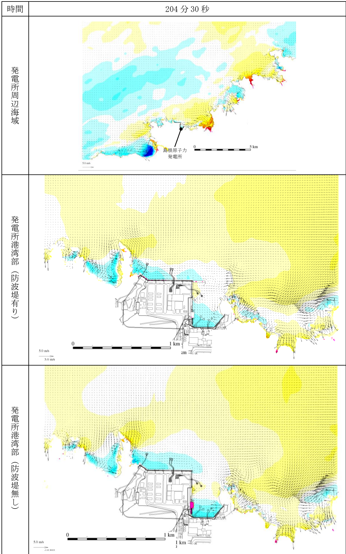
第 1 図 (210) 基準津波 1 の水位変動・流向ベクトル
