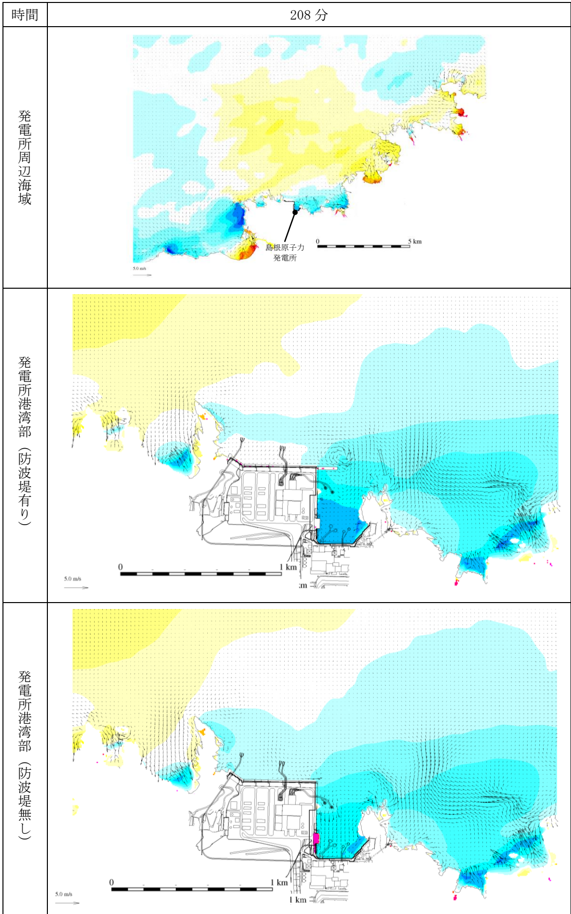
第 1 図 (217) 基準津波 1 の水位変動・流向ベクトル
