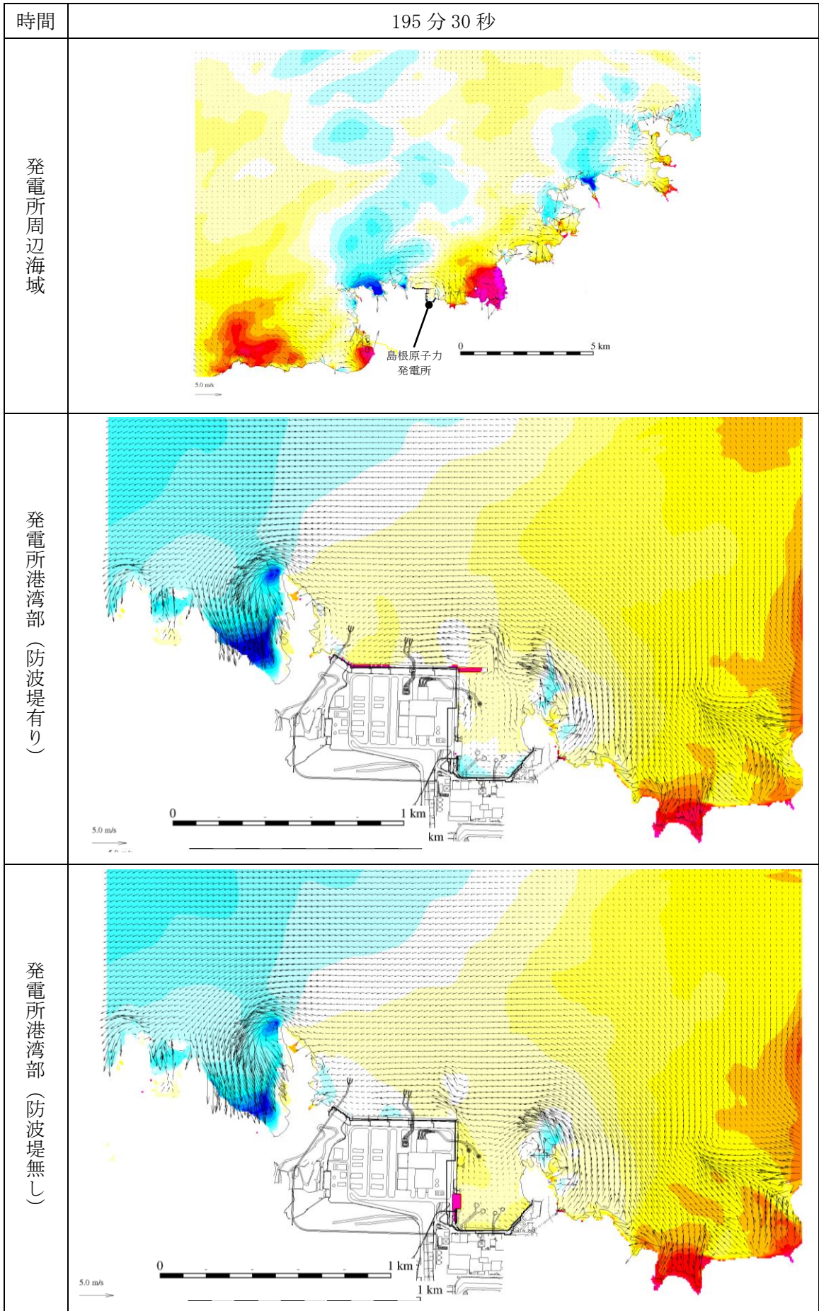
第 1 図(192) 基準津波 1 の水位変動・流向ベクトル
