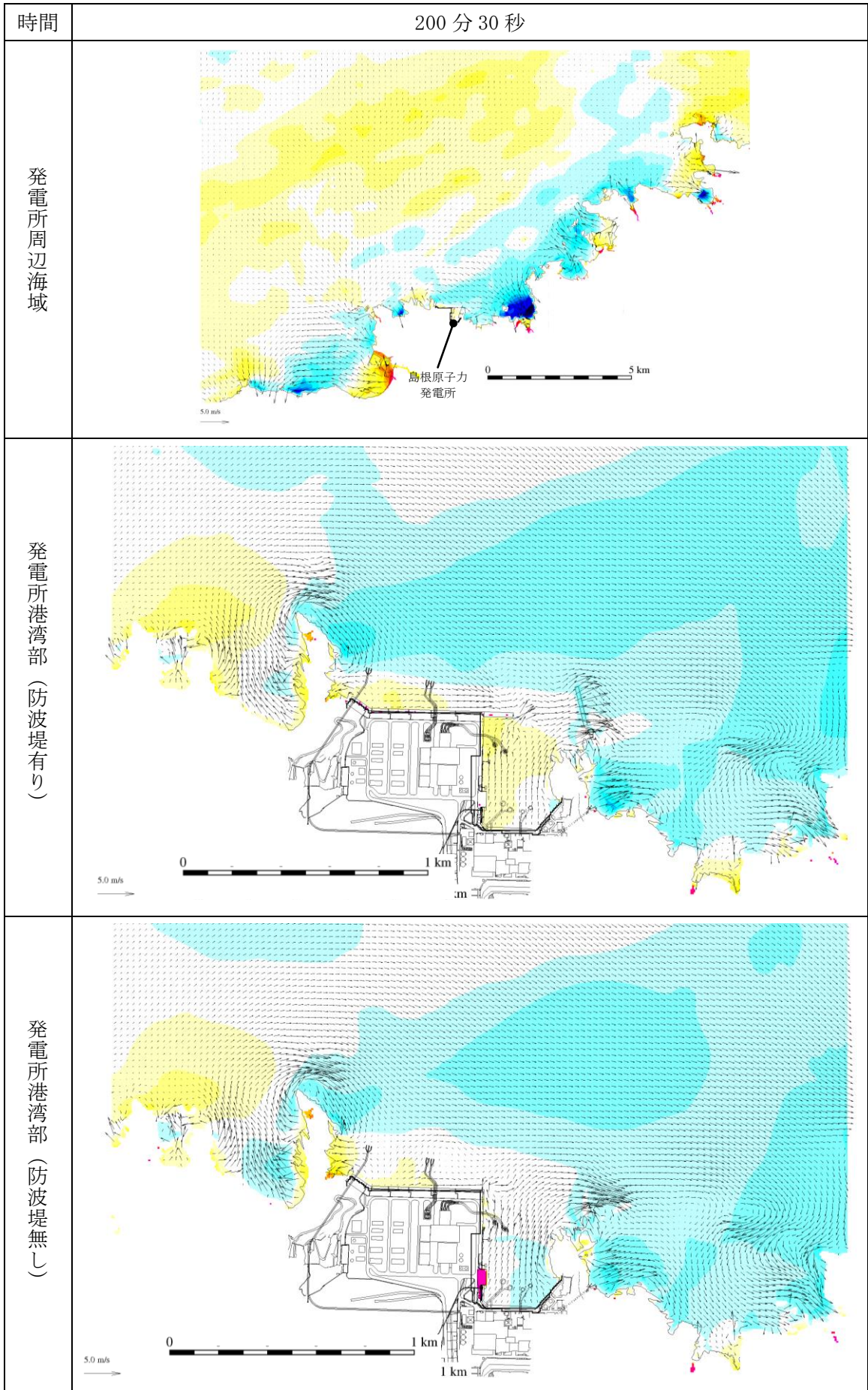
第 1 図 (202) 基準津波 1 の水位変動・流向ベクトル
