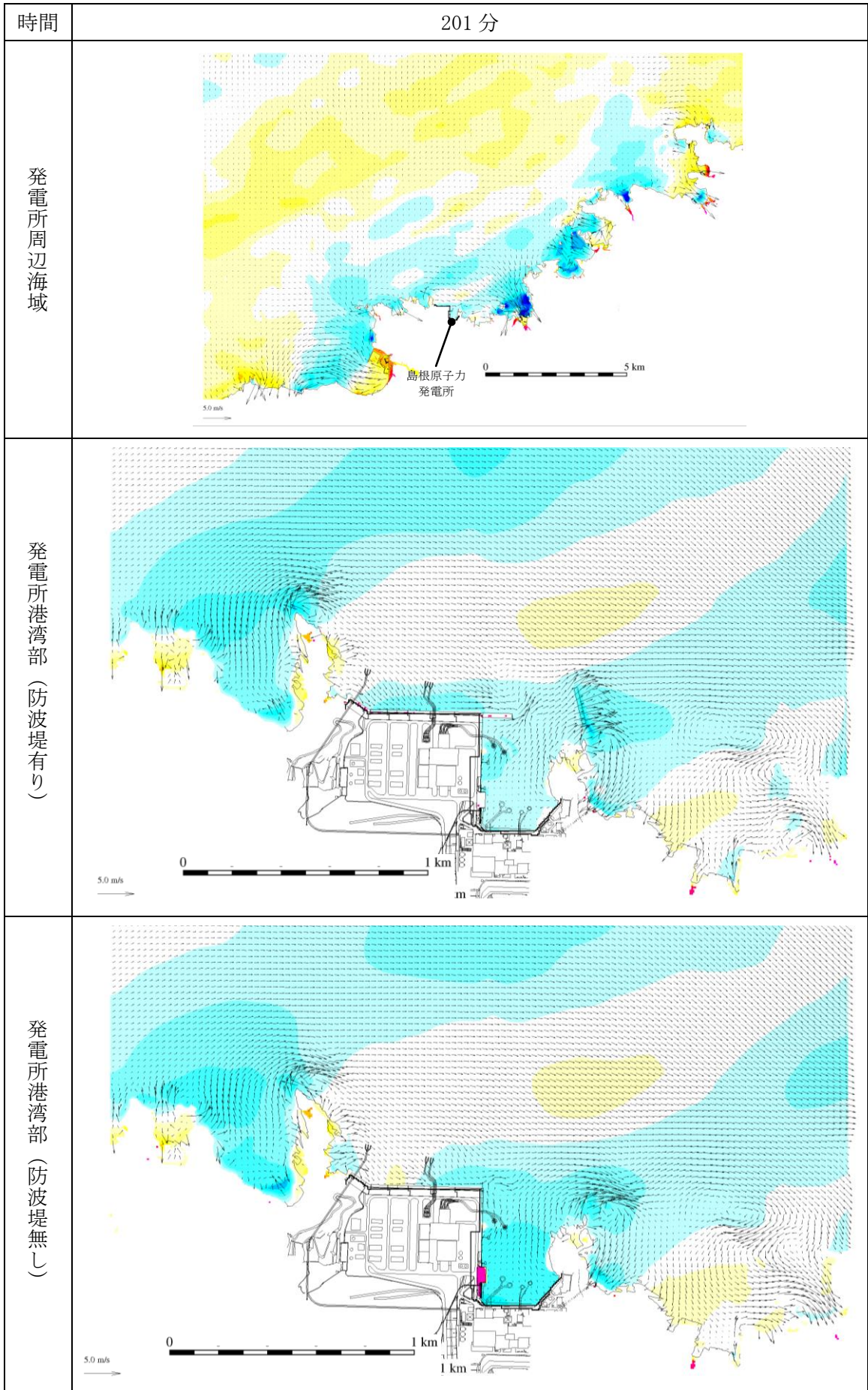
第 1 図 (203) 基準津波 1 の水位変動・流向ベクトル
