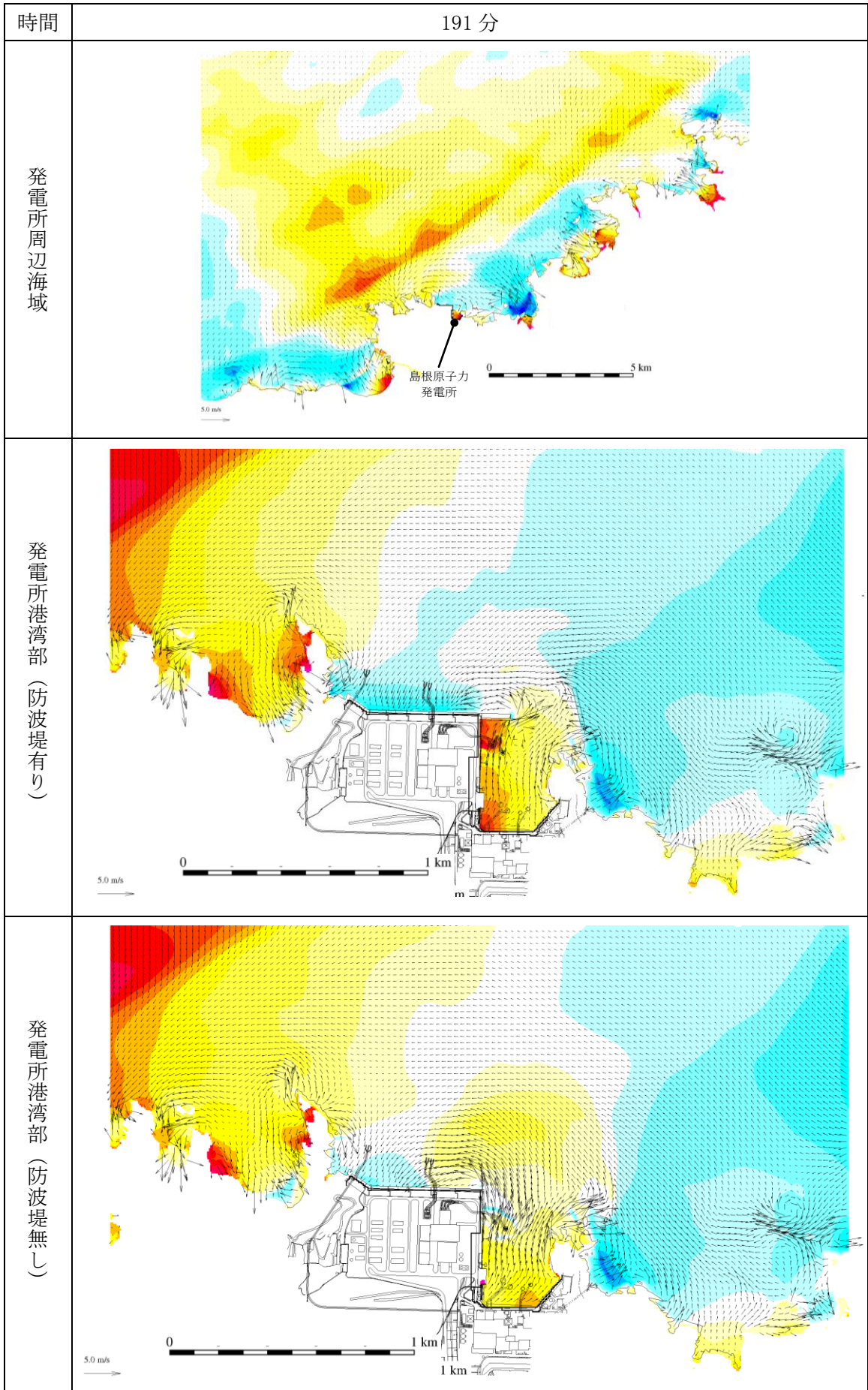
第 1 図(183) 基準津波 1 の水位変動・流向ベクトル
