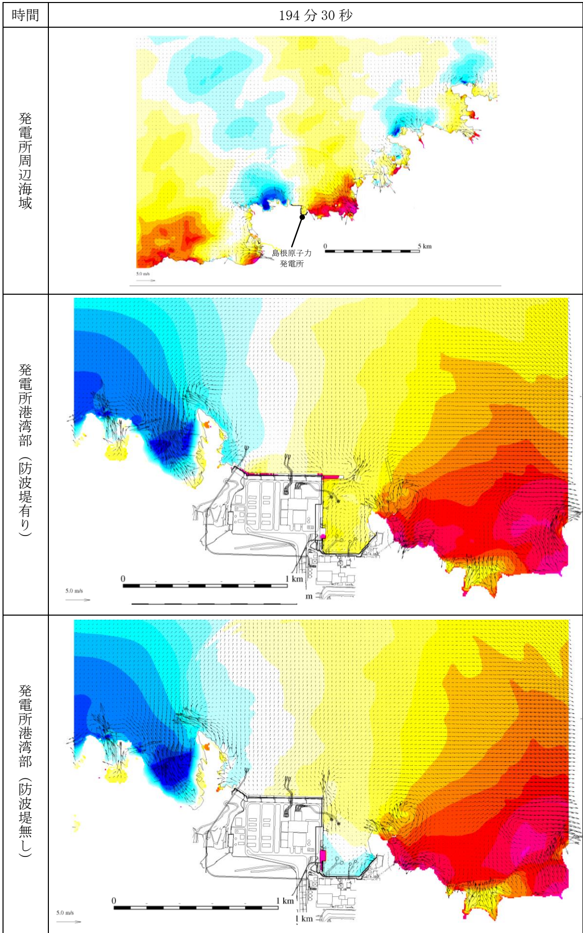
第 1 図(190) 基準津波 1 の水位変動・流向ベクトル
