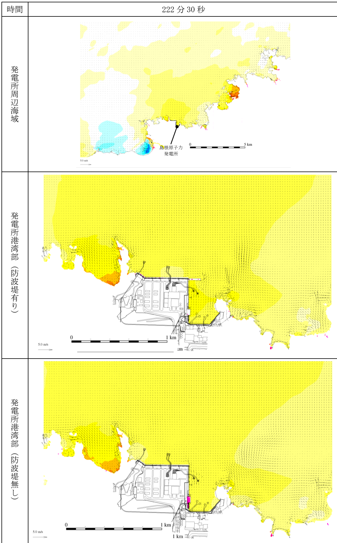
第 1 図 (246) 基準津波 1 の水位変動・流向ベクトル
