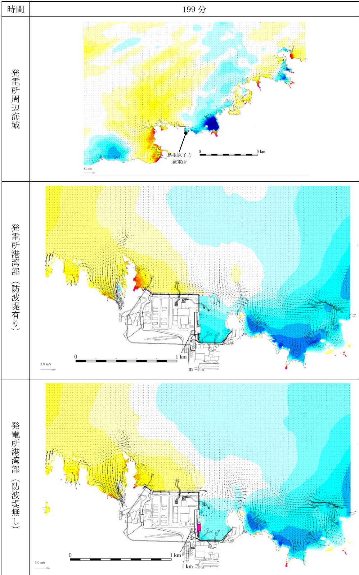
第 1 図(199) 基準津波 1 の水位変動・流向ベクトル
