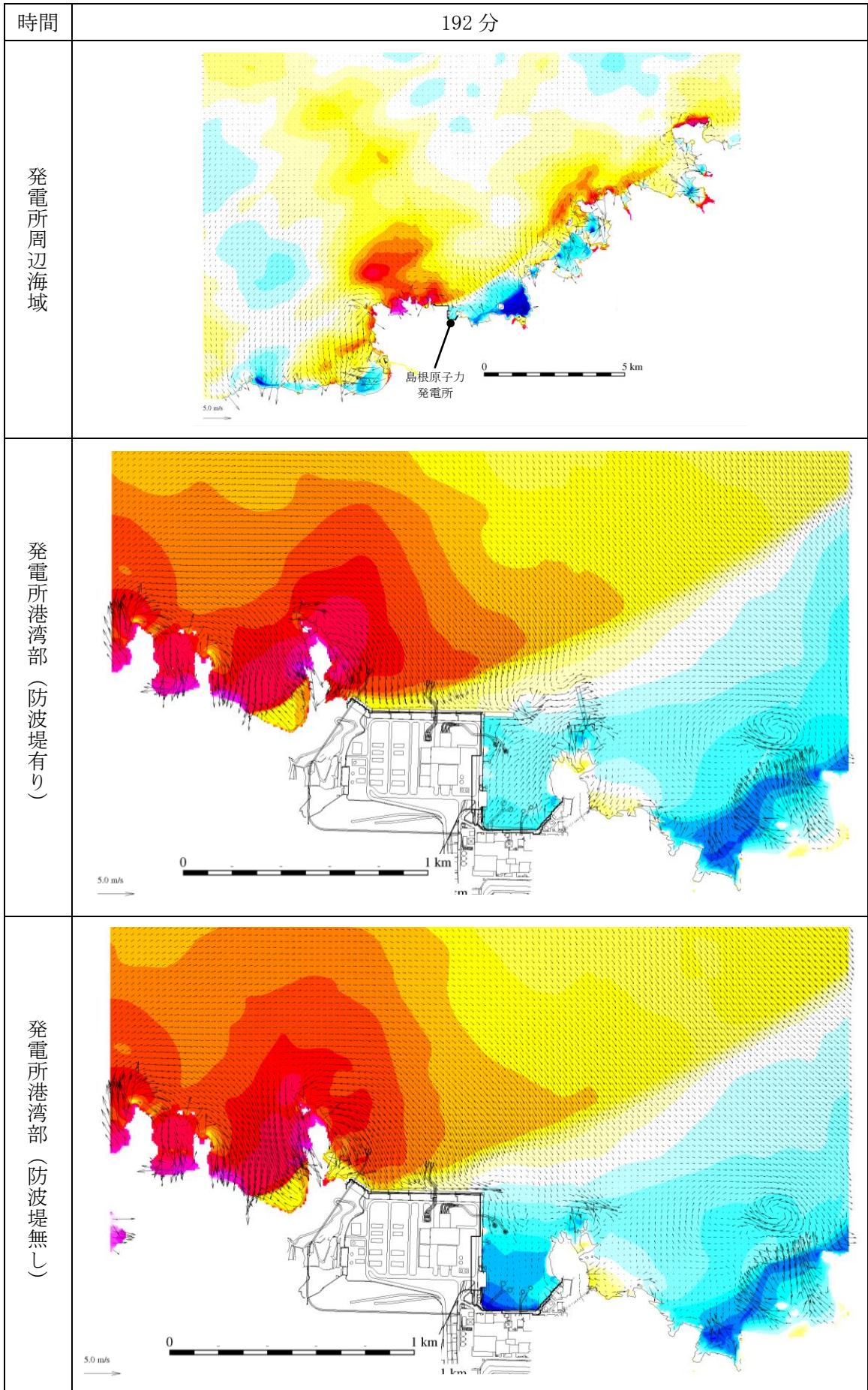
第 1 図(185) 基準津波 1 の水位変動・流向ベクトル
