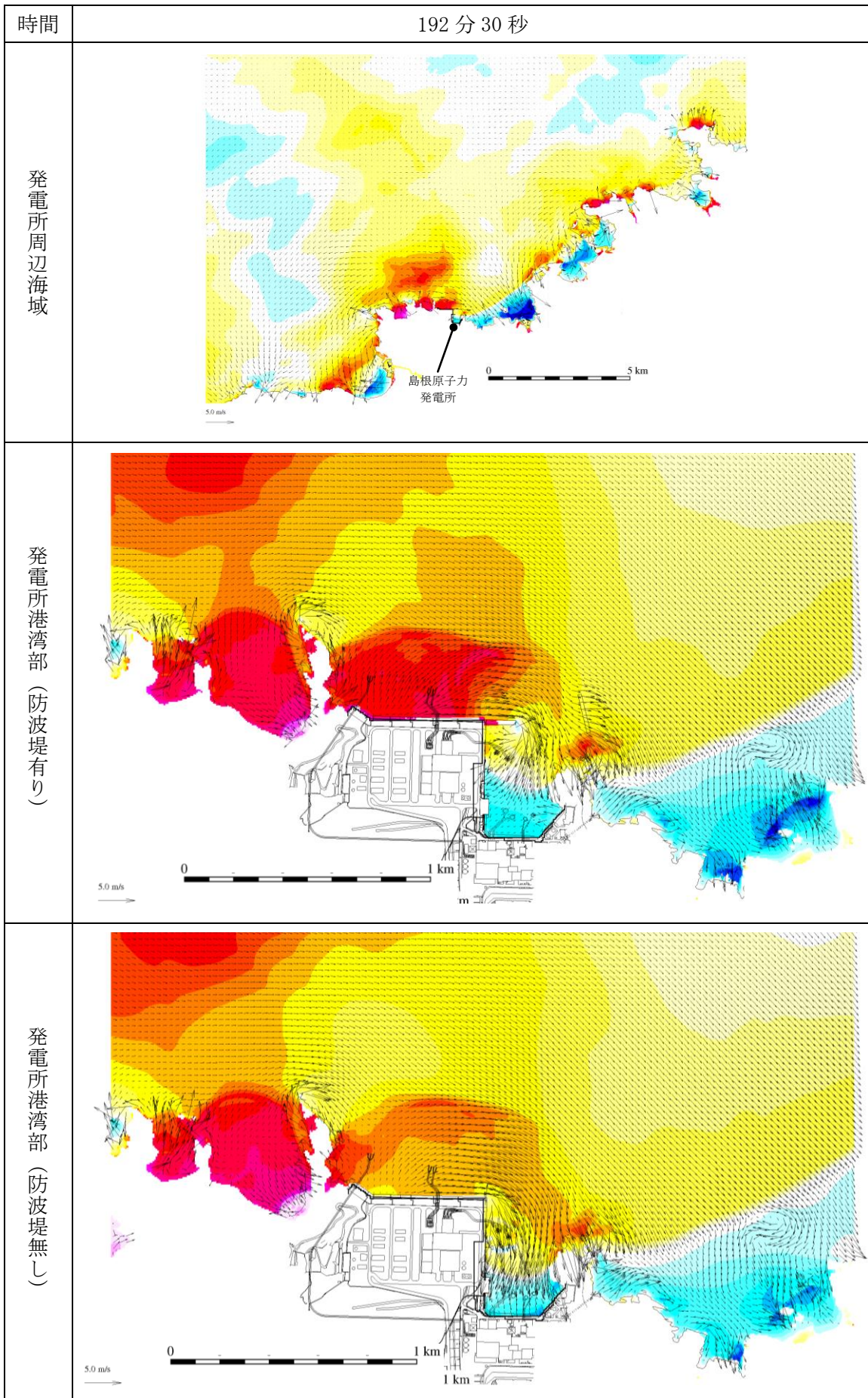
第 1 図(186) 基準津波 1 の水位変動・流向ベクトル
