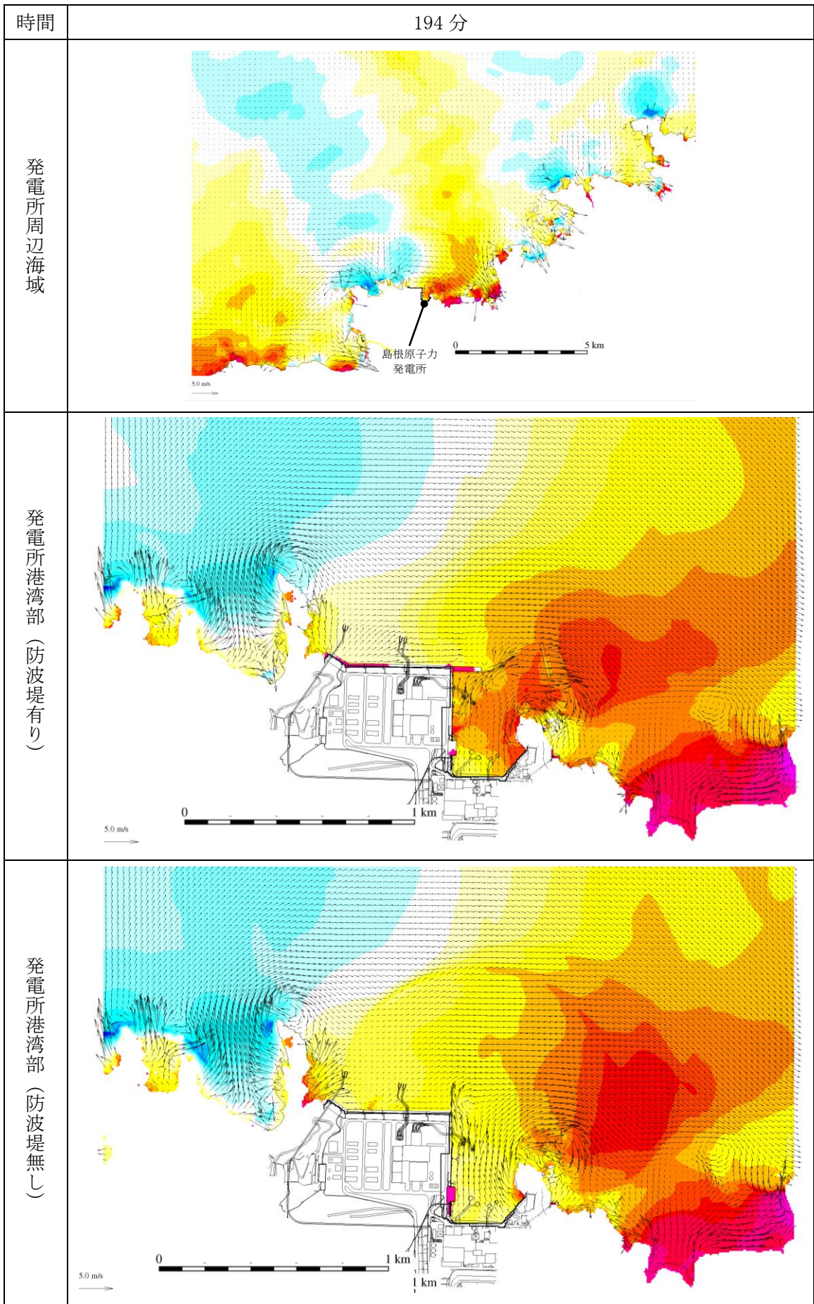
第 1 図(189) 基準津波 1 の水位変動・流向ベクトル
