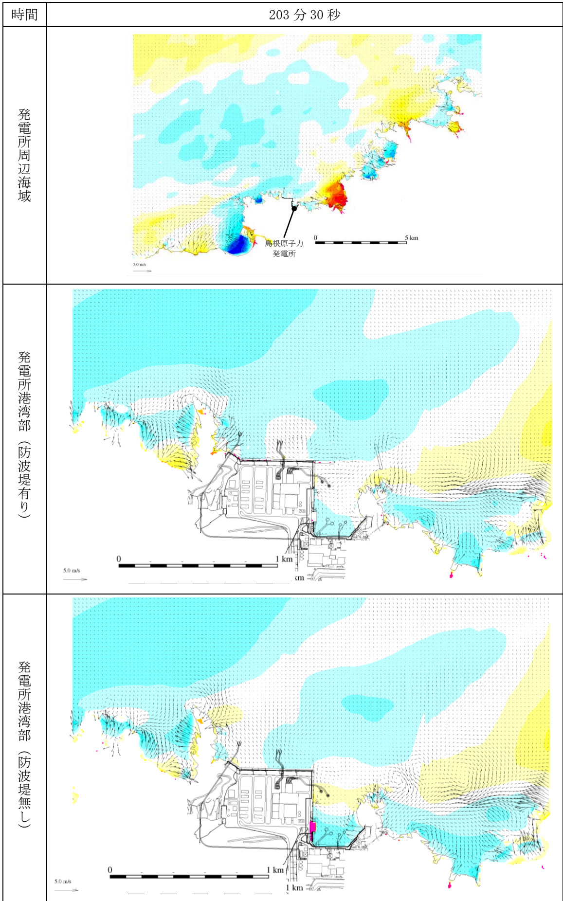
第 1 図 (208) 基準津波 1 の水位変動・流向ベクトル
