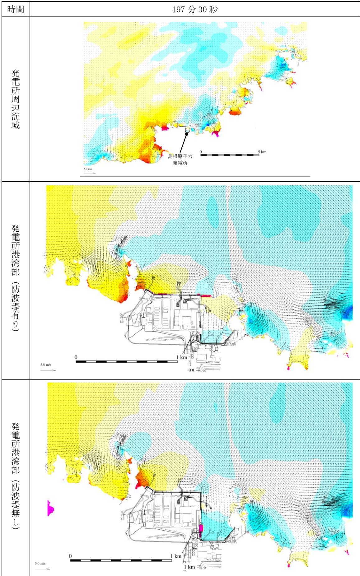
第 1 図(196) 基準津波 1 の水位変動・流向ベクトル
