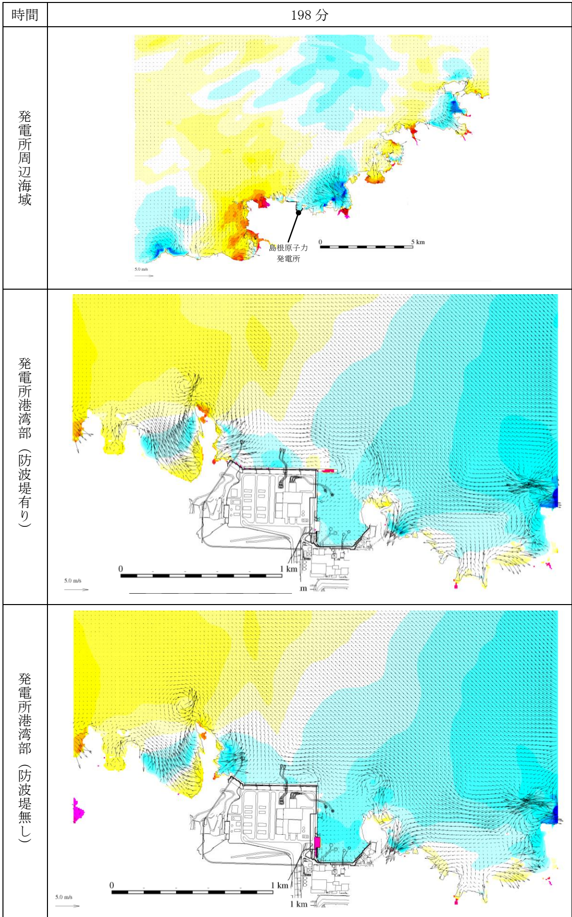
第 1 図(197) 基準津波 1 の水位変動・流向ベクトル
