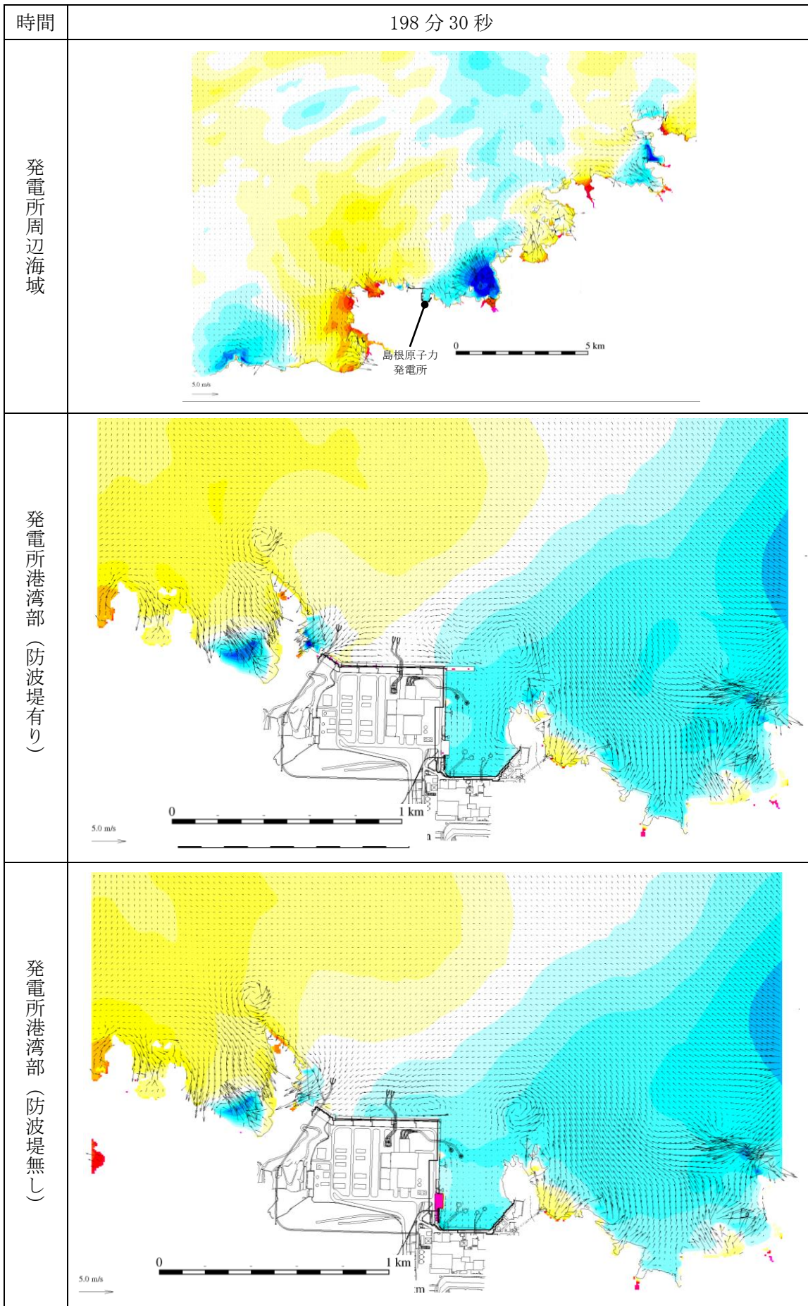
第 1 図(198) 基準津波 1 の水位変動・流向ベクトル
