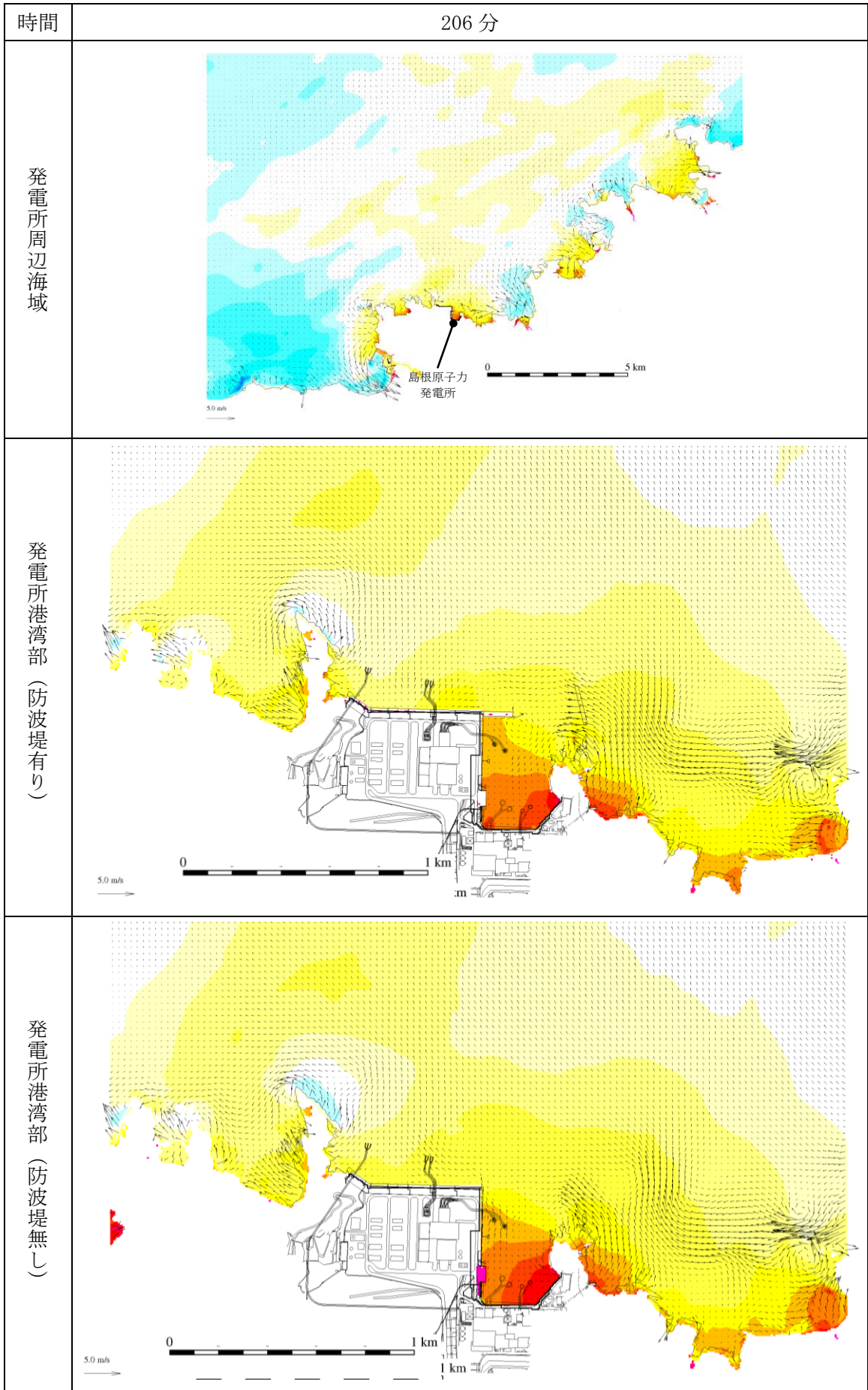
第 1 図 (213) 基準津波 1 の水位変動・流向ベクトル
