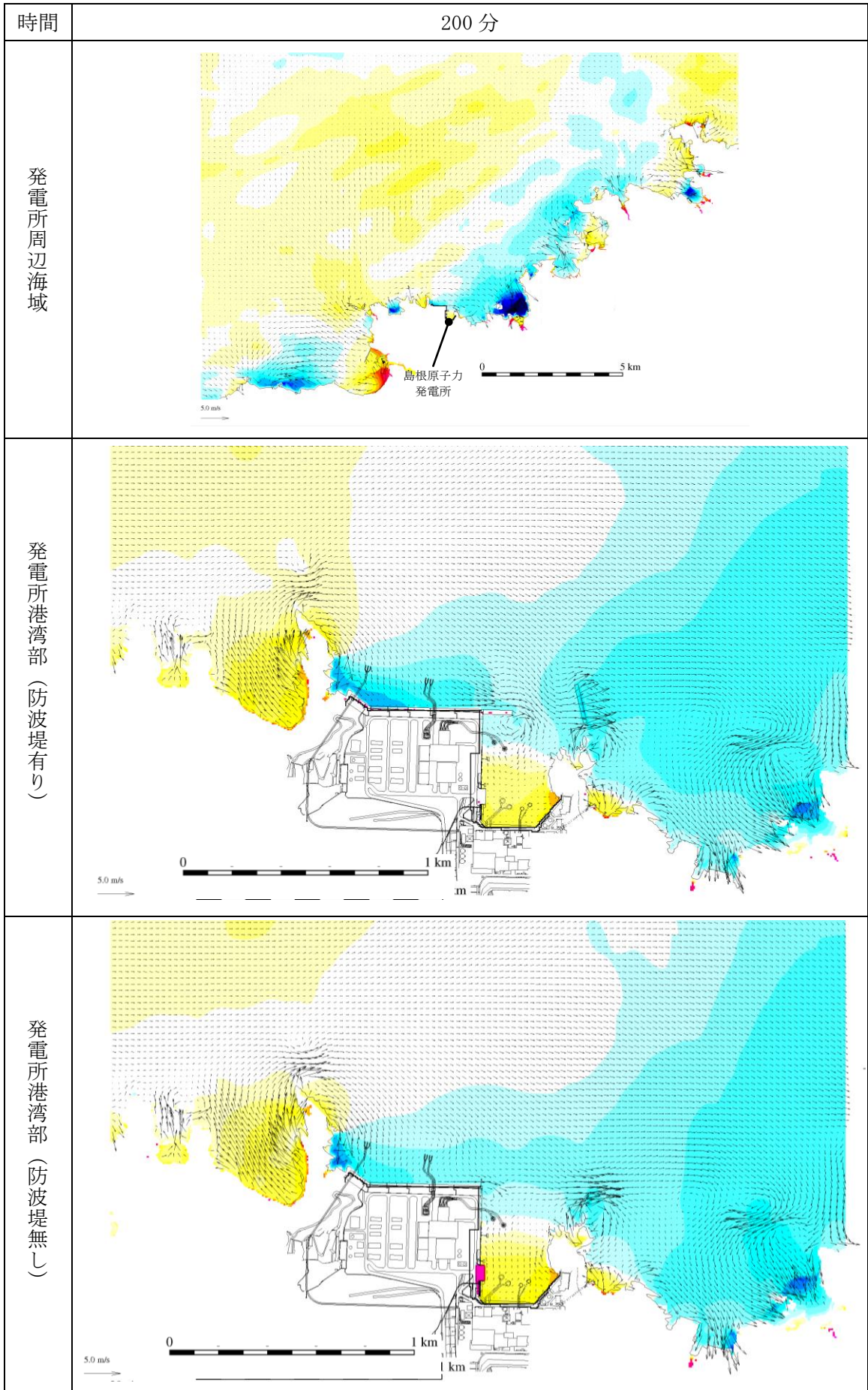
第 1 図 (201) 基準津波 1 の水位変動・流向ベクトル
