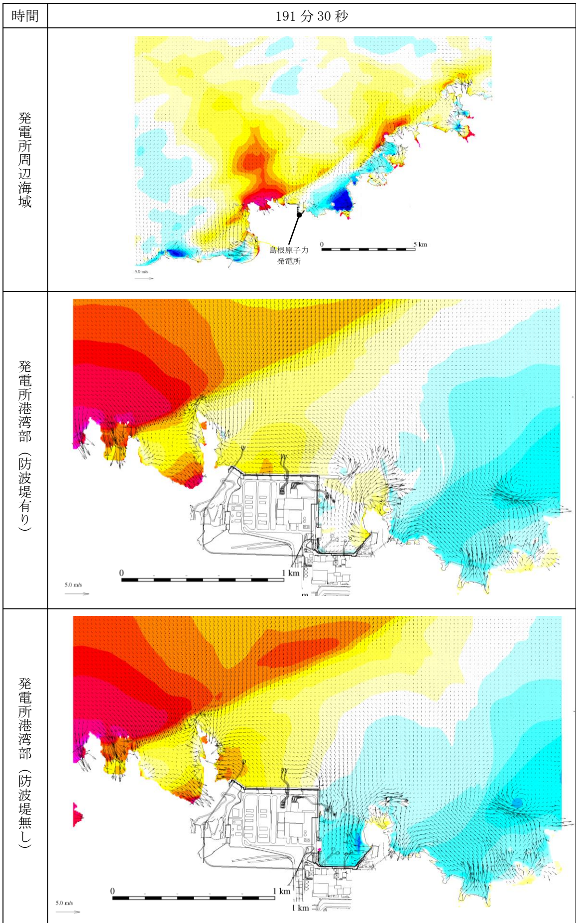
第 1 図(184) 基準津波 1 の水位変動・流向ベクトル
