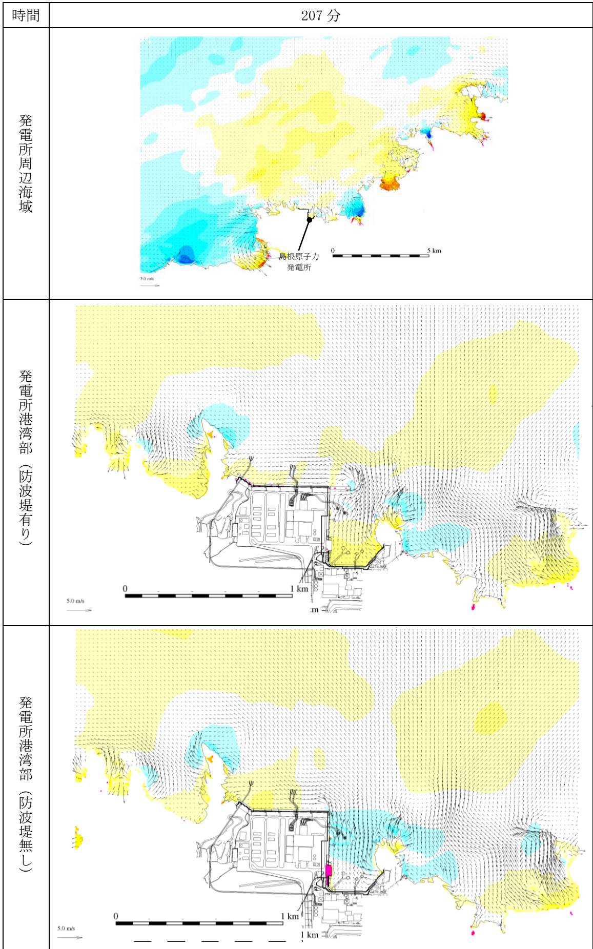
第 1 図 (215) 基準津波 1 の水位変動・流向ベクトル
