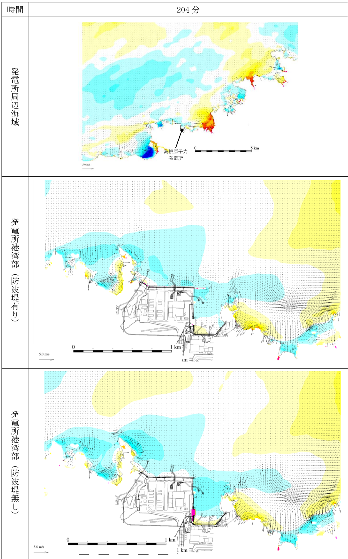
第 1 図 (209) 基準津波 1 の水位変動・流向ベクトル
