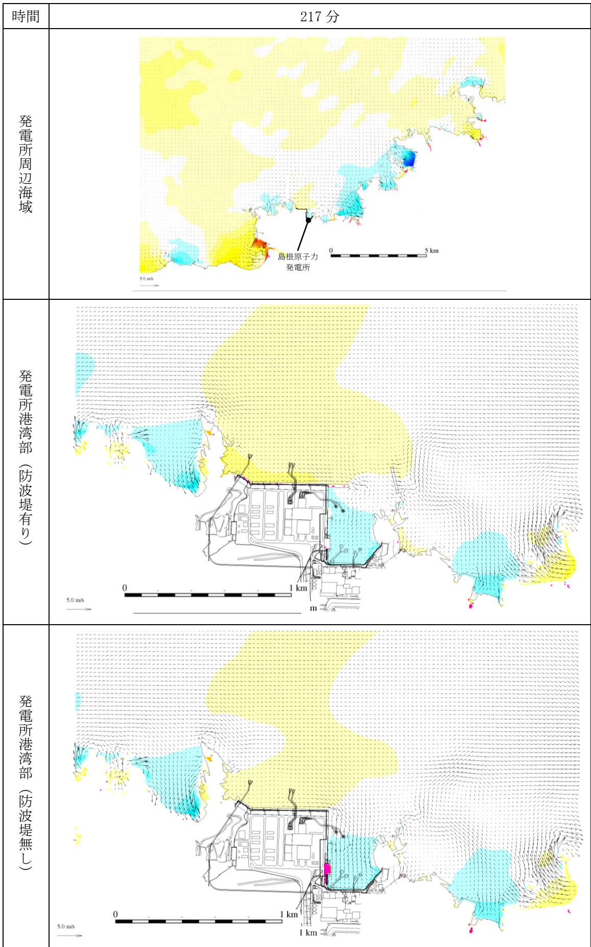
第 1 図 (235) 基準津波 1 の水位変動・流向ベクトル
