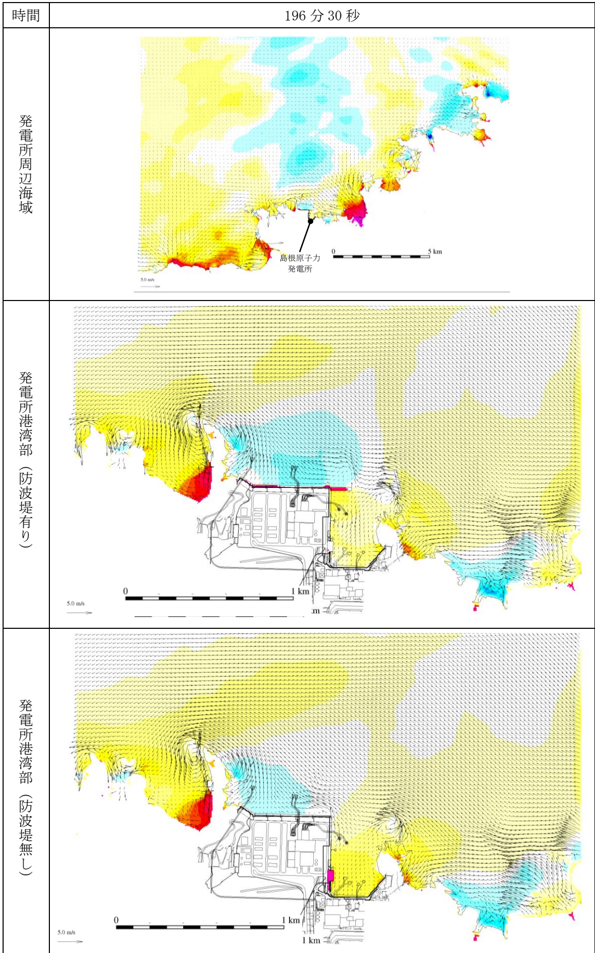
第 1 図(194) 基準津波 1 の水位変動・流向ベクトル
