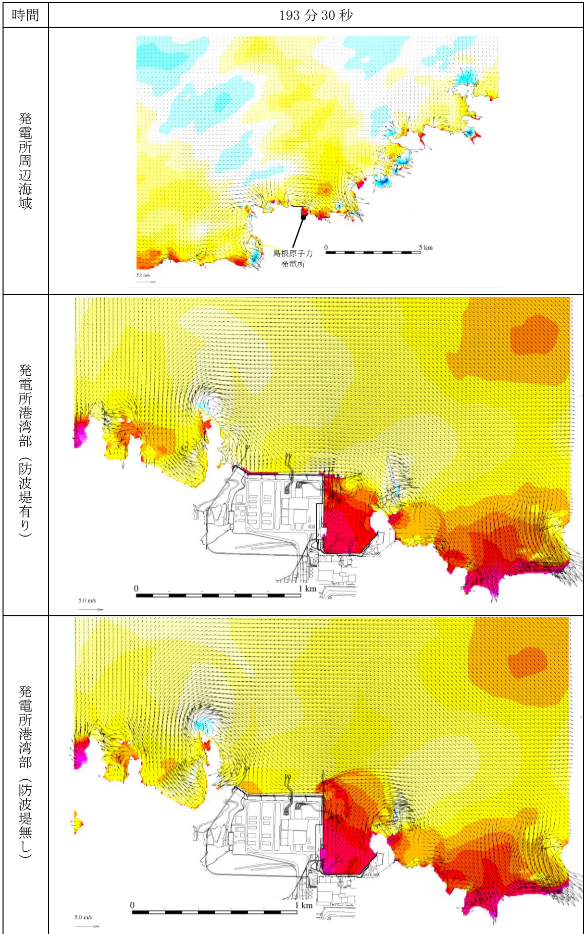
第 1 図(188) 基準津波 1 の水位変動・流向ベクトル
