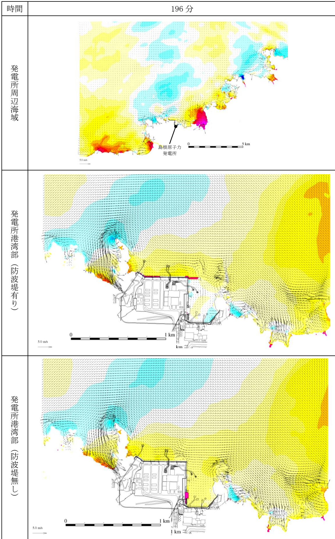
第 1 図(193) 基準津波 1 の水位変動・流向ベクトル
