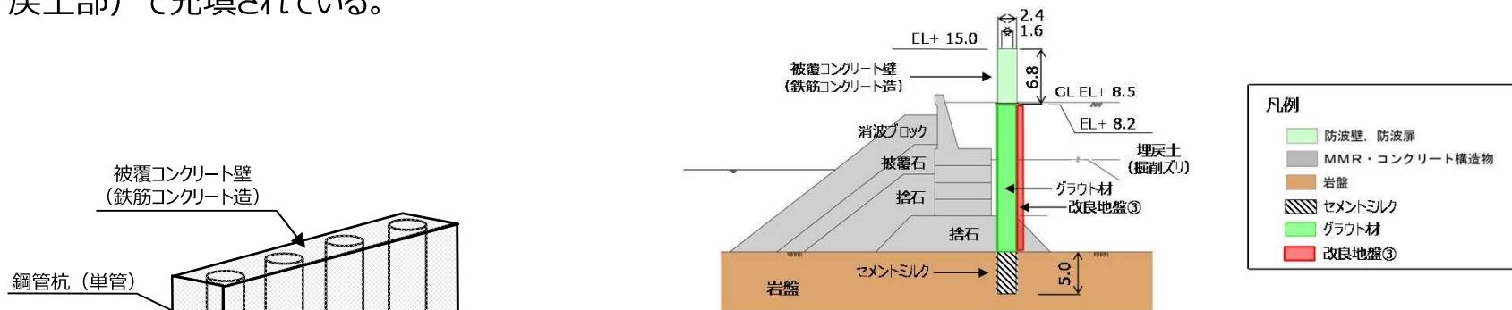
防波壁(多重鋼管杭式擁壁) 杭間部 断面図
