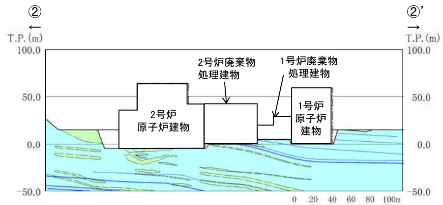
②-②' 断面図
