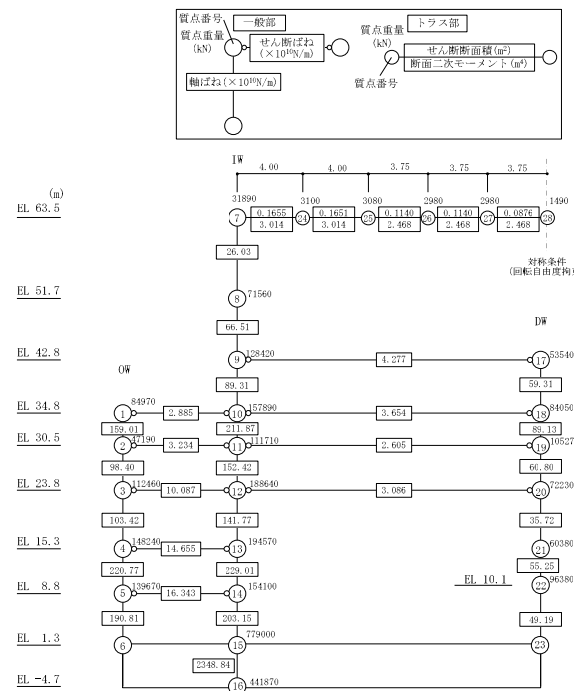
鉛直モデル
