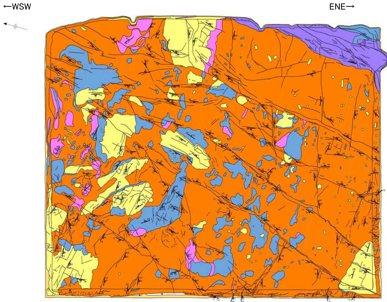
底面スケッチ図(岩相区分)
