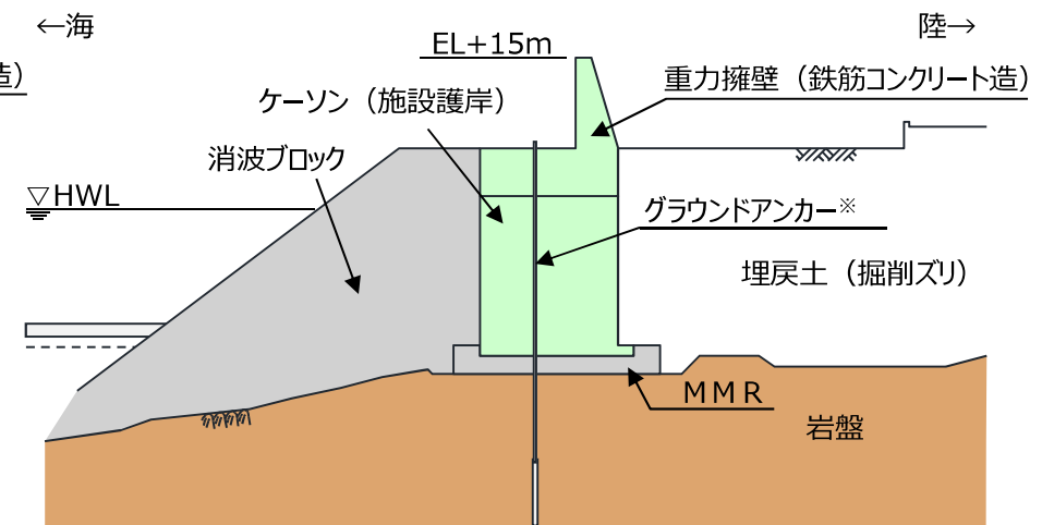
※ グラウンドアンカーの効果を期待しなくても、耐震・耐津波安全性を担保している。 防波壁（波返重力擁壁）（岩盤部）断面図
