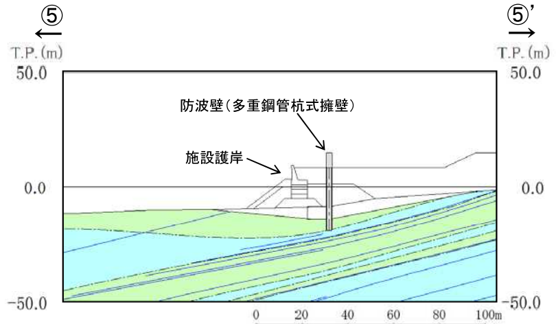
⑤-⑤' 断面図
