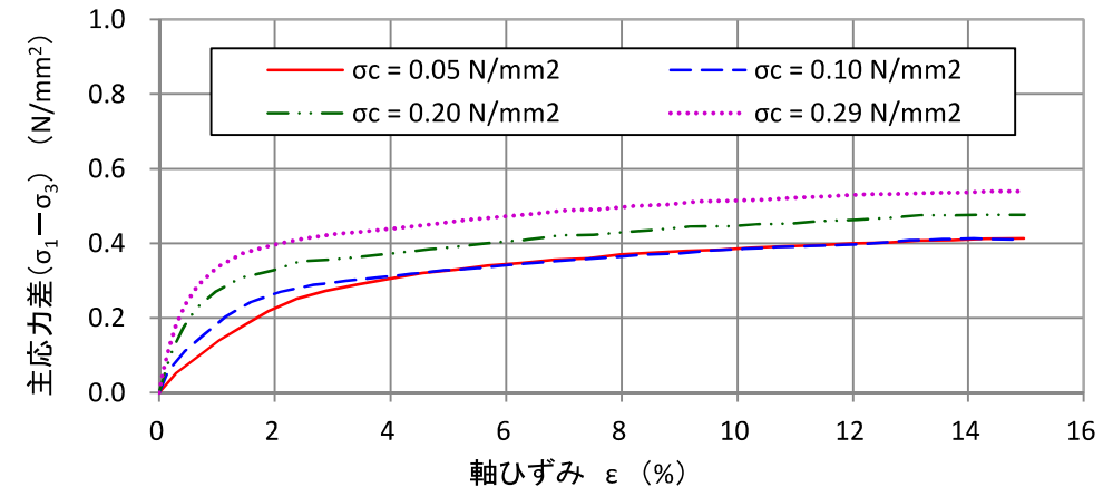
大型三軸圧縮試験結果(応力-ひずみ関係)
