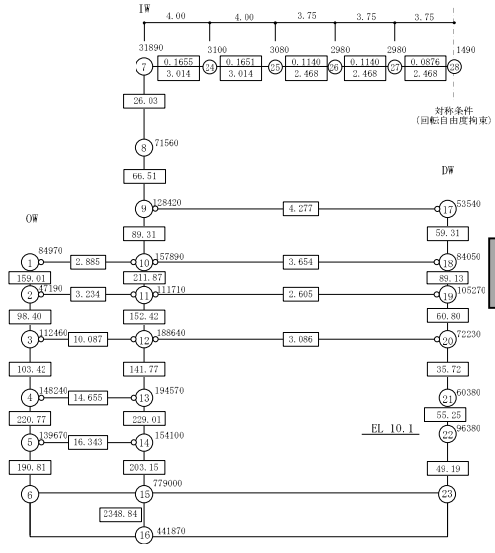
鉛直モデル
