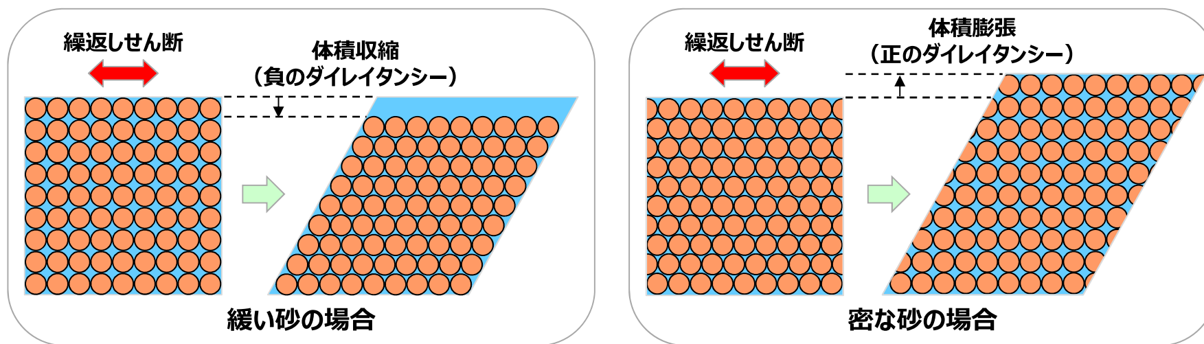
地盤のダイレイタンスー特性の概要
