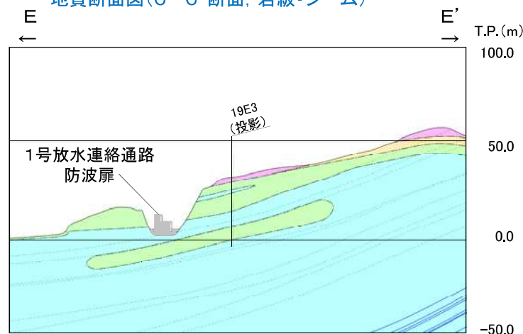
地質断面図(E-E'断面, 岩級・シーム)
