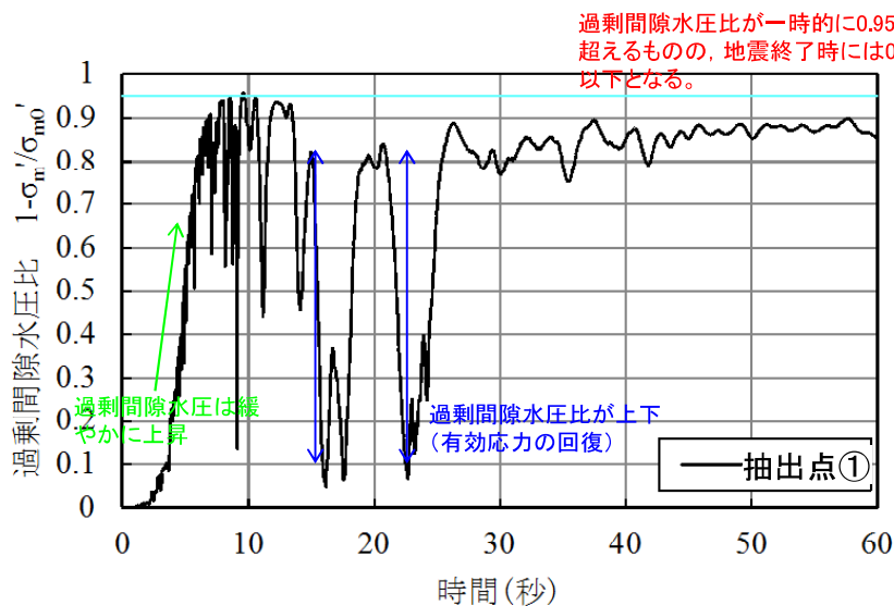
過剰間隙水圧比(抽出点①)
