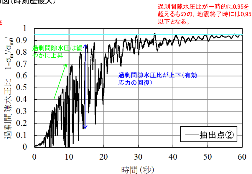
過剰間隙水圧比(抽出点②)
