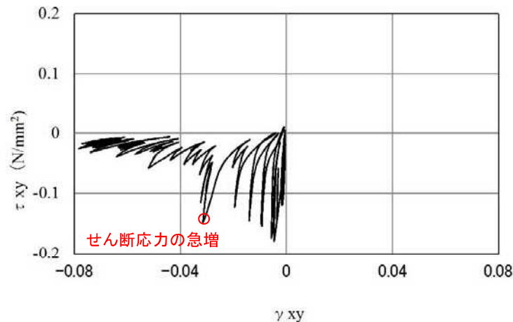
せん断応力～せん断ひずみ(抽出点②)
