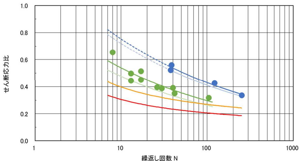
液状化強度曲線の比較
