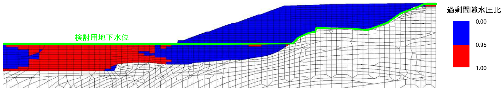
過剰間隙水圧比分布図(時刻歴最大)
