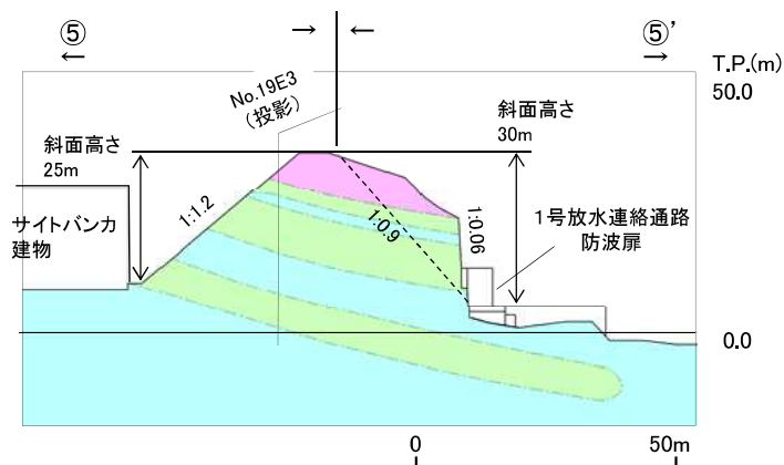
1号放水連絡通路防波扉等周辺斜面(⑤-⑤'断面, 岩級・シーム)
