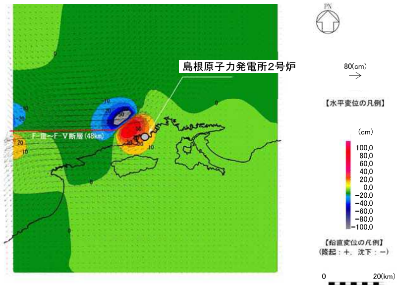
地殻変動解析結果(F-Ⅲ~F-V断層 上昇最大ケース)
