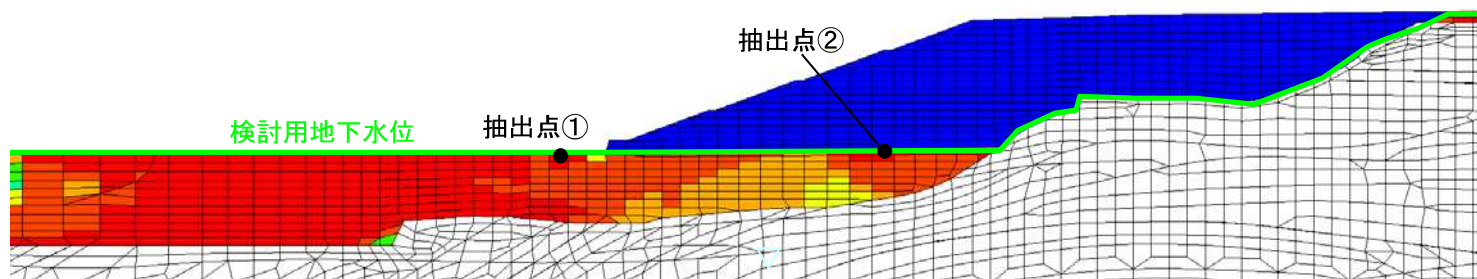
過剰間隙水圧比分布図(時刻歴最大)
