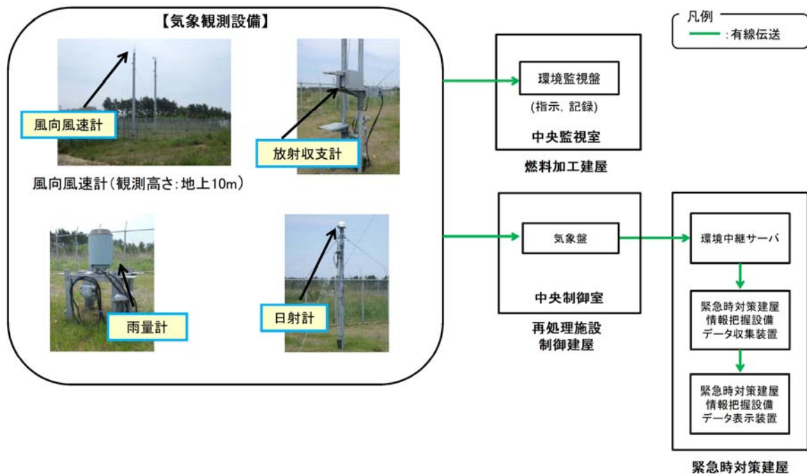
第 6 図 気象観測設備の外観及び伝送概略図
