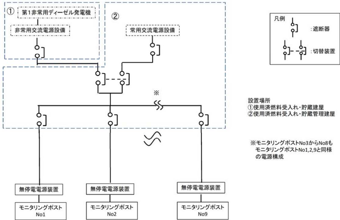
第 11. 1 . 1 図 電源構成概略図
