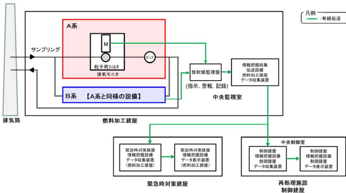
第1図 排気モニタの系統概要図
