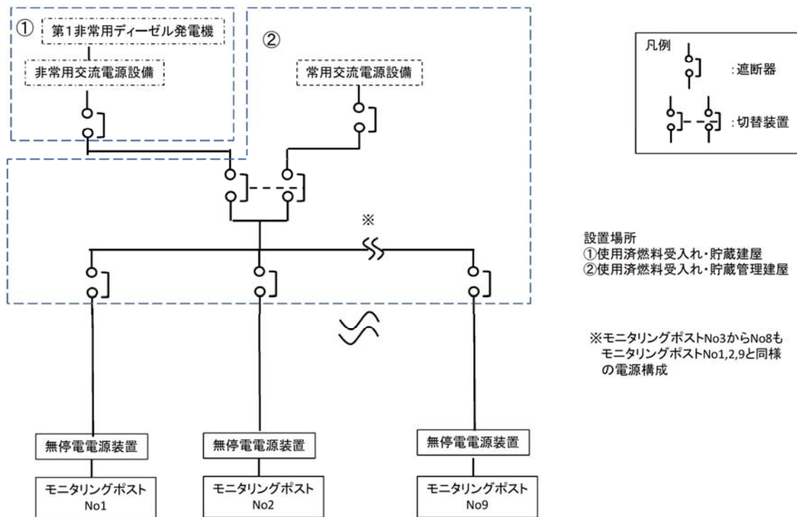
第3図 モニタリングポスト等の電源構成概略図
