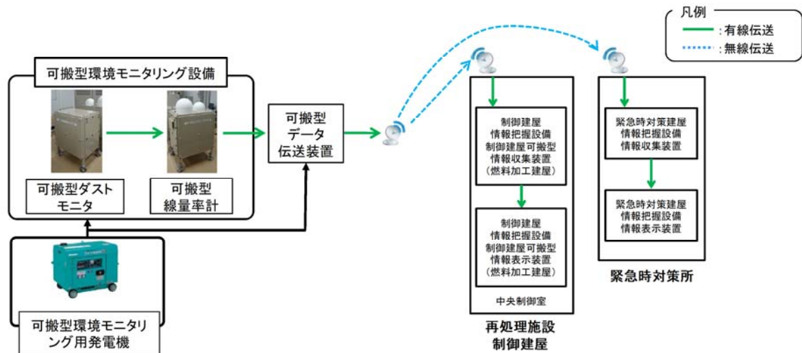
第 4 . 1 . 2 図 可搬型環境モニタリング設備の伝送概略図
