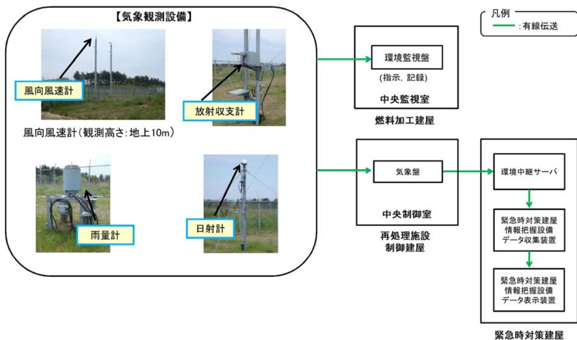
第9. 1. 1図 気象観測設備の外観及び伝送概略図
