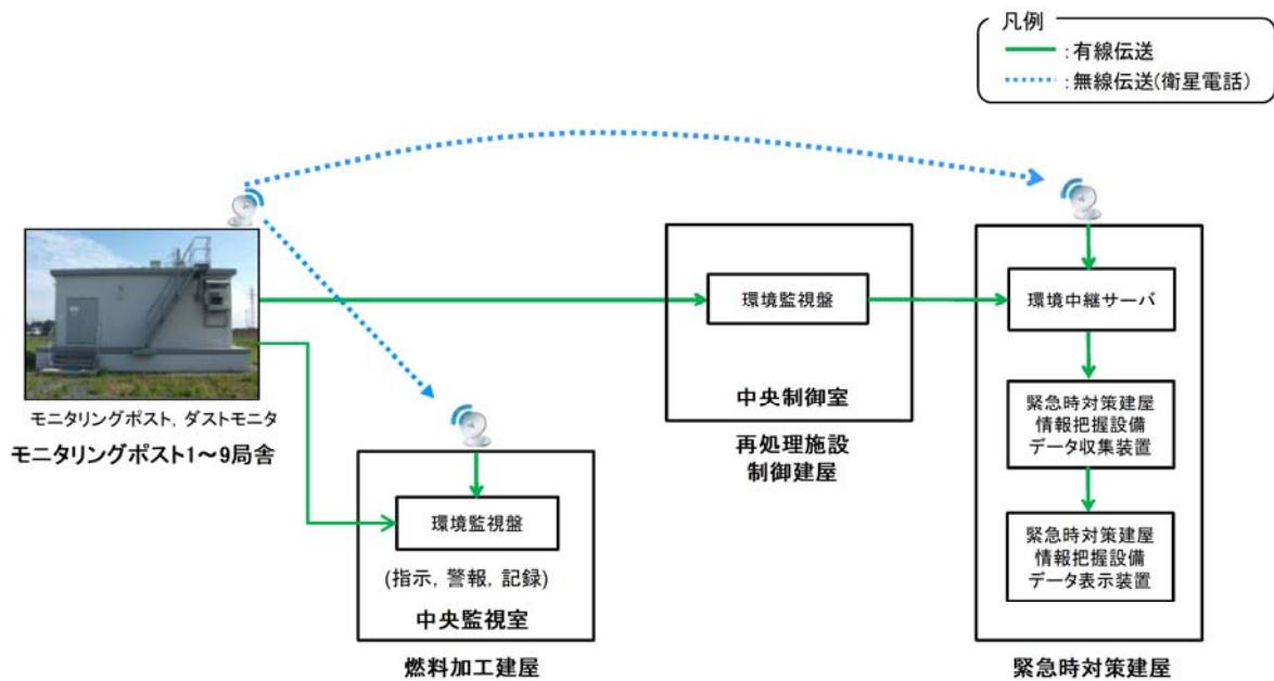
第4図 モニタリングポスト等の系統概略図
