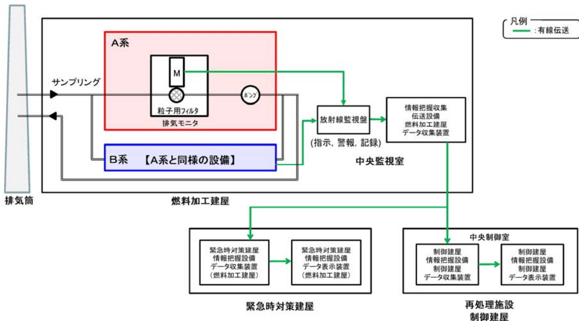
第1. 1. 1図 排気モニタの系統概要図
