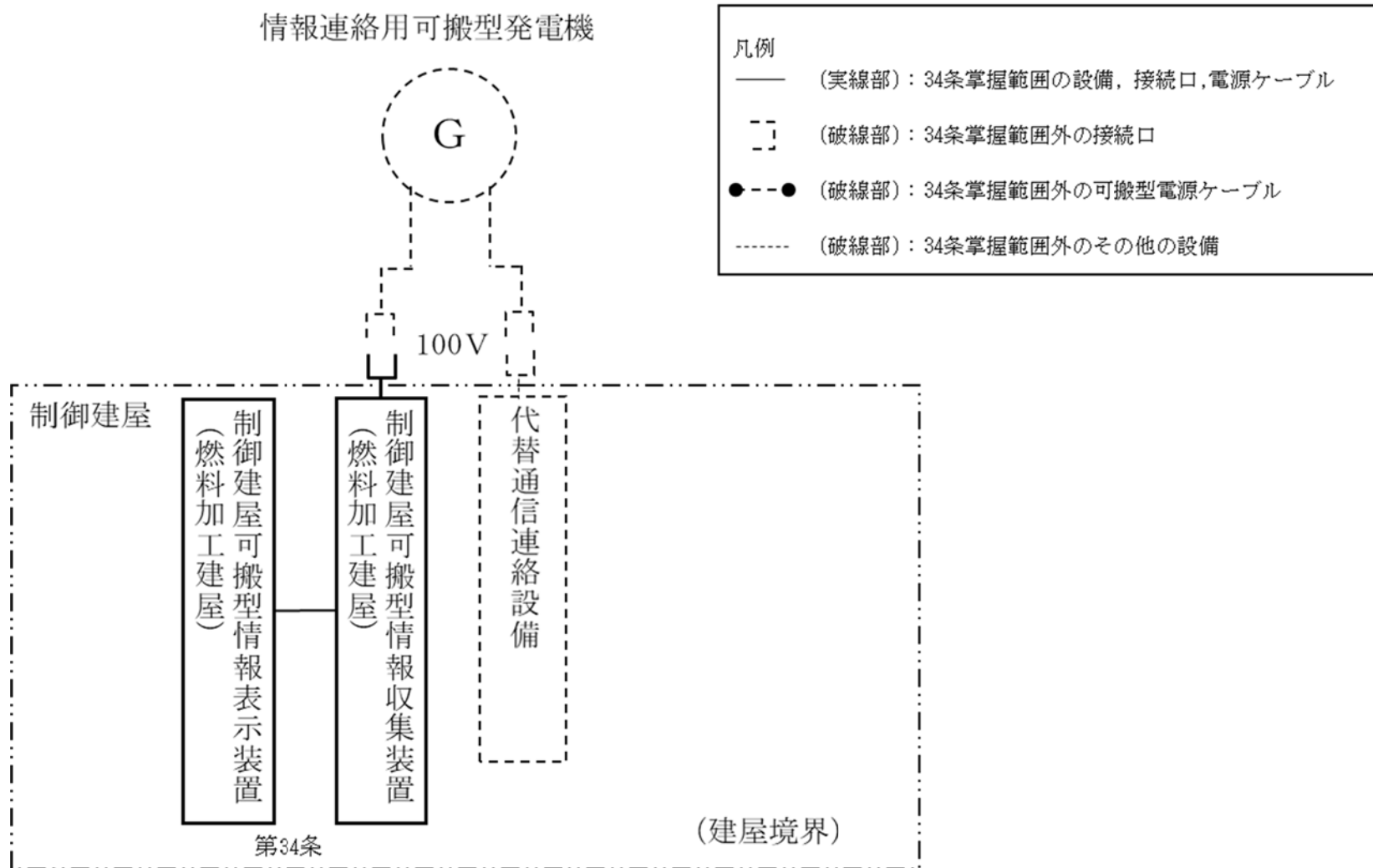
第 34. 7 図 情報把握設備 電源供給系統図 (2 / 5)
