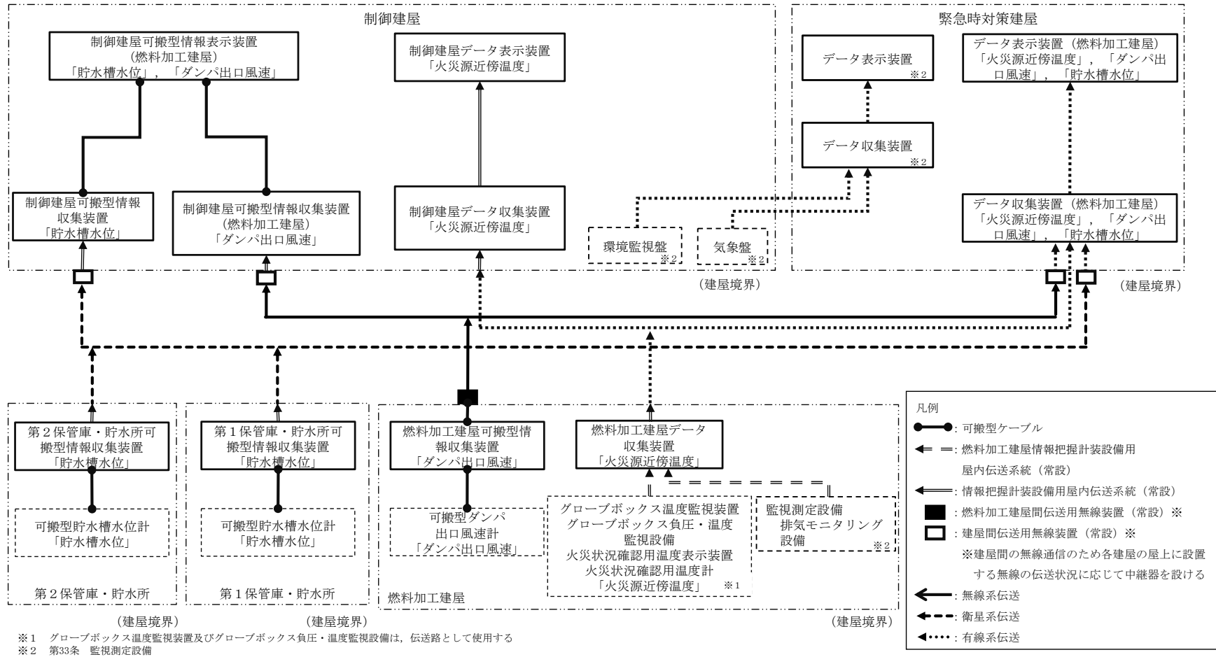
第 34. 4 図 情報把握設備 全体系統概要図 (2 / 2)
