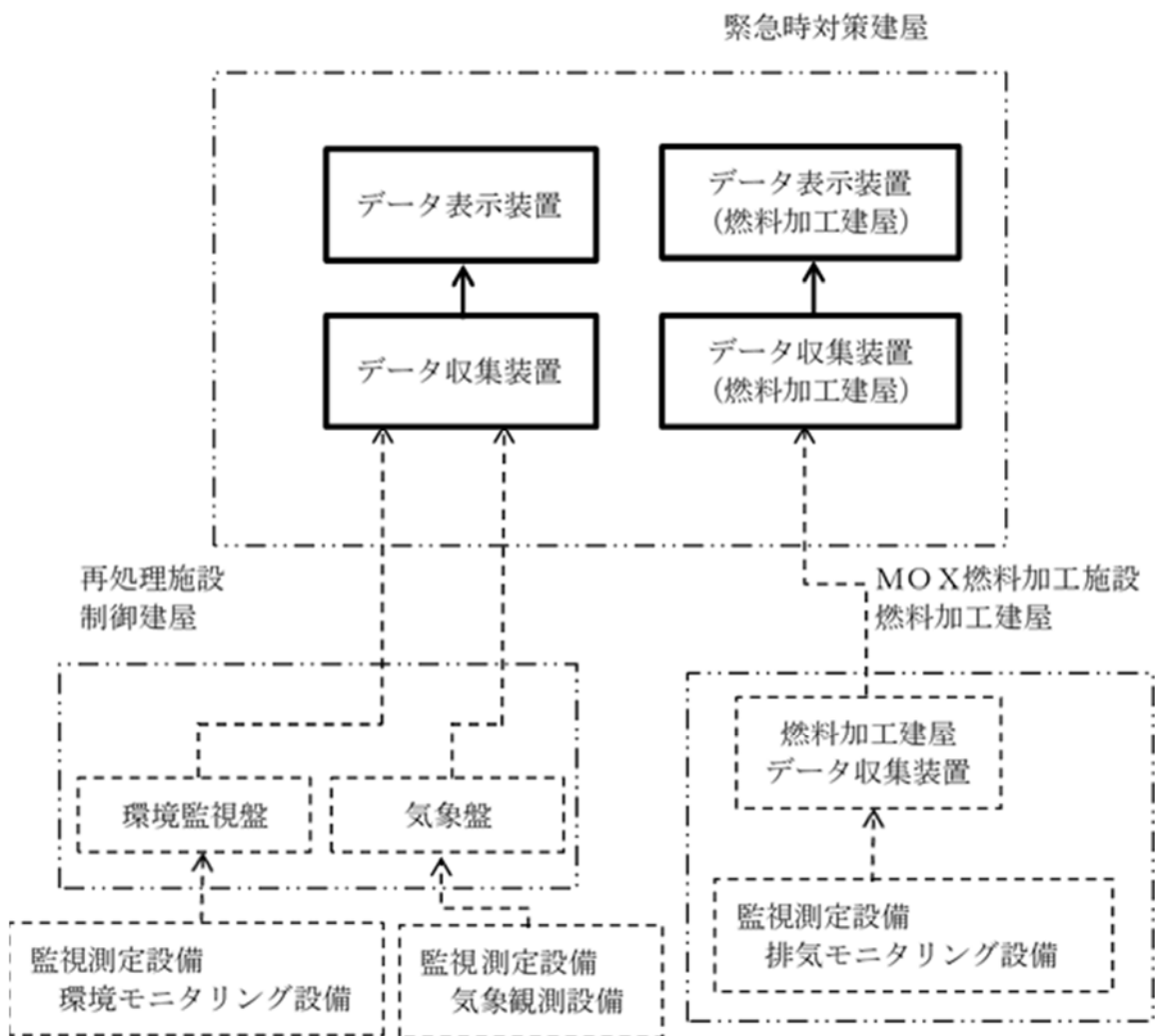
第 34. 6 図 情報把握設備 系統概要図 (第 33 条 監視測定設備関係 全交流動力電源の喪失を伴わない安全機能の喪失) (2 / 2)
