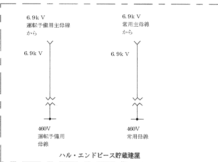
第5. 2. 7-2. 2-2 (4) 図 主要建物内単線結線図
