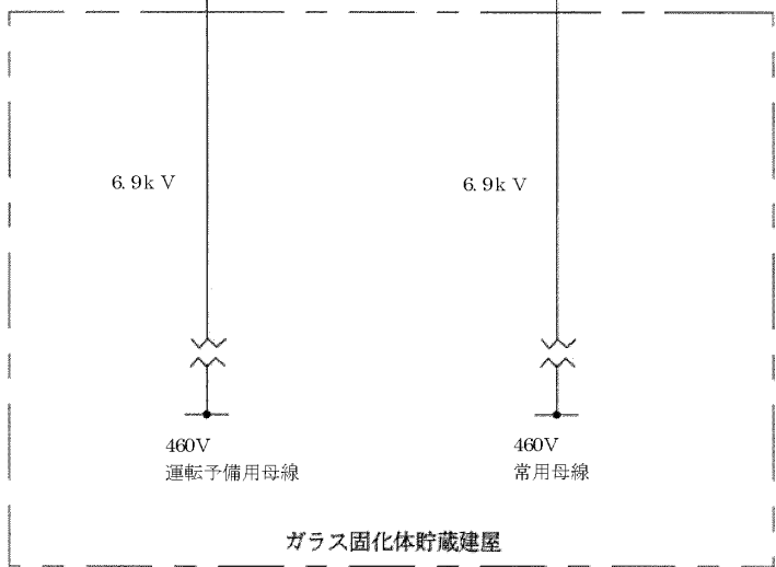
第5. 2. 7-2. 2-2 (4) 図 主要建物内単線結線図
