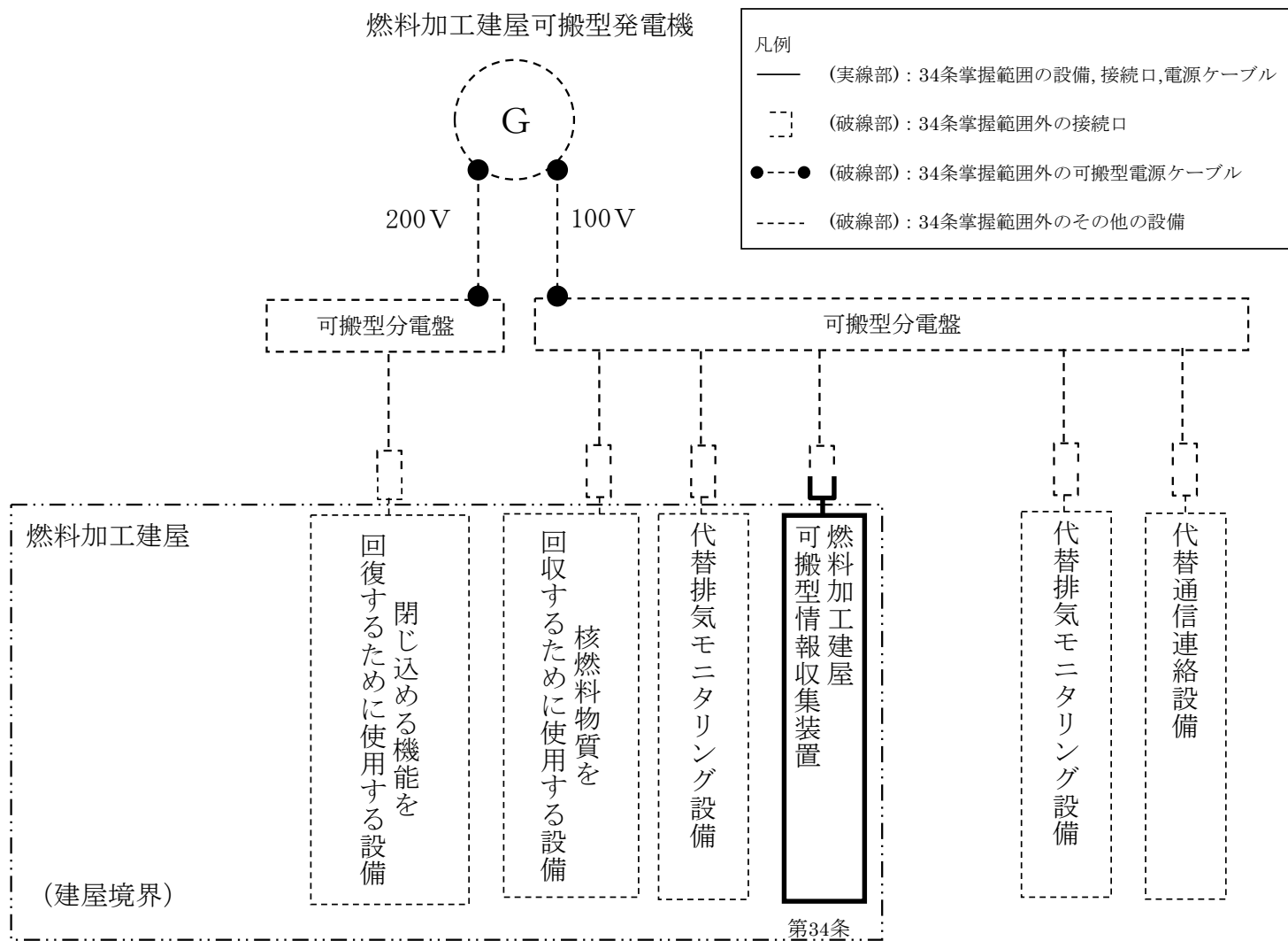
第 34. 6 図 情報把握設備 電源供給系統図 ( 1 / 5 )
