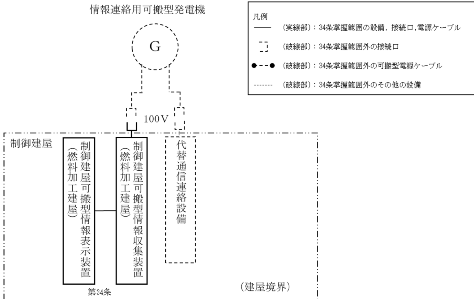
第 34. 6 図 情報把握設備 電源供給系統図 ( 2 / 5 )
