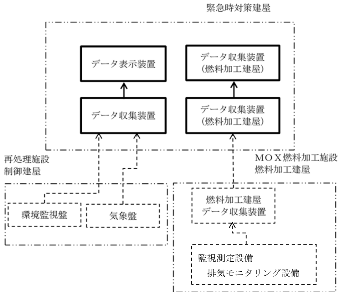
第 34. 5 図 情報把握設備 系統概要図 (第 33 条 監視測定設備関係 全交流動力電源の喪失を伴わない安全機能の喪失) (2 / 2)
