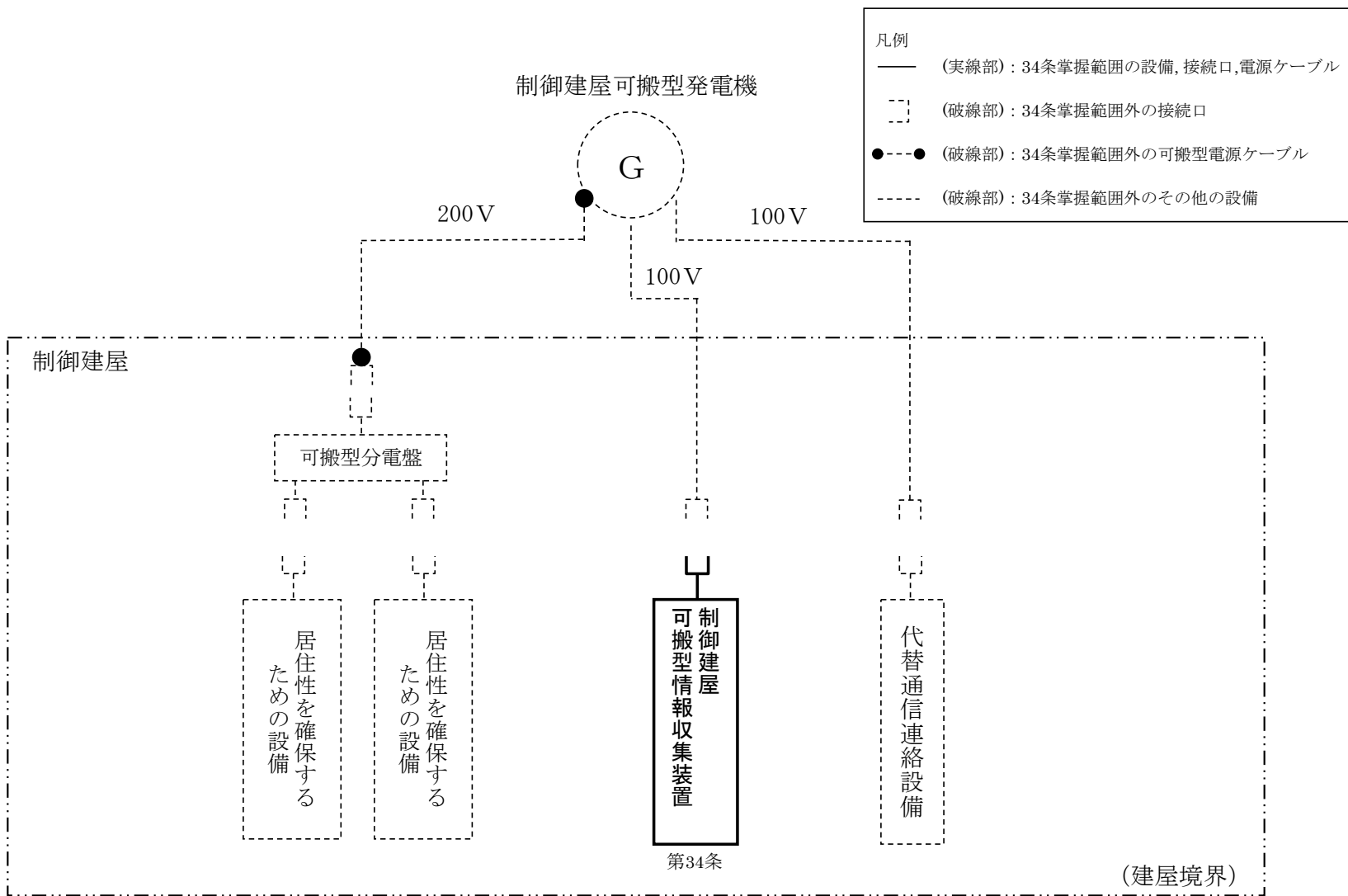
第 34. 6 図 情報把握設備 電源供給系統図 ( 3 / 5 )
