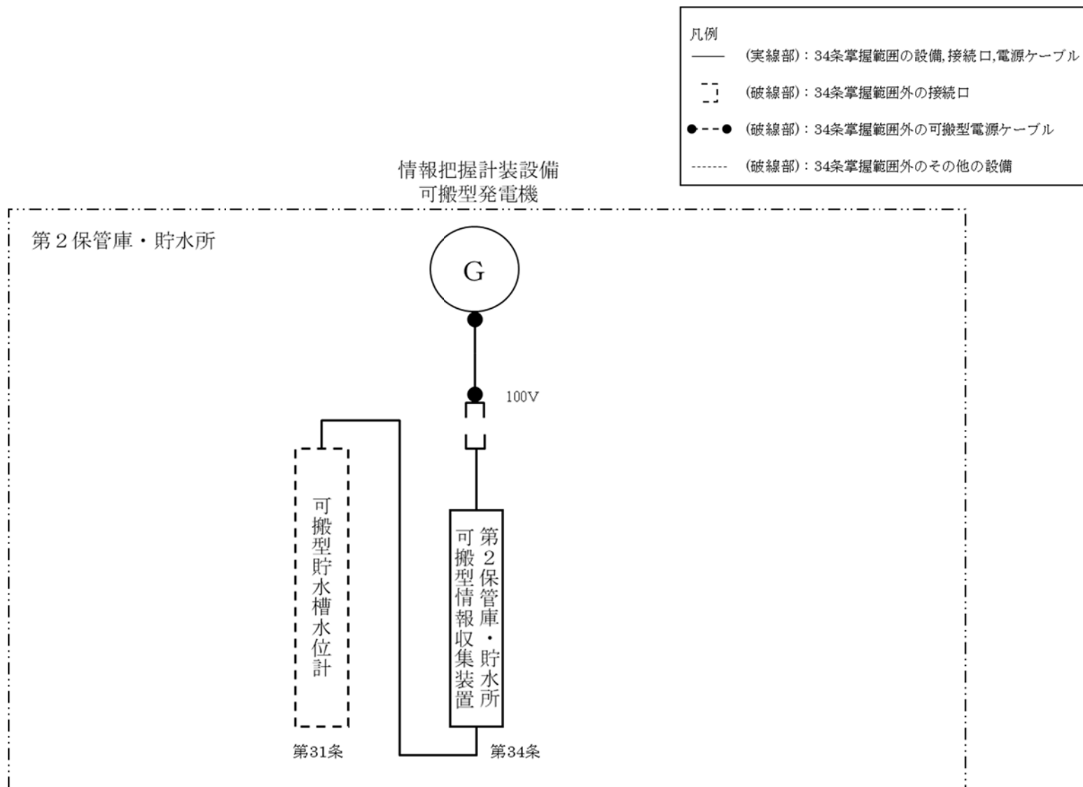
第 34. 6 図 情報把握設備 電源供給系統図 ( 5 / 5 )
