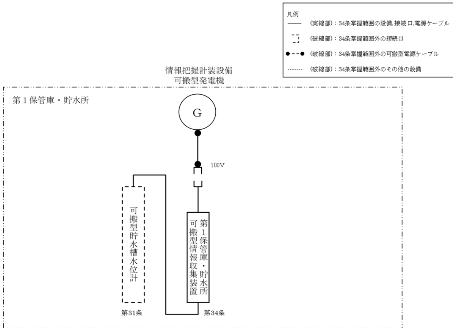
第 34. 6 図 情報把握設備 電源供給系統図 ( 4 / 5 )
