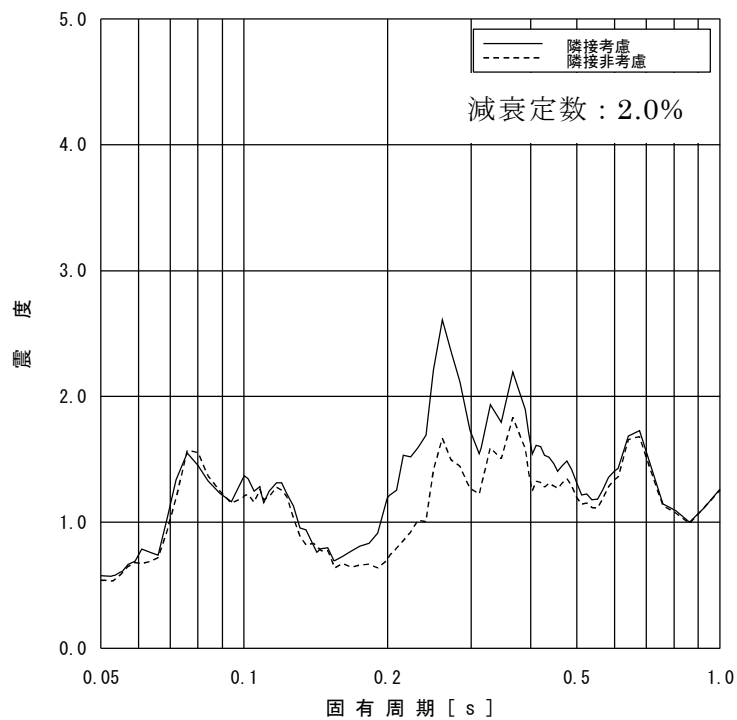
図添 5-1 (17/21) 床応答スペクトル (水平方向, T. M. S. L. 15.266m)
