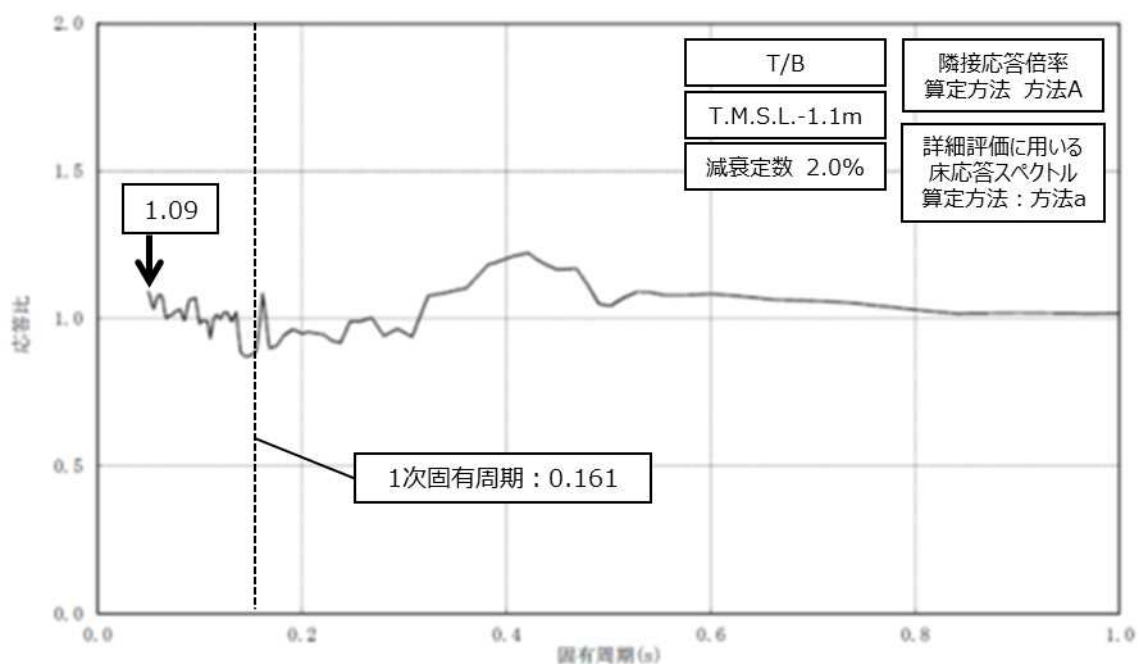
図添2-9 隣接応答倍率の算定 (RCW-T-5)
