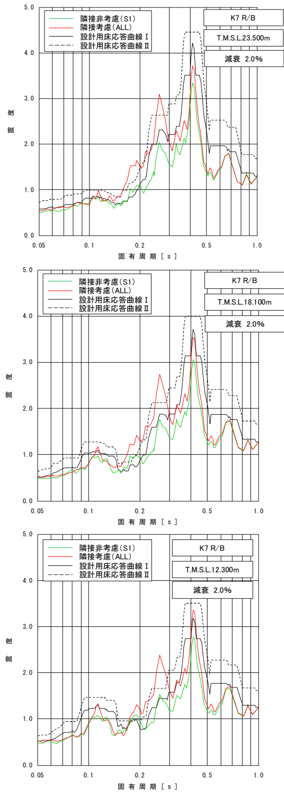
図添 1-1 床応答スペクトルの比較 (7号機原子炉建屋, 水平方向, 減衰 2.0%) (2/3)
