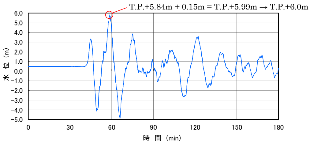
第 1.4.1 図(2) 入力津波波形 (2)
