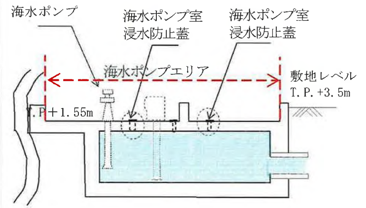
A-A断面図
