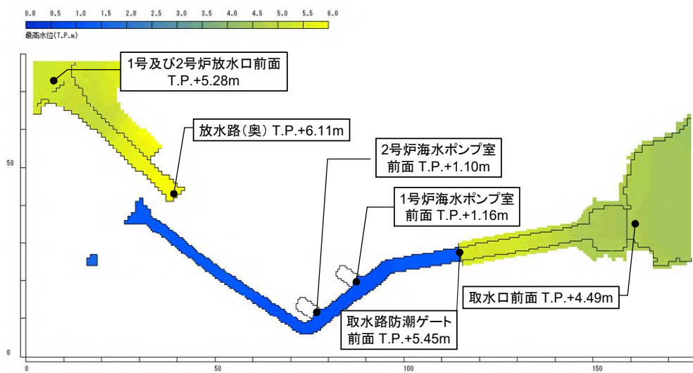
第 1.4.2 図(1) 基準津波 1 による最高水位分布
