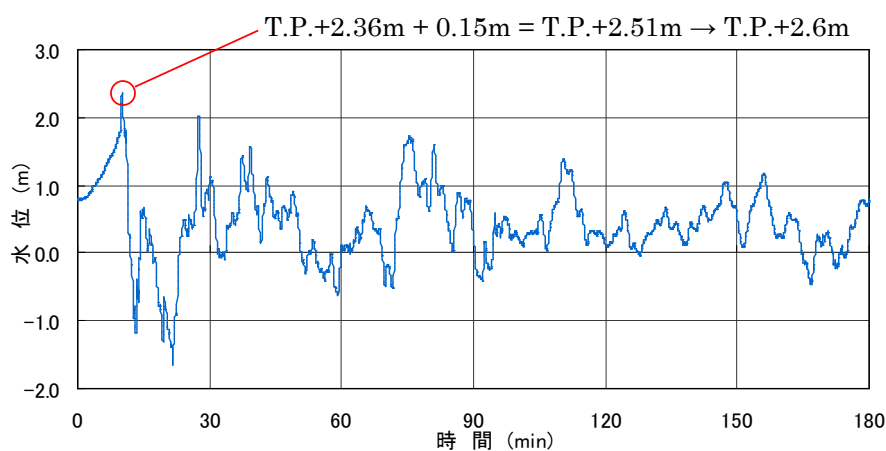
第 1.4.1 図(1) 入力津波波形(1)
