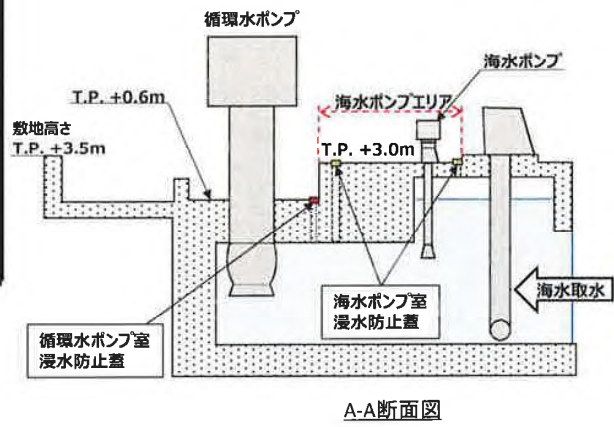
第 1.4.5 図(1) 1号炉海水ポンプ室周辺エリア浸水防止設備の概要
