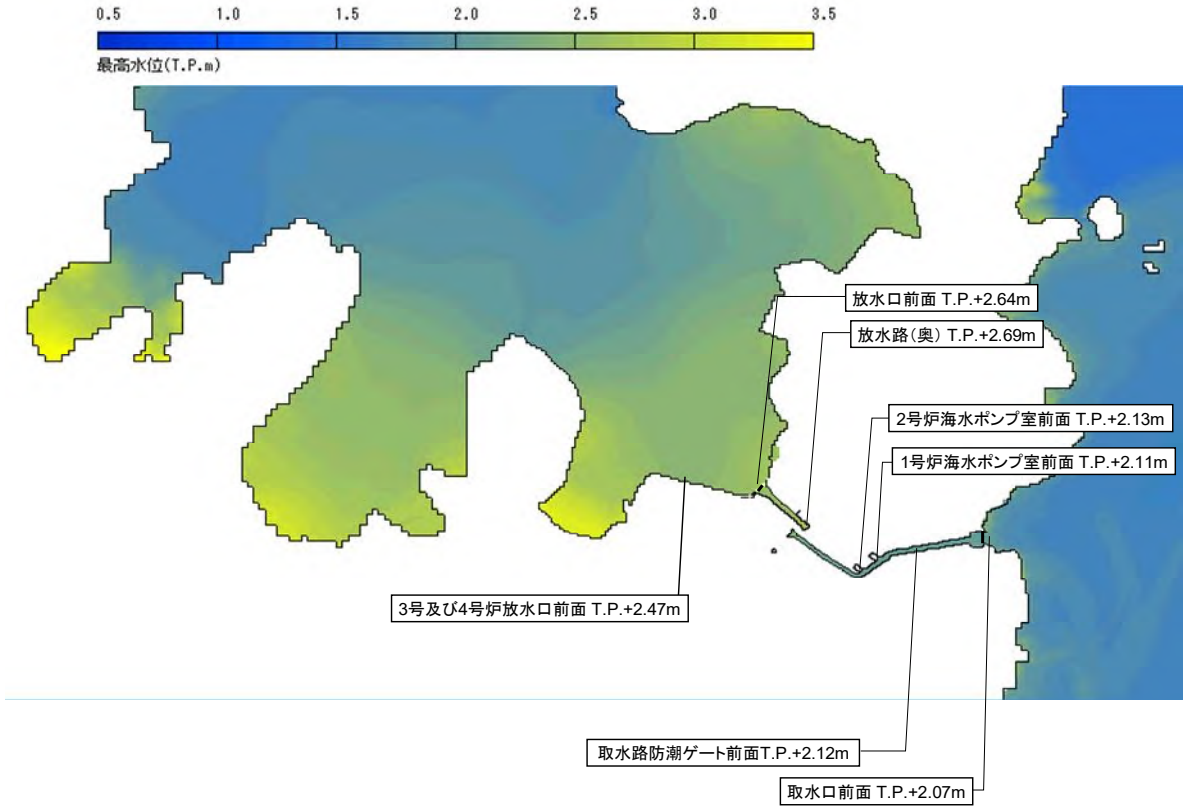
第 1.4.2 図(2) 基準津波 2 による最高水位分布
