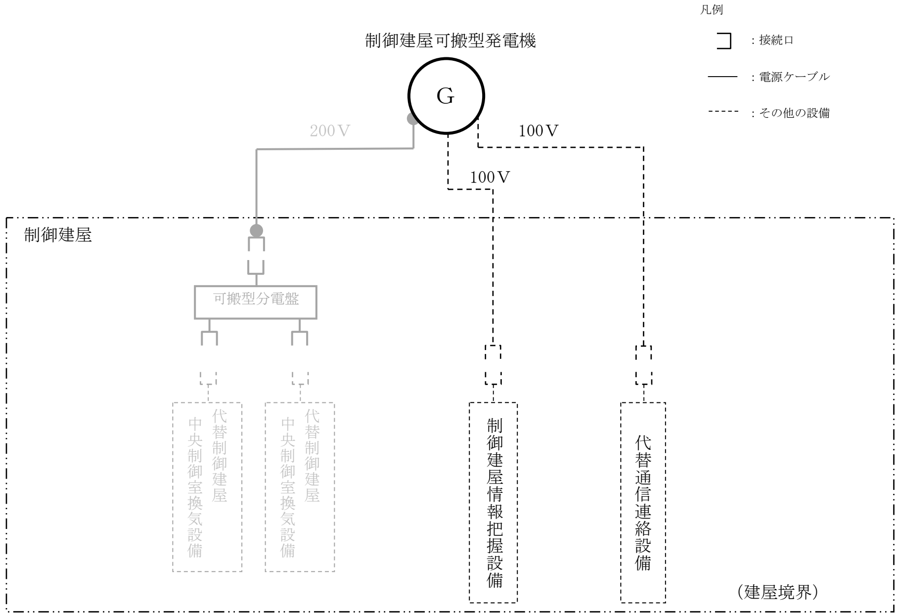
第 32. 3 図 全交流電源喪失時において重大事故等に対処するための電力を確保するための設備の系統図 (再処理施設の制御建屋可搬型発電機)
