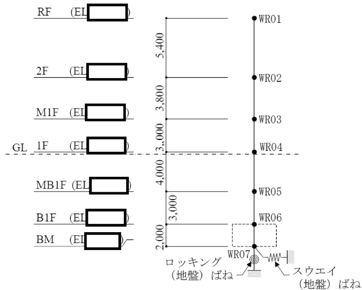
第2-2図 廃樹脂処理建屋の解析モデル図
