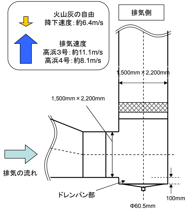
図1 格納容器排気筒曲がり部の構造（高浜3号機）
