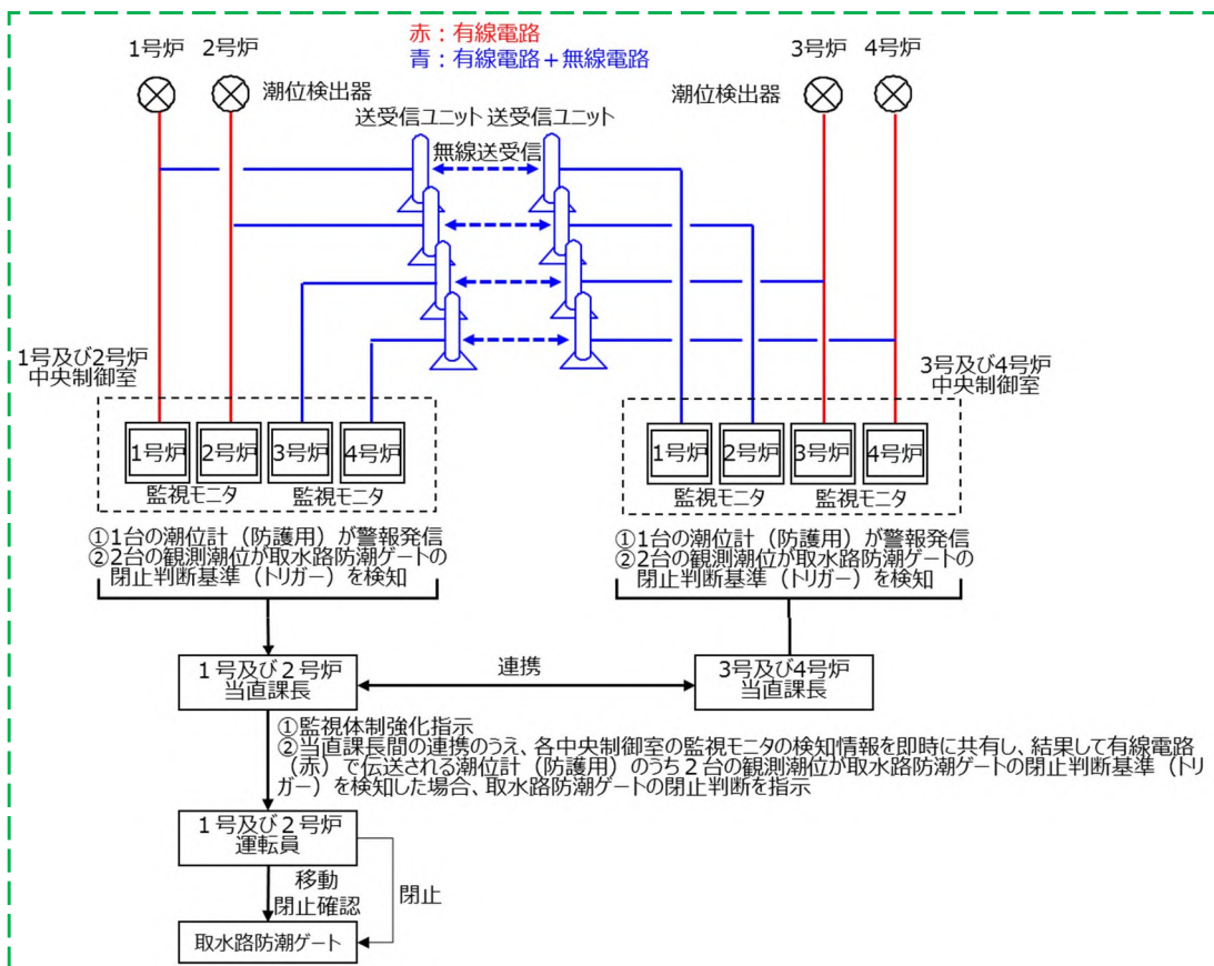
図3 取水路防潮ゲートの閉止判断基準（トリガー）を検知するための一連の設備
