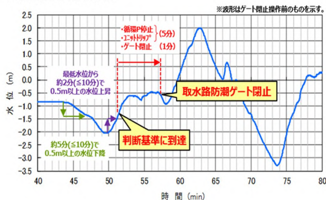
図 1 取水路防潮ゲートの閉止判断基準（トリガー）の一例
