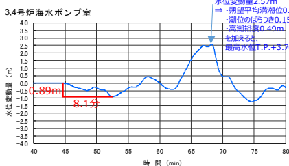
図 1 5 崩壊規模のパラメータスタディ結果 (津波検知の判断基準 (トリガー) による検知可否の確認)
