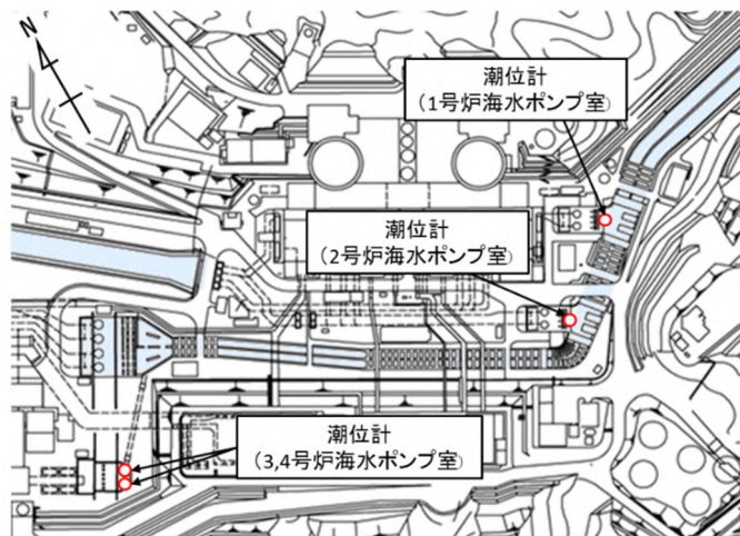
図 3 3 潮位計(防護用)の設置位置
