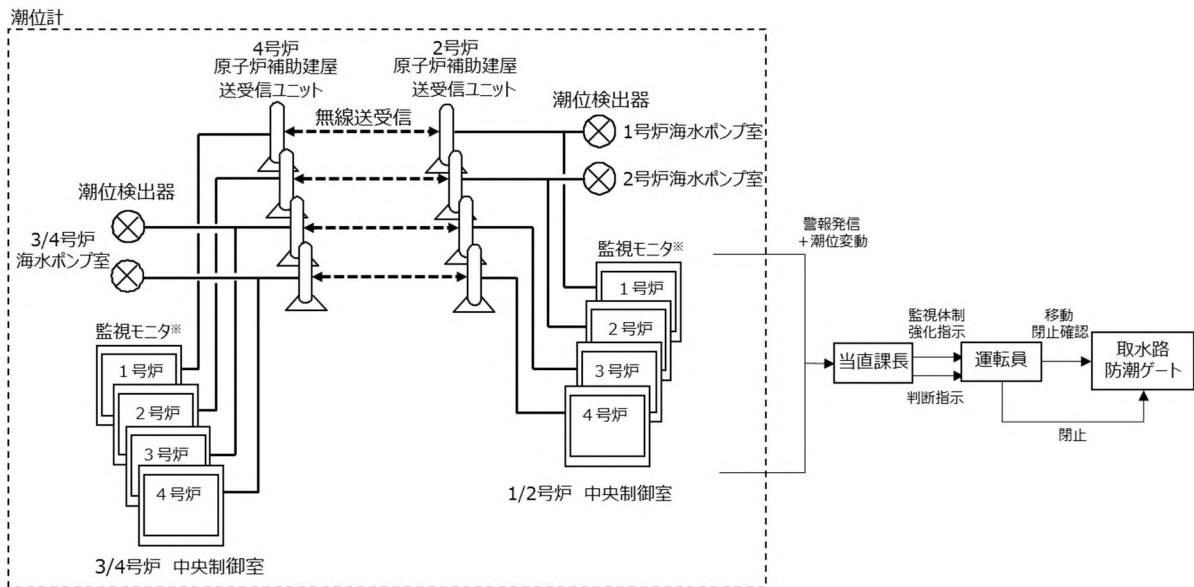
図3 取水路防潮ゲートの閉止判断基準（トリガー）を検知するための一連の設備
