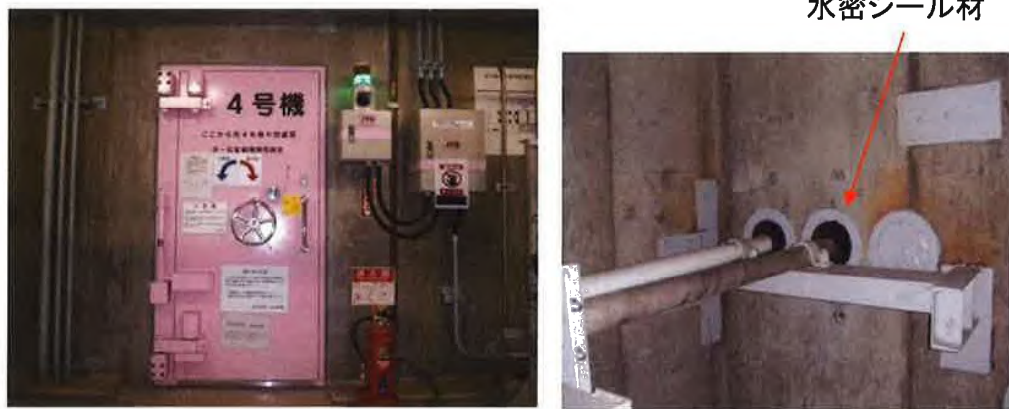
図-2-4-38 水密扉、貫通部対策の代表例
