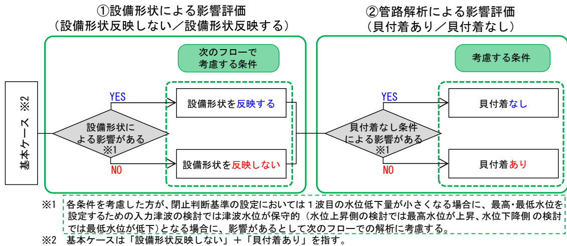
図-1-4-2 取水口側の影響評価検討フロー
