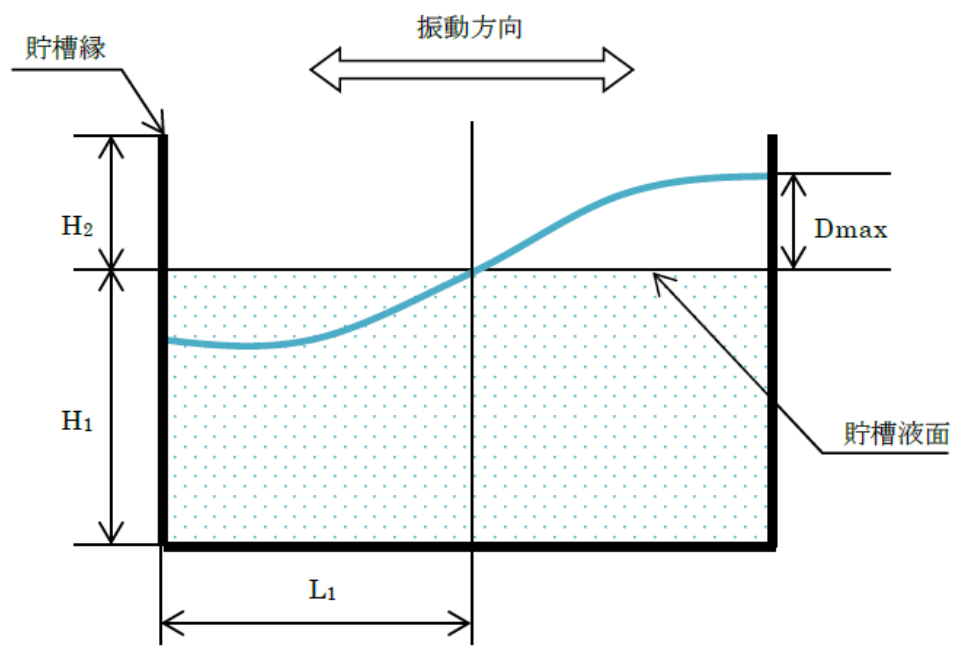
[立面図]
