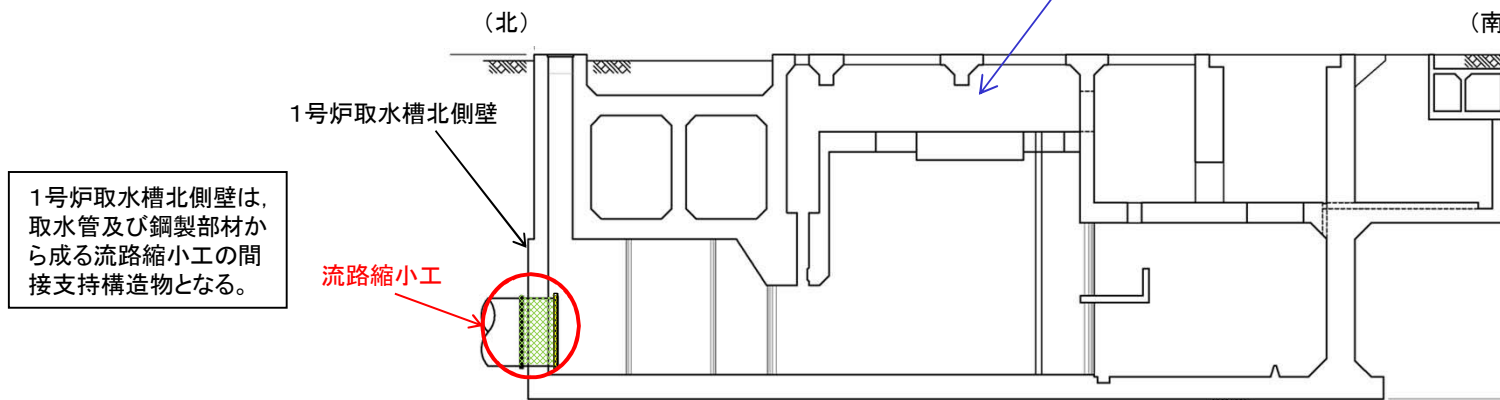
(1号取水槽断面図)
