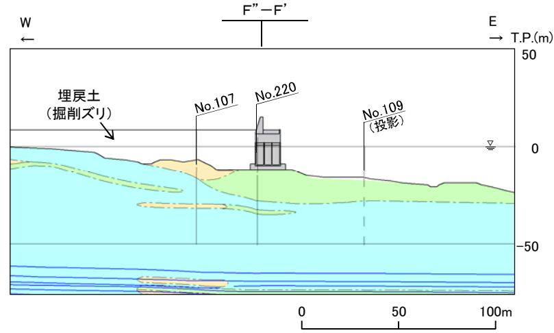
防波壁(波返重力擁壁) F-3 断面横断面図(岩級・シーム)
