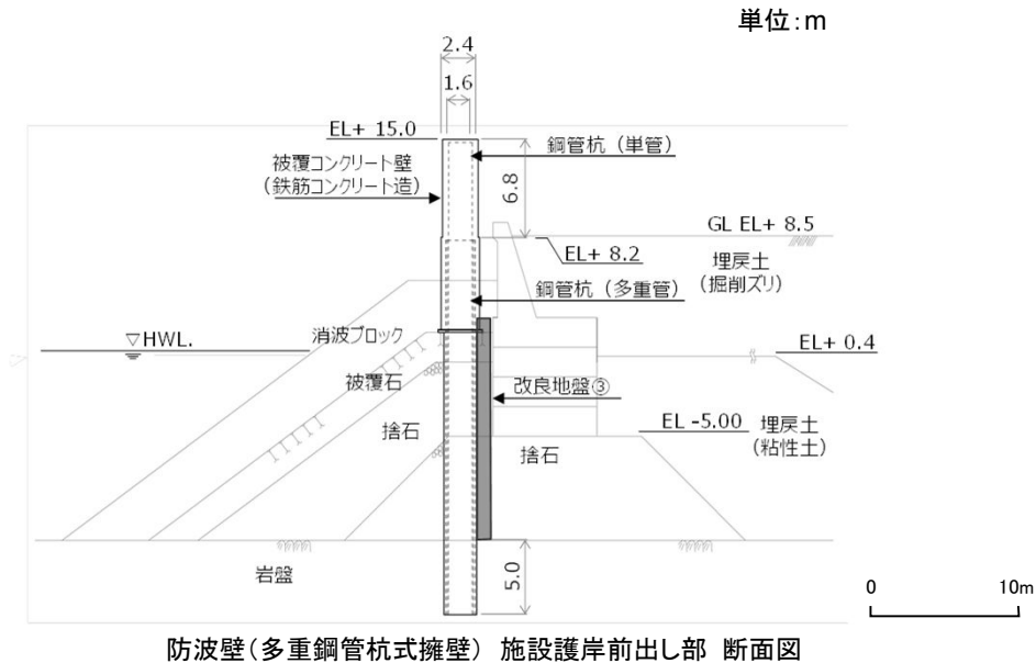
防波壁(多重鋼管杭式擁壁) 施設護岸前出し部 断面図
