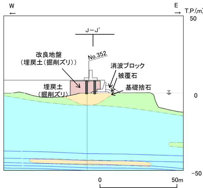
防波壁(鋼管杭式逆T擁壁) J-1断面横断面図(岩級・シーム)
