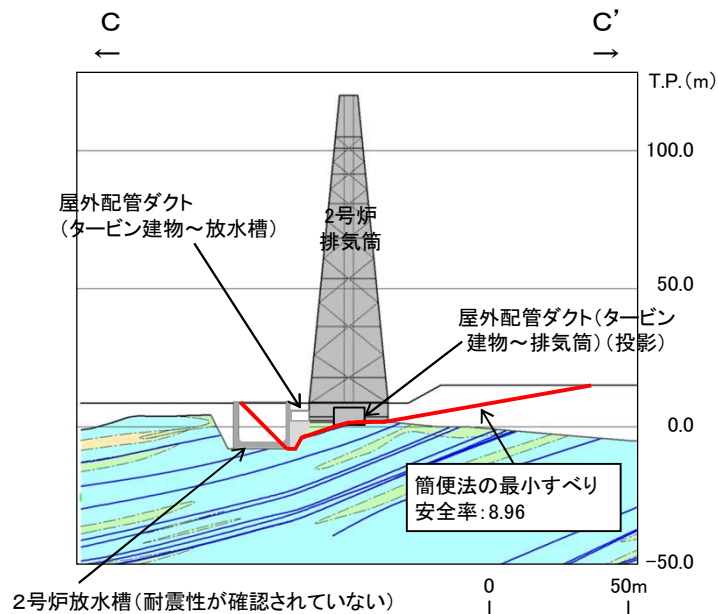
2号炉排気筒等 地質断面図(岩級・シーム)
