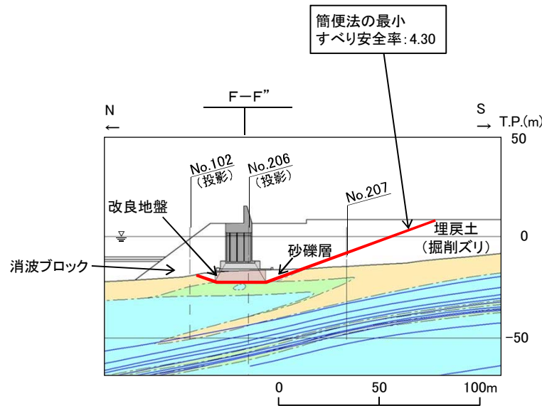
防波壁(波返重力擁壁) F-1断面 横断面図(岩級・シーム)
