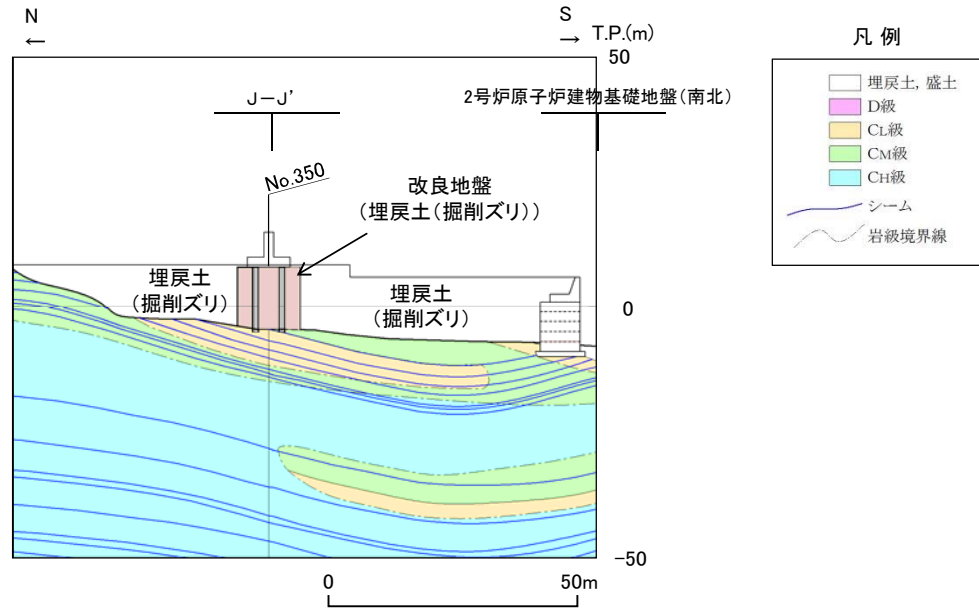
防波壁(鋼管杭式逆T擁壁) J-3断面 横断面図(岩級・シーム)
