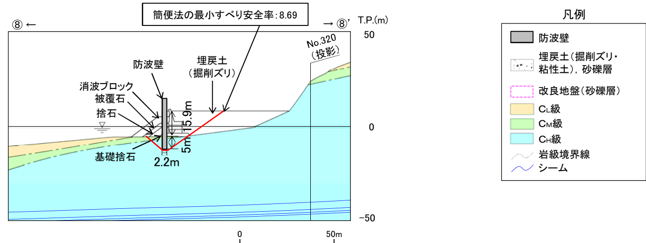
防波壁(多重鋼管杭式擁壁) ⑧-⑧'断面横断面図(岩級・シーム)
