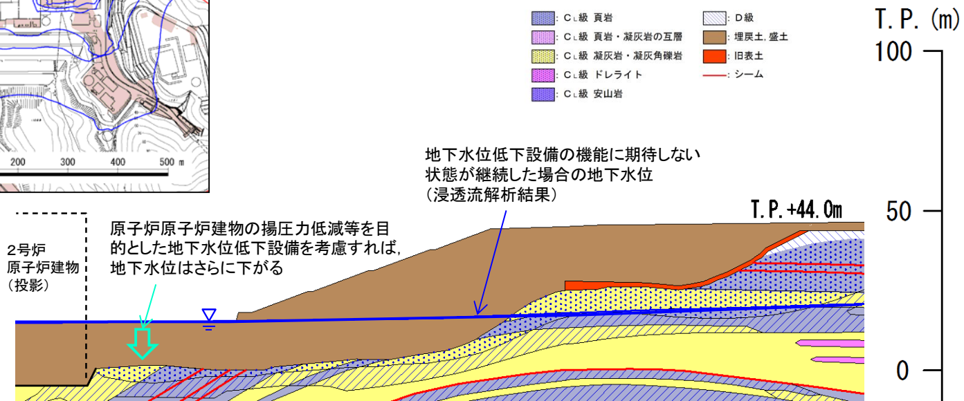
地下水位低下設備の機能に期待しない状態が継続した場合の浸透流解析結果(断面図)
