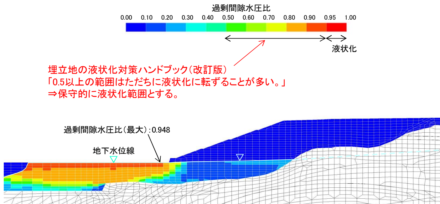
2号炉南側盛土斜面(⑥-⑥'断面)の過剰間隙水圧比分布図(時刻歴最大)
