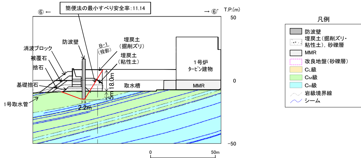
防波壁(多重鋼管杭式擁壁) ⑥-⑥'断面横断面図(岩級・シーム)
