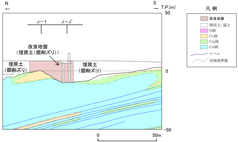
防波壁(鋼管杭式逆T擁壁) J-2断面横断面図(岩級・シーム)
