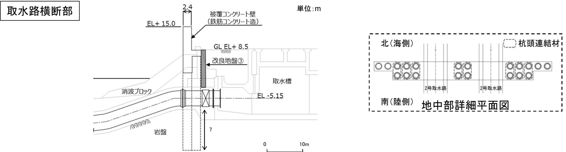
防波壁(多重鋼管杭式擁壁) 取水路横断部 断面図
