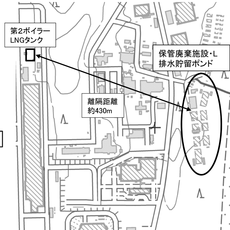
第2ボイラーLNGタンクと排水貯留ポンド及び保管廃棄施設・Lの離隔距離
