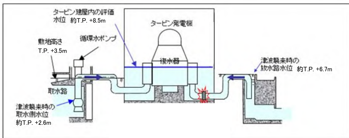
図-2-4-12 タービン建屋内の評価水位と取水側水位及び放水ピット側水位の概略図
