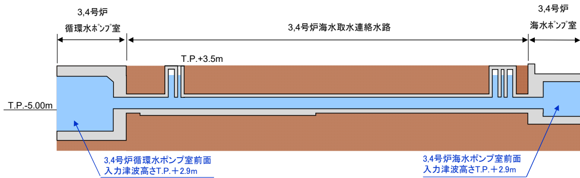
図-2-2-25 3,4号炉海水取水連絡水路断面図
