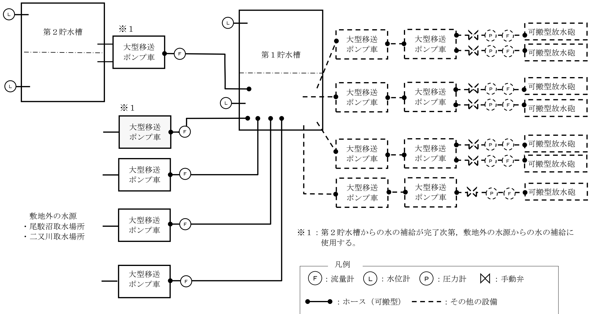
第 31. 1 図 重大事故等への対処に必要となる水の供給設備の系統概要図 (その 1) (大気中への放射性物質の拡散抑制への対処及び第 1 貯水槽へ水を補給の対処)
