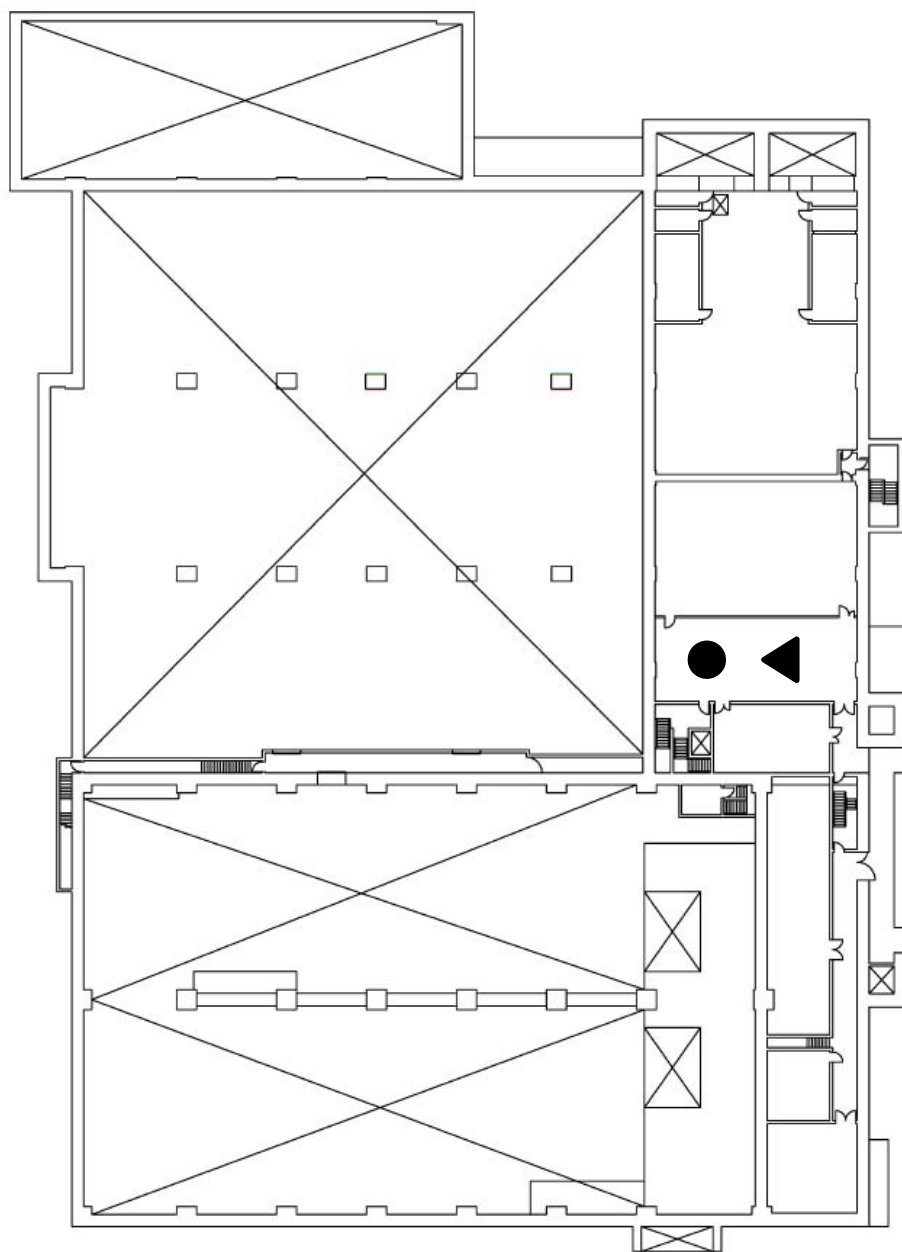
第1.11-15図 使用済燃料受入れ・貯蔵建屋環境測定設備，制御建屋放射線計測設備配置図
