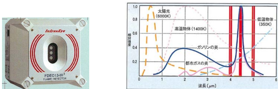
第2図 防爆型炎感知器の概要
