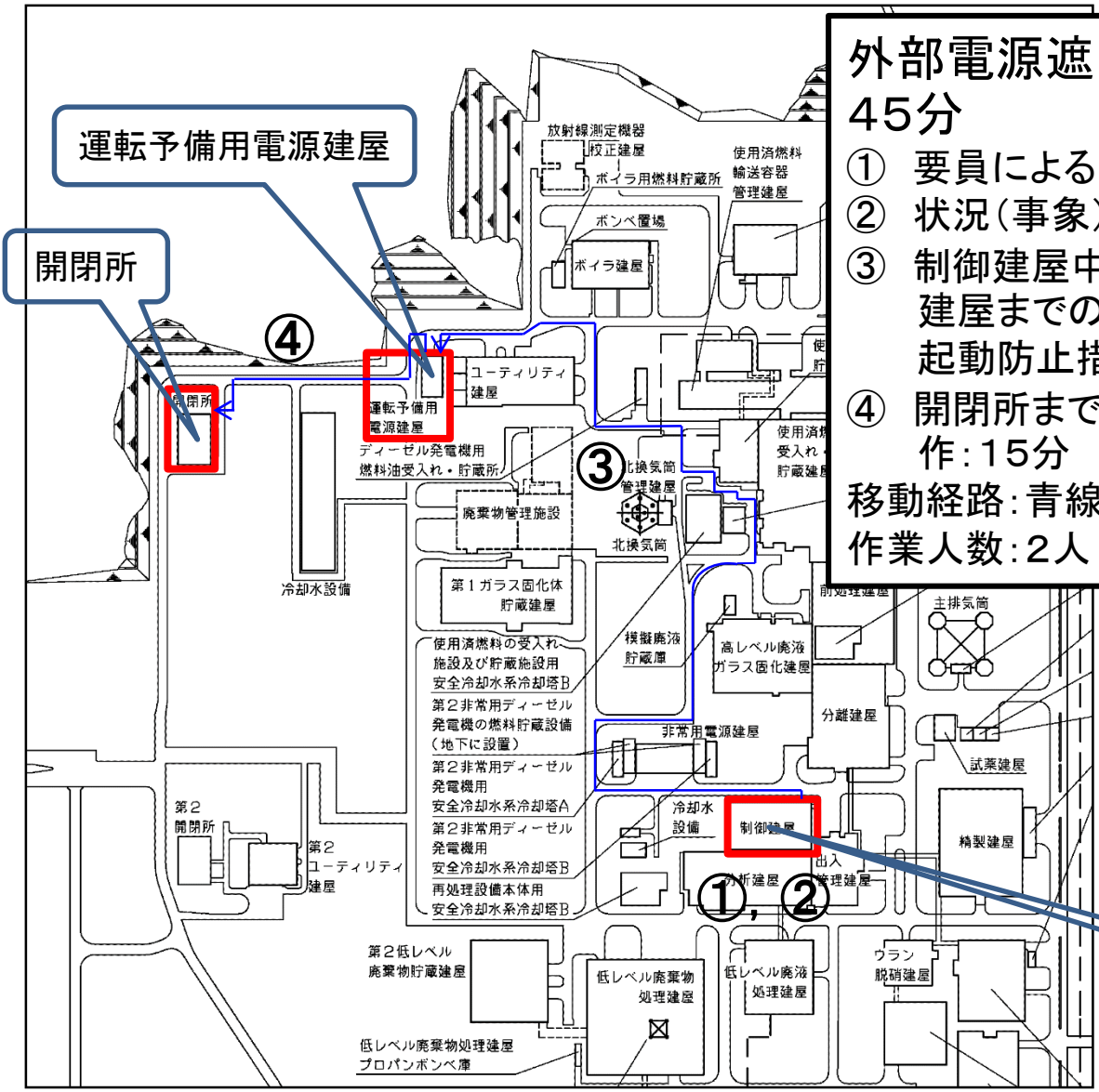
図4: 外部電源の遮断場所の配置と操作時間
