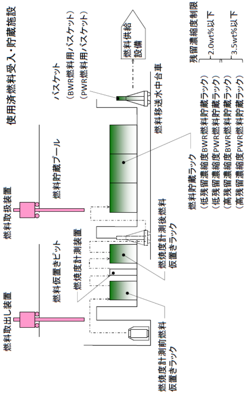
図1：使用済燃料貯蔵施設における臨界管理
