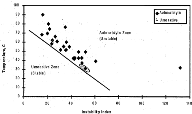
図1：HANの不安定性指標 1)
