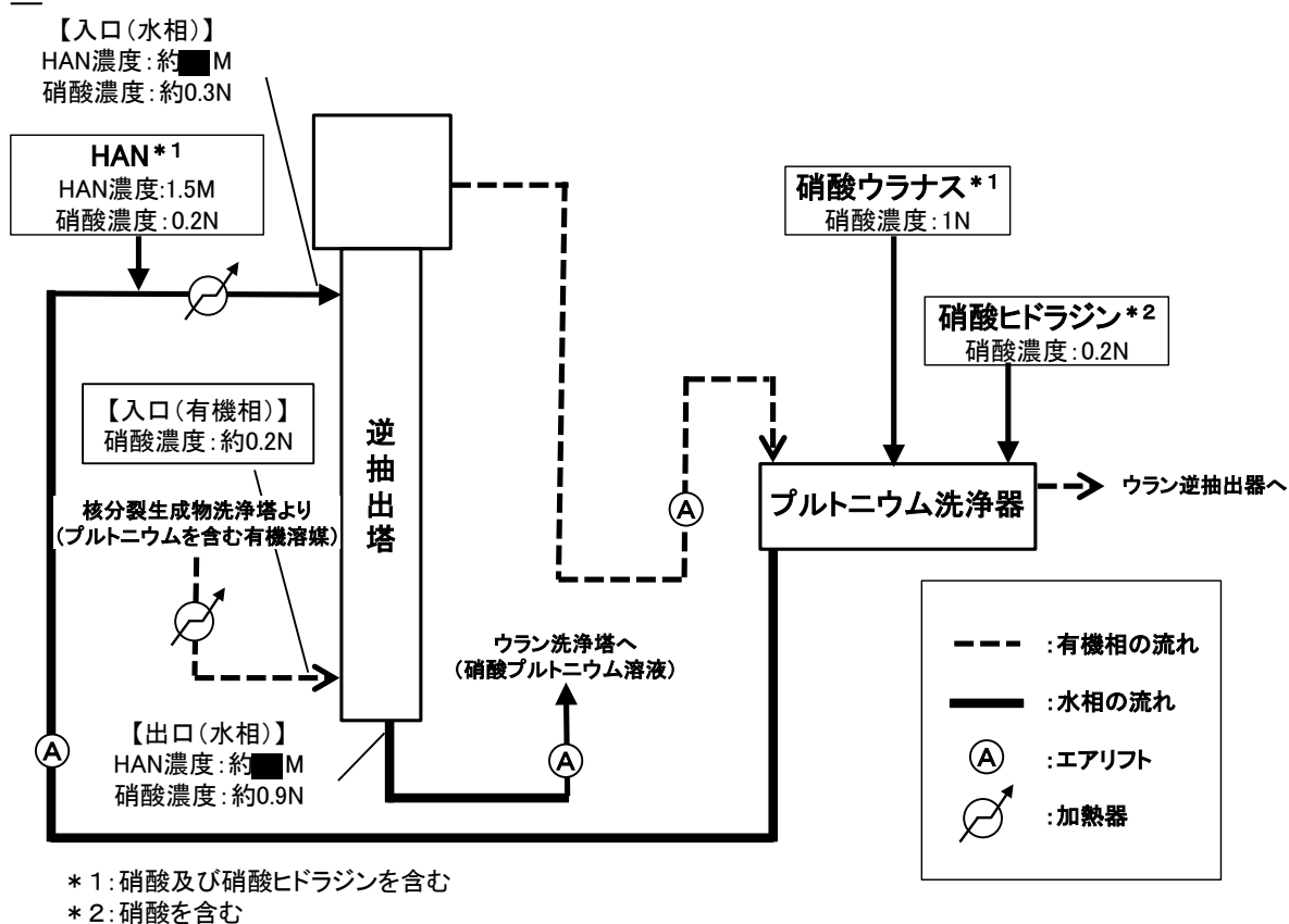
図 2 : 逆抽出塔周辺の系統概要
