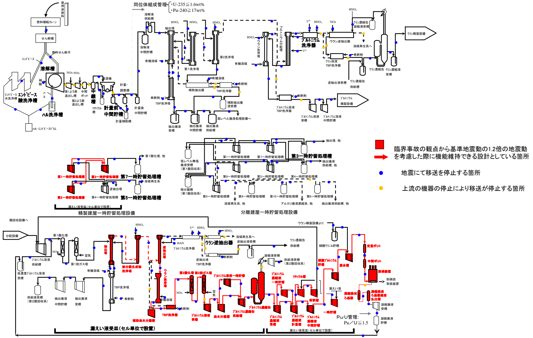
図1: 臨界事故の観点から基準地震動の1.2倍の地震動を考慮した際に機能維持できる設計としている対象箇所と地震により移送が停止する箇所(セル内)
