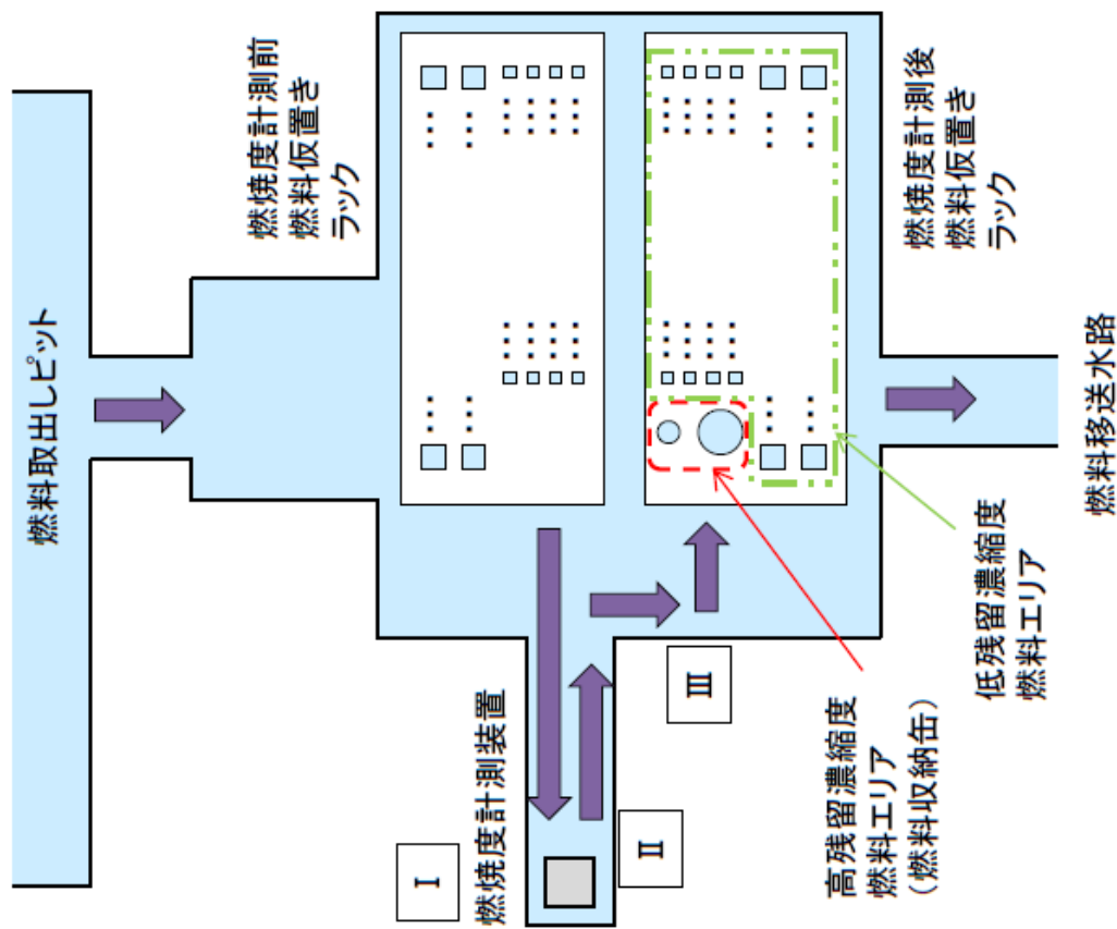
図2：使用済燃料貯蔵集合体の燃焼度計測の流れ
