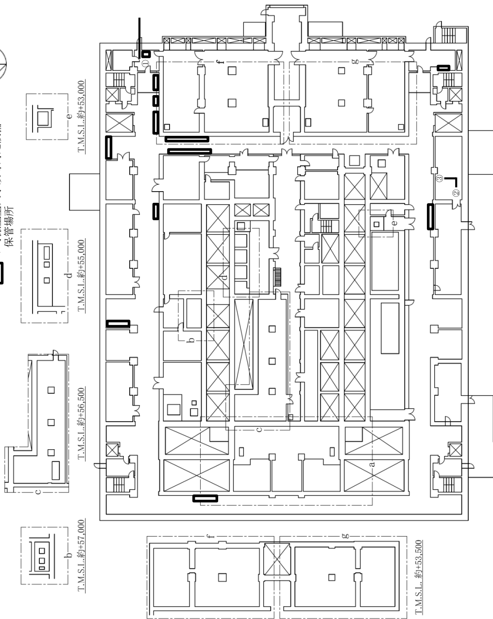
第29図 「地震発生による全交流動力電源の喪失を伴う精製建屋の水素掃気機能喪失事故」の 発生防止対策（個別供給）の建屋内ホース敷設ルート（第1接続口） （南1ルート）（地上1階）
