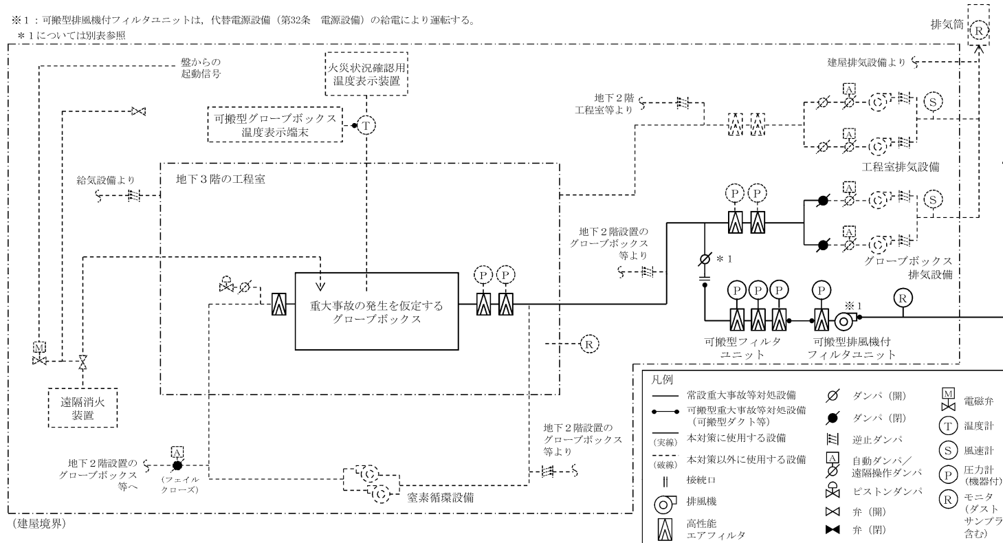
第 2-3.5 図 代替グローブボックス排気系の系統概要図
