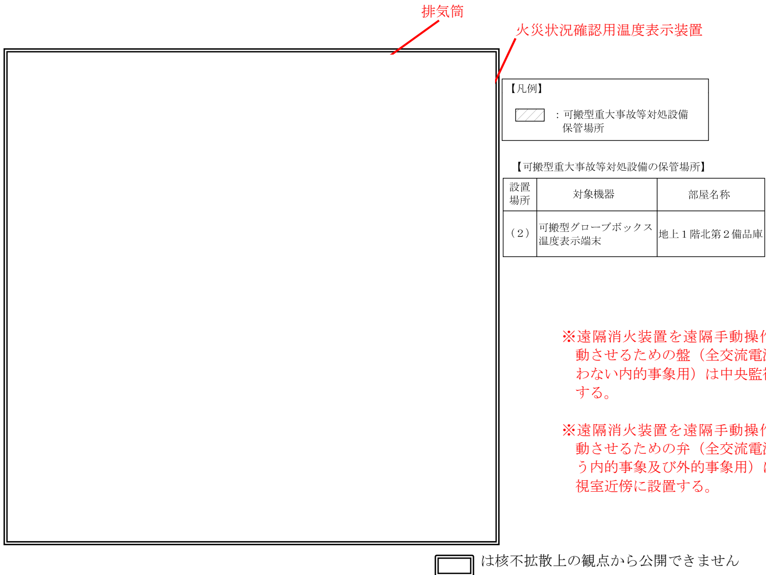
第 2-2.3 図 閉じ込める機能の喪失に対処するための設備の機器配置概要図（燃料加工建屋地上 1 階）
