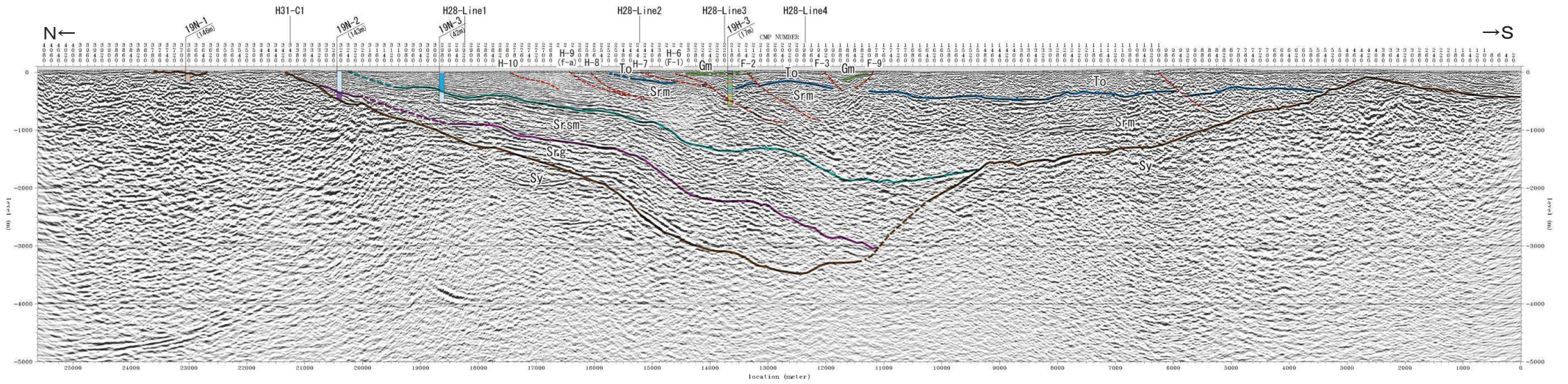
深度断面図(解釈あり)
