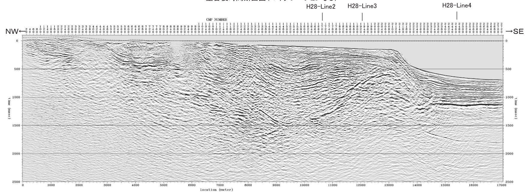
マイグレーション後時間断面
