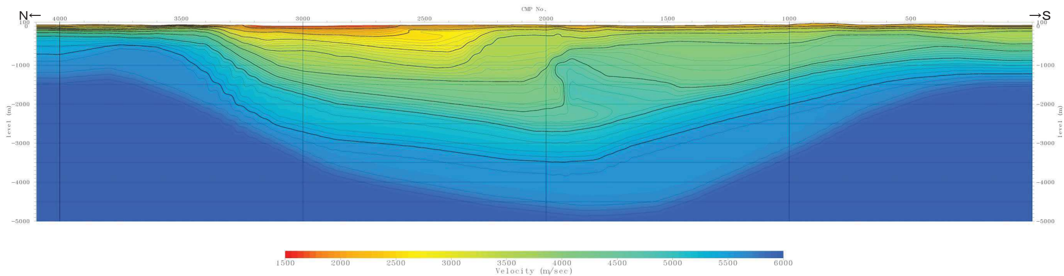
区間速度分布図
