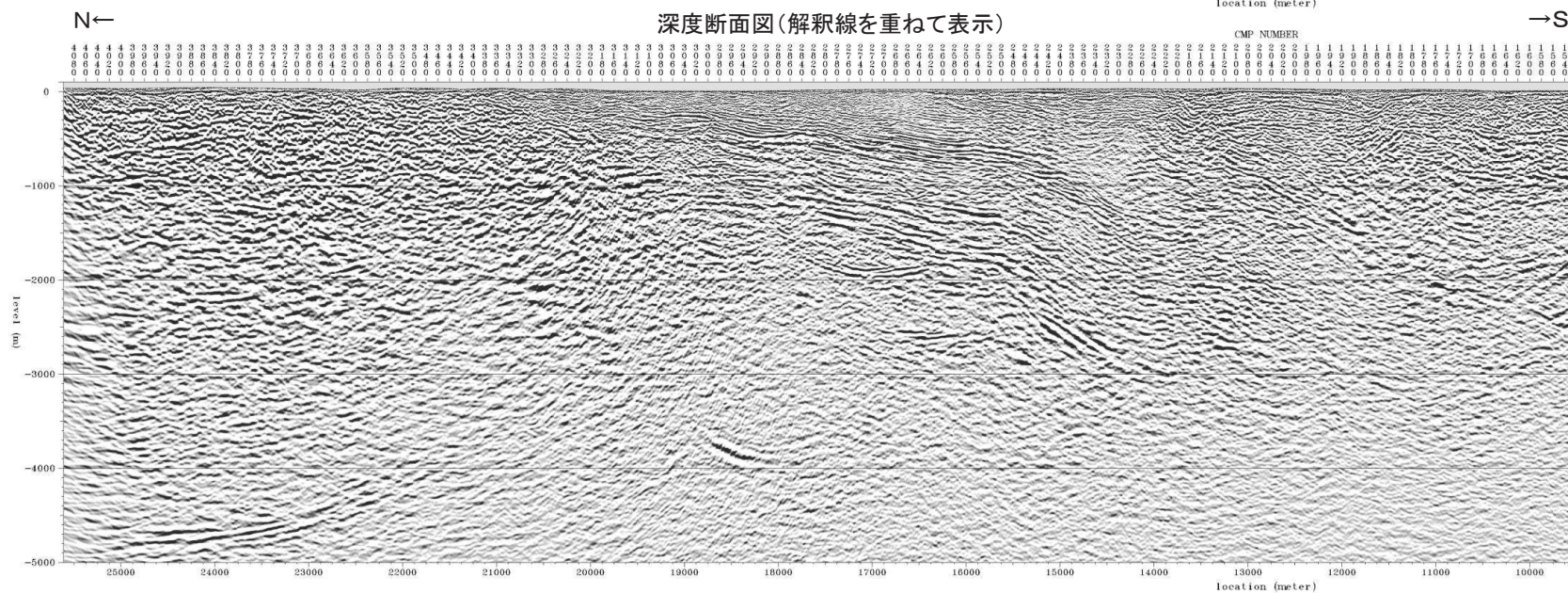
深度断面図
