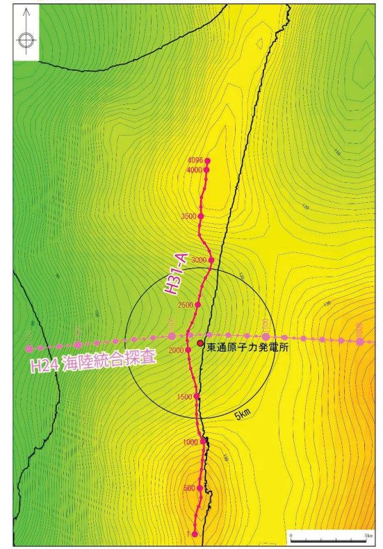
ブーゲー異常
