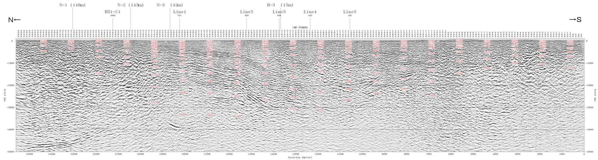
深度断面図(区間速度)
