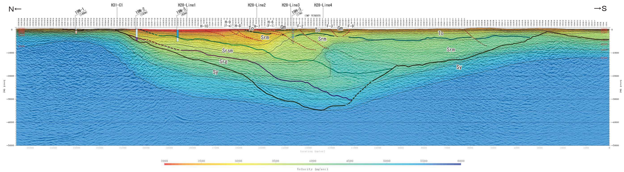
深度断面図(速度構造・解釈あり)
