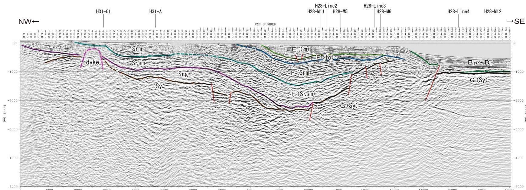
深度断面図(解釈線を重ねて表示)
