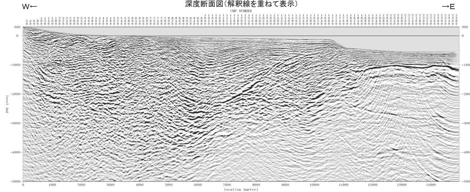
深度断面図
