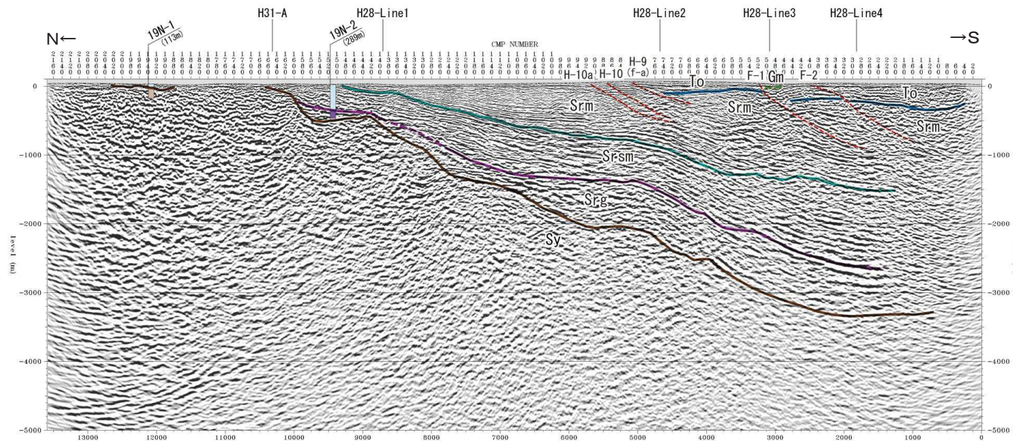
深度断面図(解釈線を重ねて表示)
