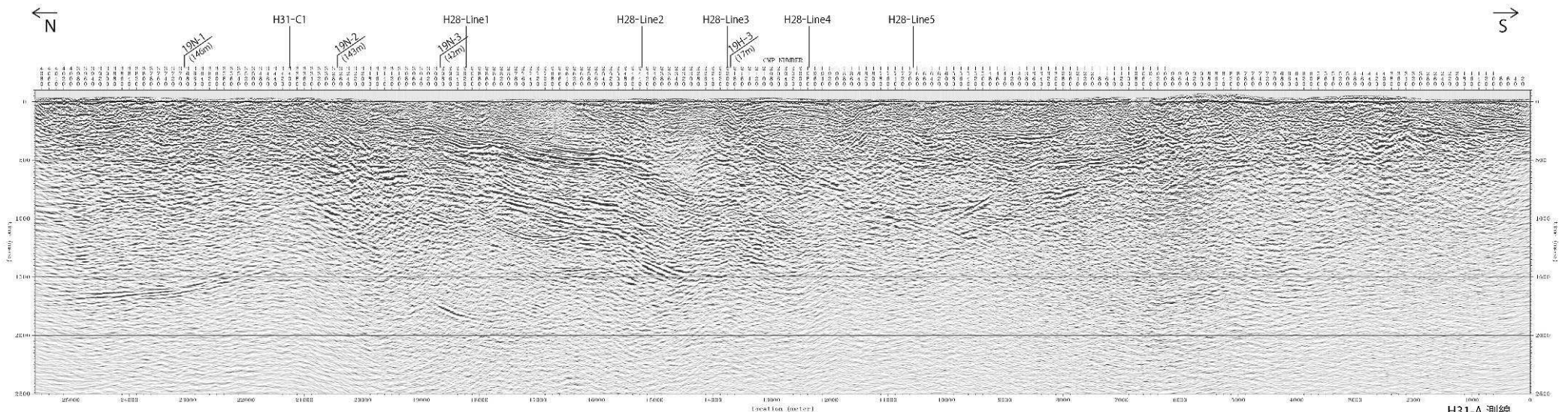
マイグレーション後時間断面図
