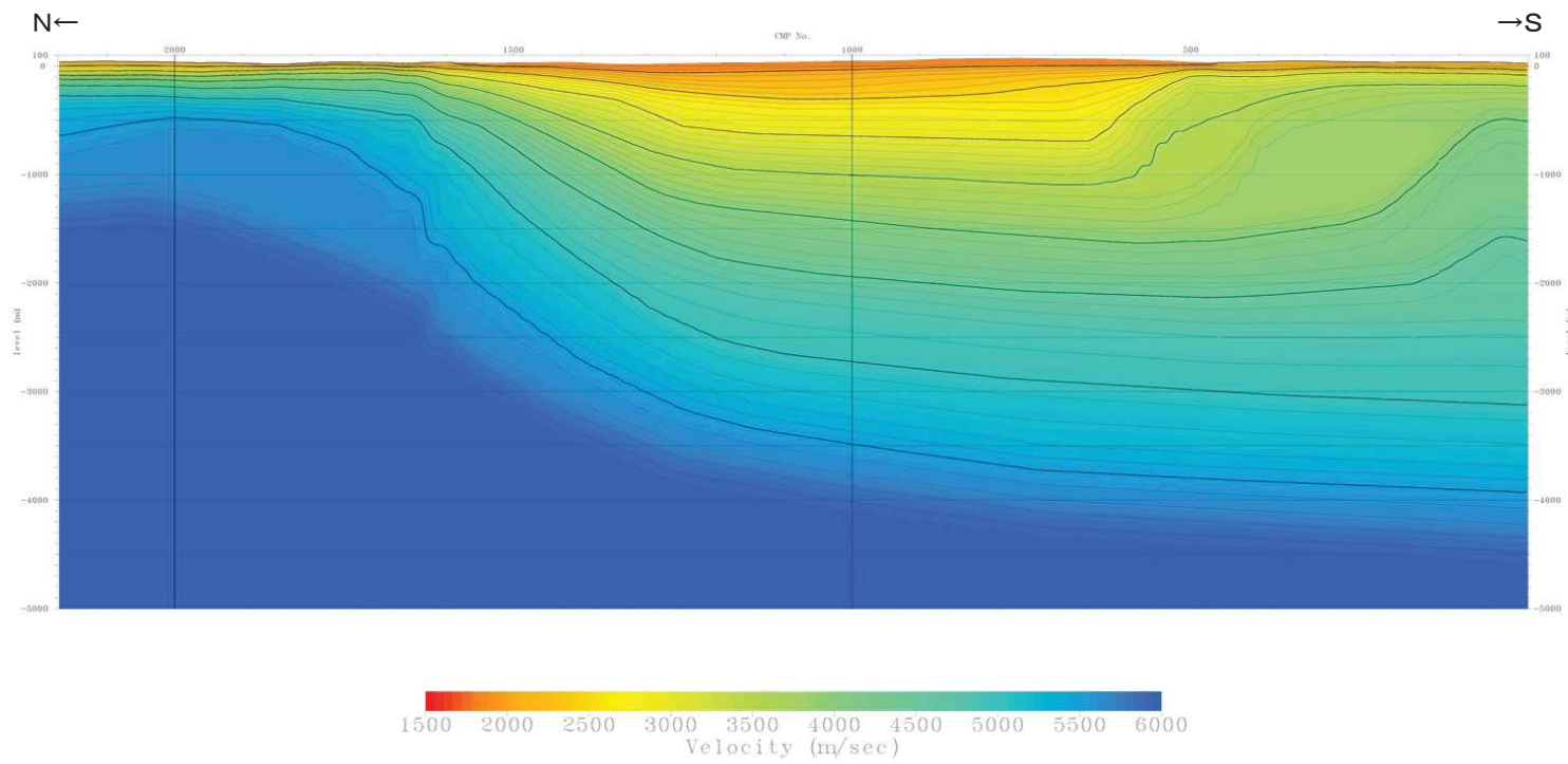
区間速度分布図
