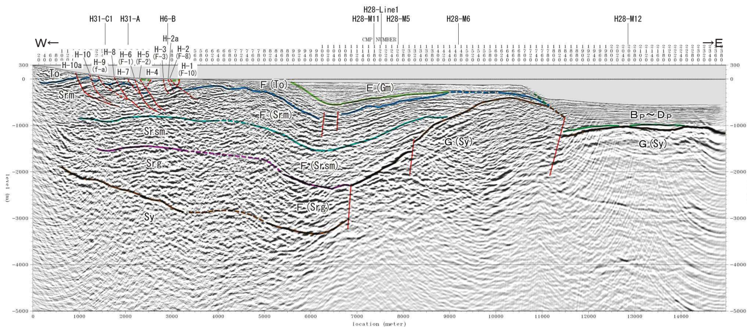
深度断面図(解釈線を重ねて表示)
