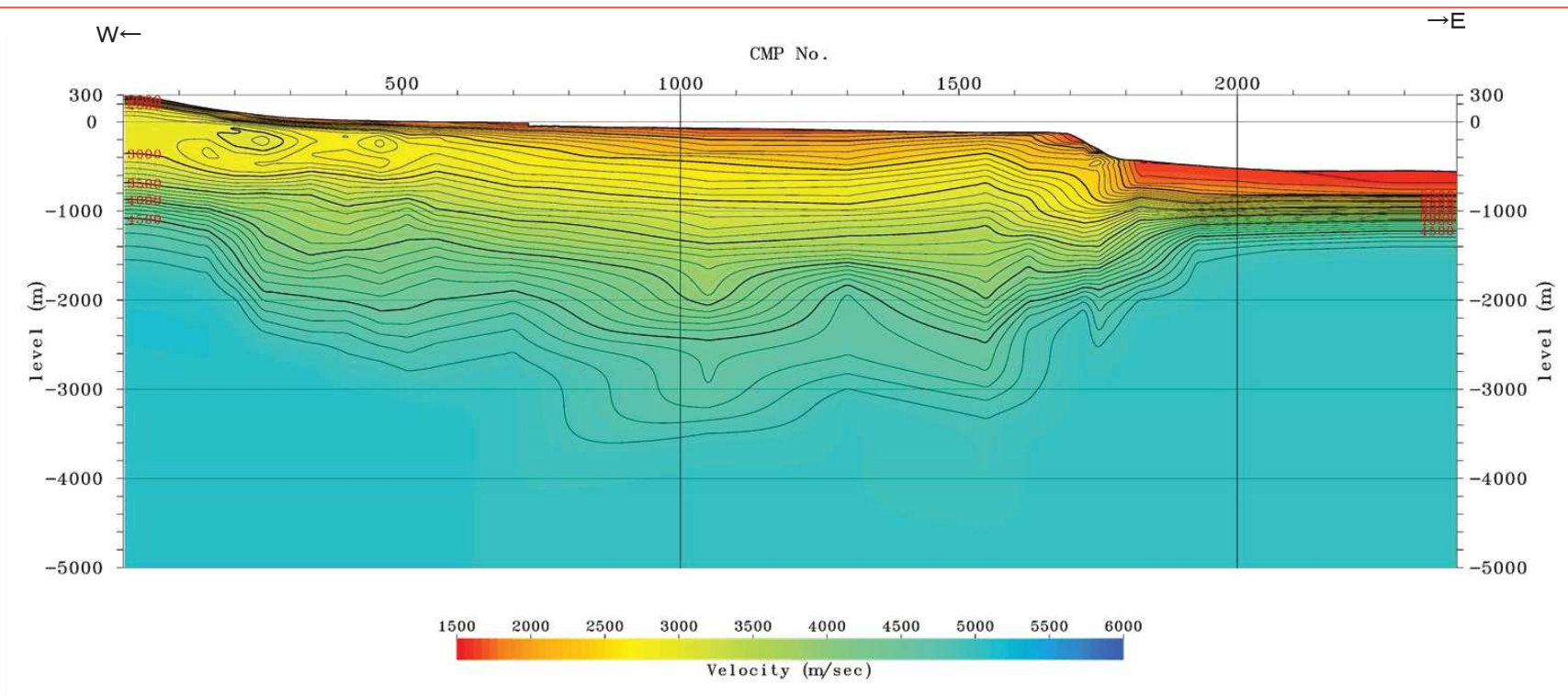
区間速度分布図
