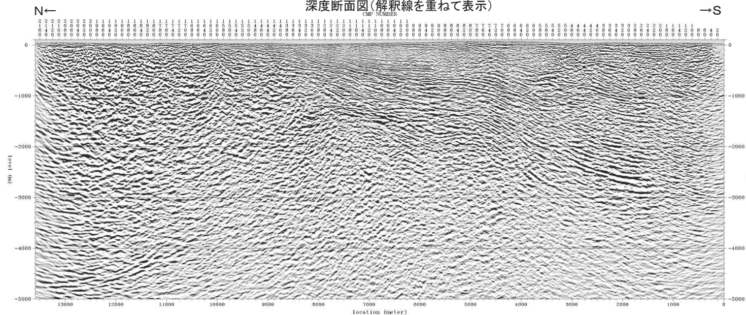
深度断面図
