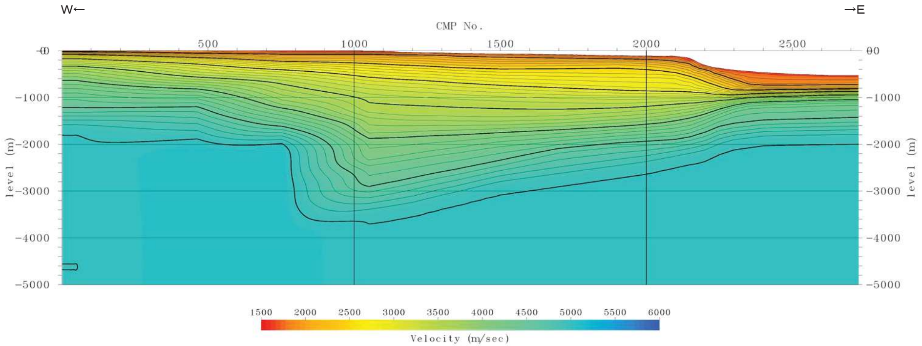
区間速度分布図
