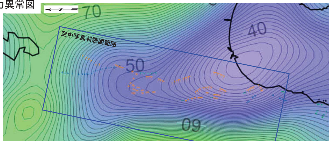
重力異常図
