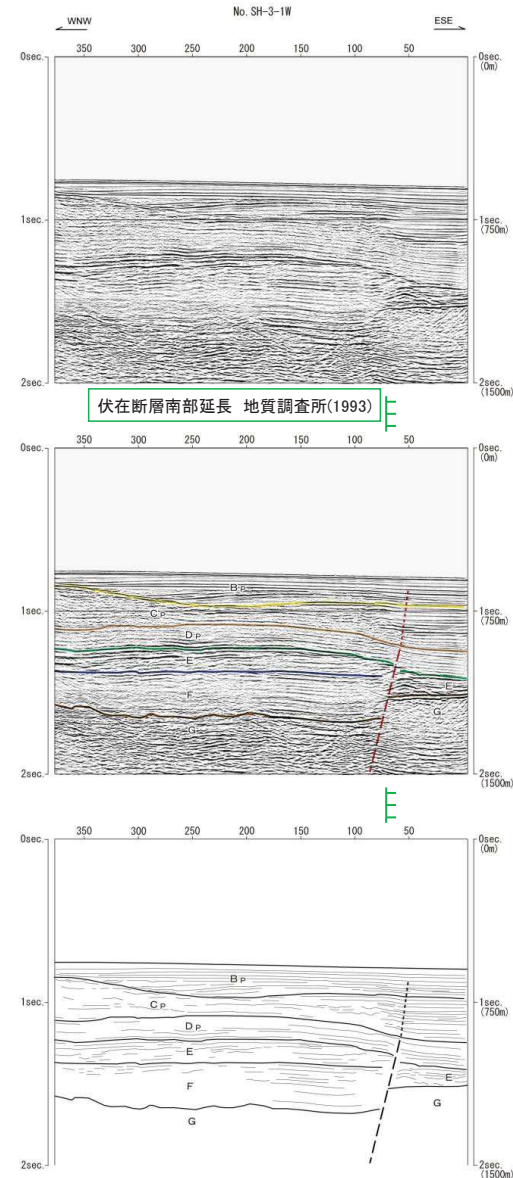
音波探査記録及び海底地質断面図(No.SH-3-1W測線)
