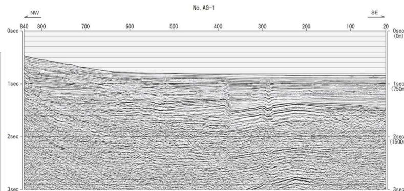
伏在断層位置 地質調査所(1993)
