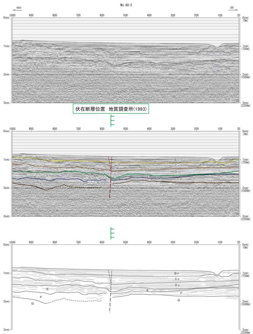
音波探査記録及び海底地質断面図(No.AG-2測線)
