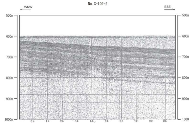
伏在断層位置 地質調査所(1993)
