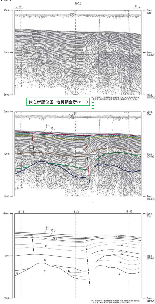
音波探査記録及び海底地質断面図(G-35測線)
