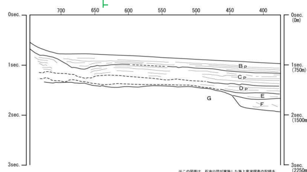
音波探査記録及び海底地質断面図(JS73-1測線)
