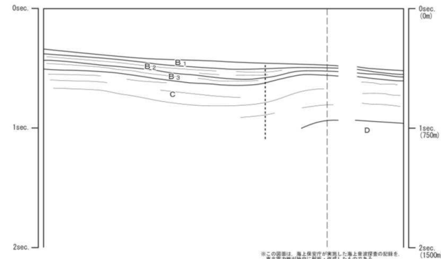
音波探査記録及び海底地質断面図(H-16-2測線)
