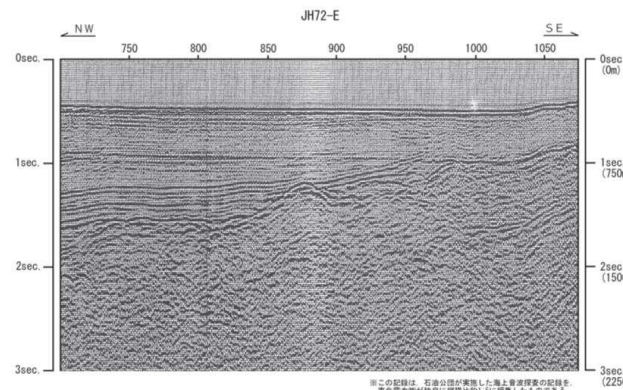
伏在断層南部延長 地質調査所(1993)
