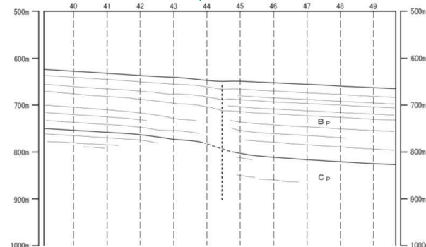
音波探査記録及び海底地質断面図(No.C-102-2測線)
