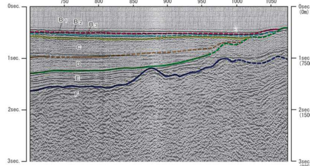
伏在断層南部延長 地質調査所(1993)
