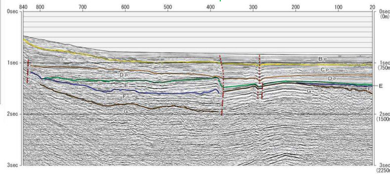
伏在断層位置 地質調査所(1993)
