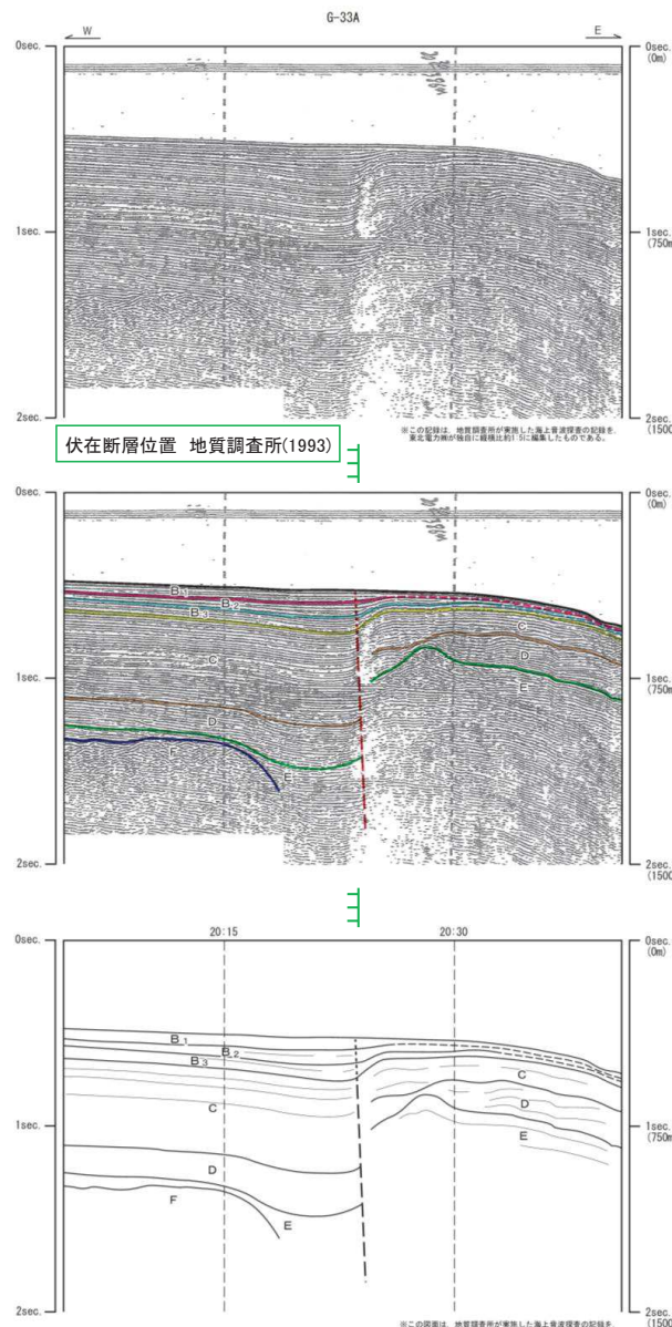
音波探査記録及び海底地質断面図(G-33A測線)
