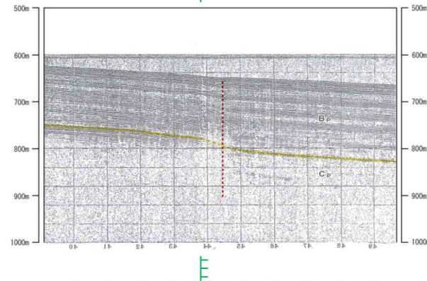
伏在断層位置 地質調査所(1993)
