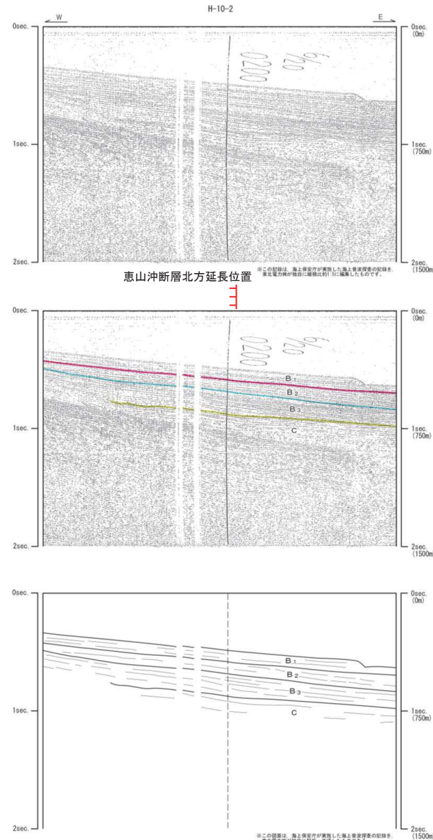
音波探査記録及び海底地質断面図(H-10-2測線)
