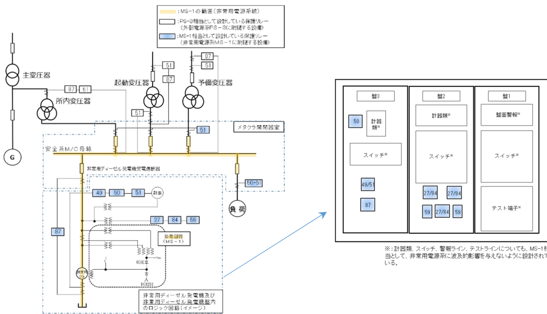
図2 非常用電源系及び外部電源系に附属する保護リレーに対する設計整理図
