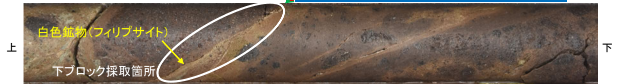
ボーリングコア写真(H' - -1.3孔) — 粘土状破砕部 — 固結した破砕部
