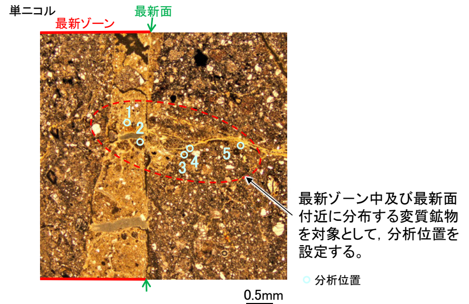
EPMA分析(定量)の分析位置の例 (S-1, K-10.3SW孔)
